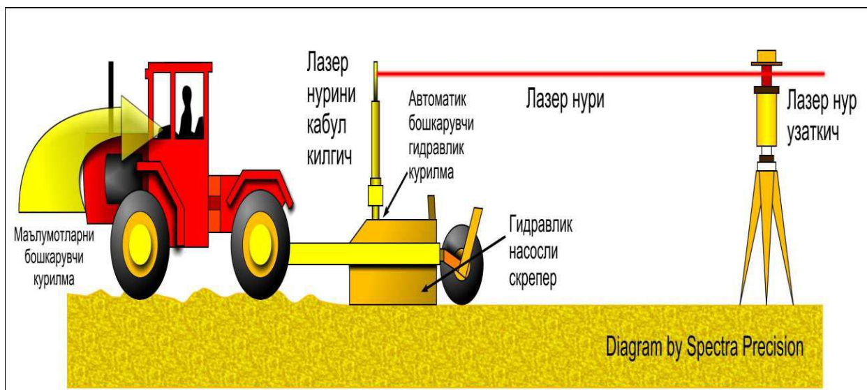
Расм. Лазер нивелири қурилмаларининг ишлаш принциплари
