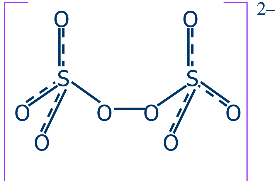
Пероксодисульфат-ион \text{S}_2\text{O}_6(\text{O}_2)^{2-}
