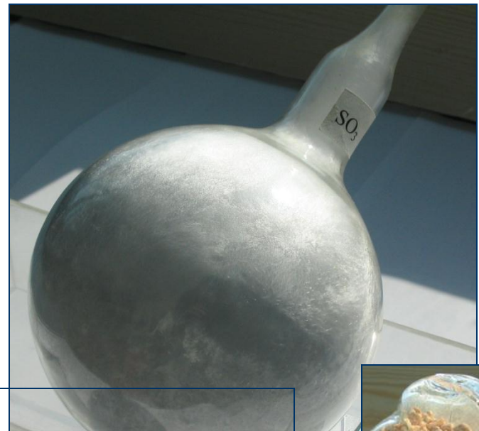
Препарат (\text{SO}_3)_x
