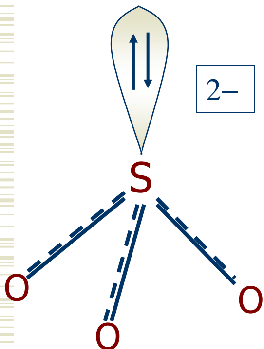
Сульфит-ион
