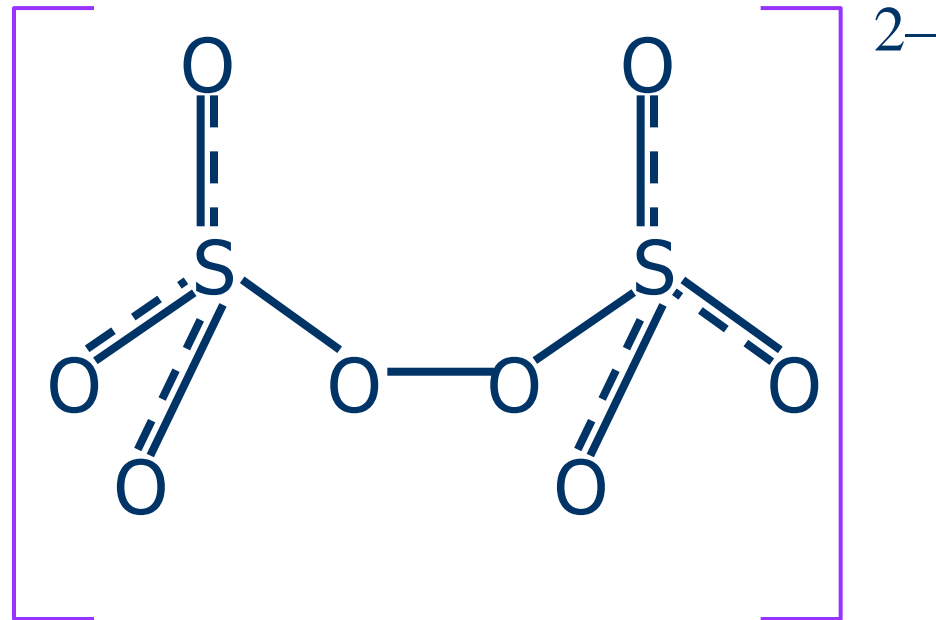
Пероксодисульфат-ион \text{S}_2\text{O}_6(\text{O}_2)^{2-}
