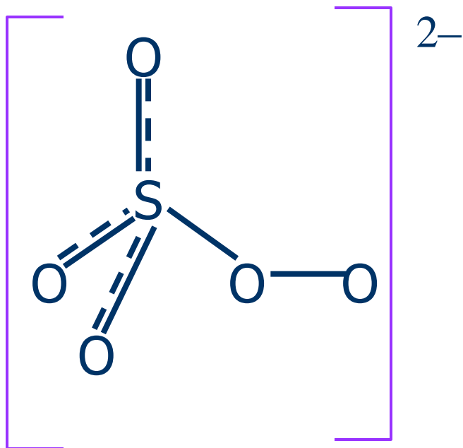
Пероксосульфат-ион \text{SO}_3(\text{O}_2)^{2-}
