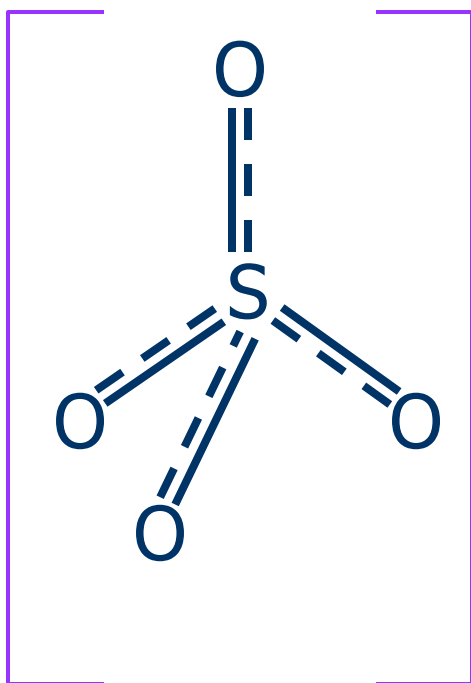
Сульфат-ион
