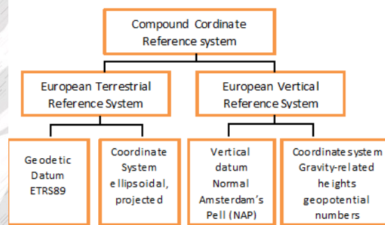
2-Расм CCRS-блок схемаси
