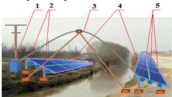
5-rasm. Bevosita dala yoqasidan oqib oʻtatigan suv xavzasi boʻyiga kichik quvvatli quyosh elektr stansiyalarini qurish (meliorativ tadbirlarga xalaqit bermaydigan uslubda).
