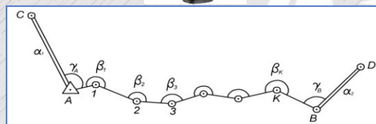
1-rasm: Trimble S5 taxeometr va poligonometriya yo'li sxemasi
