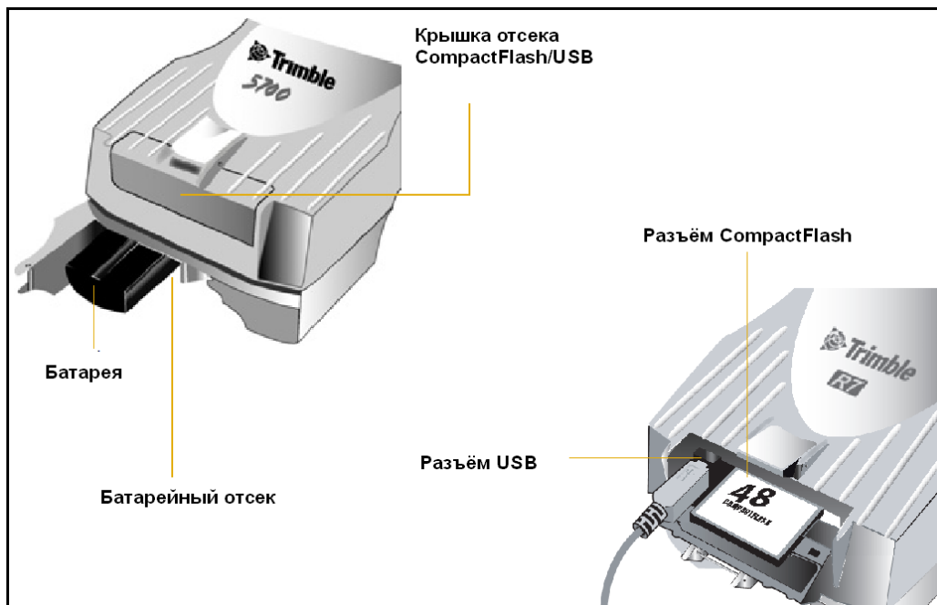
Рисунок 3.5 Нижняя панель
