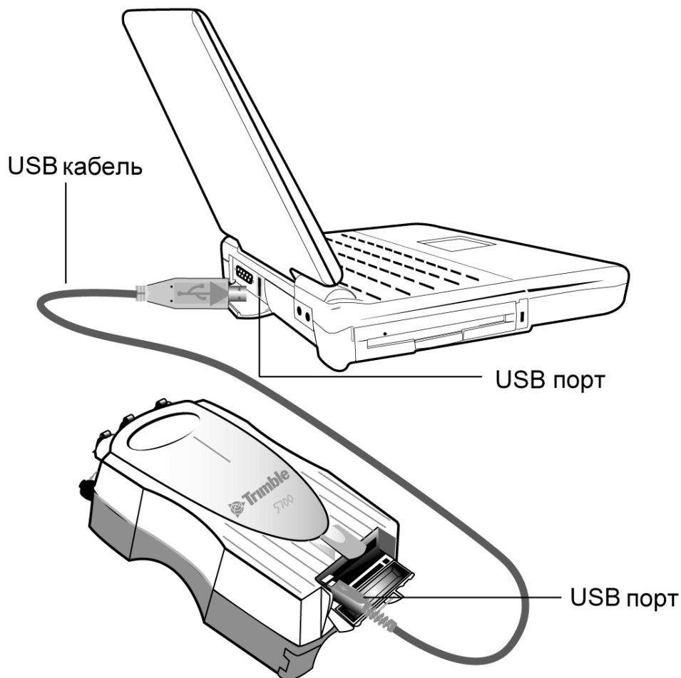
Рис. 5.2. Подсоединение приемника 5700 к компьютеру по USB
