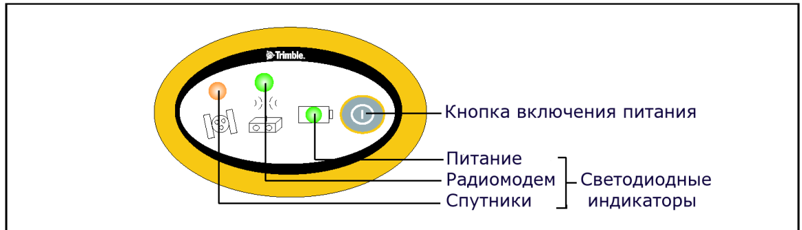
Рис. 13.1. Кнопки и светодиодные индикаторы на передней панели приемника 5800.
