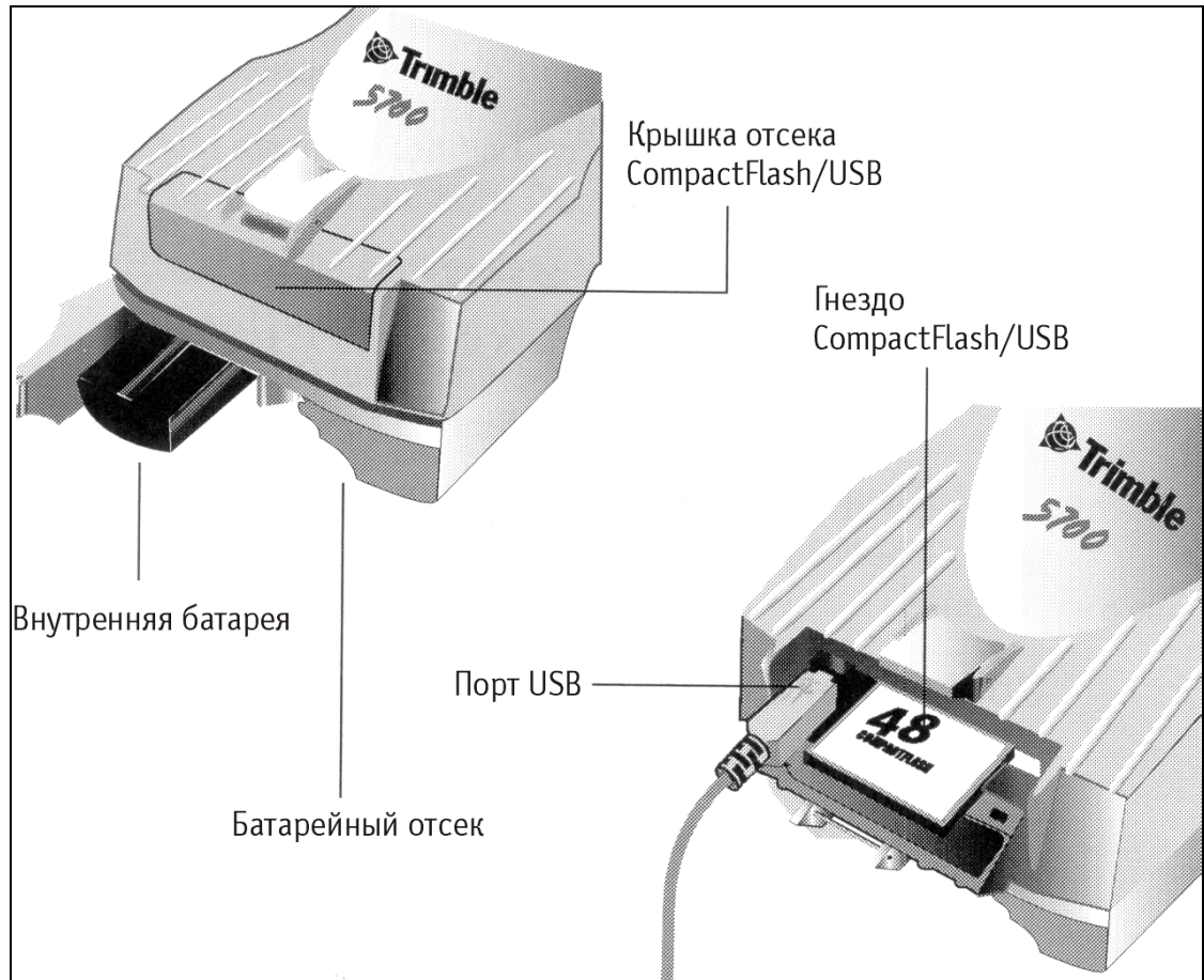
Рис. 2.5 Верхняя панель
