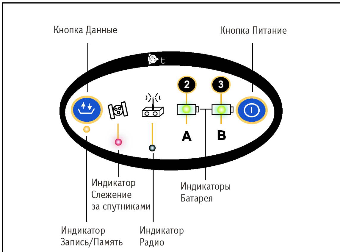
Рис. 3.1 Органы управления, расположенные на передней панели
