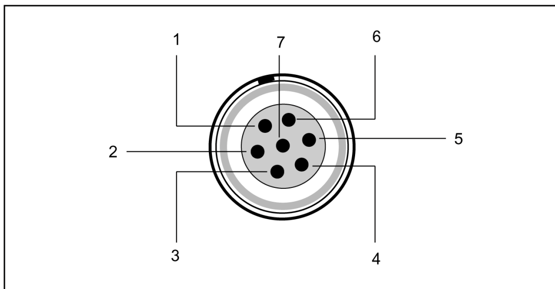
Рис. 9.2. Нумерация контактов разъема Порт 1.
