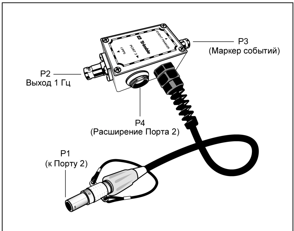
Рис. 9.3. Кабель Маркер События / PPS
