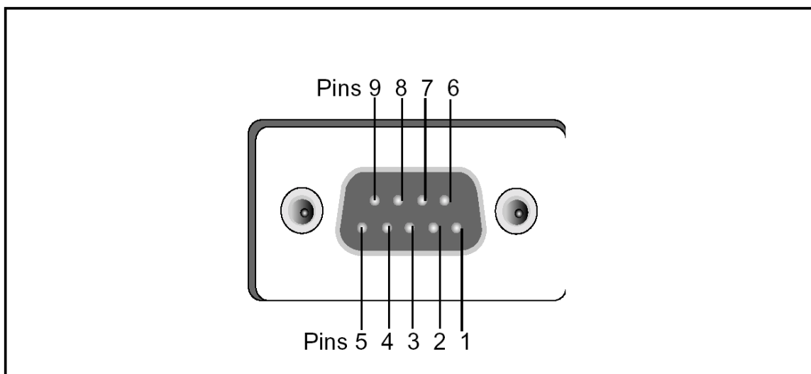
Рис. 18.3. Нумерация контактов разъема Порт 2.
