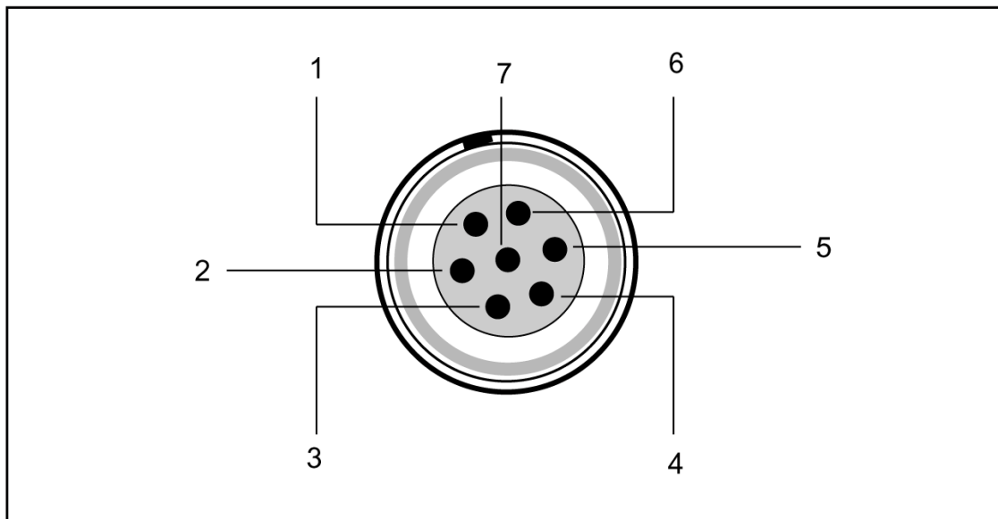
Рис. 18.2. Нумерация контактов разъема Порт 1.
