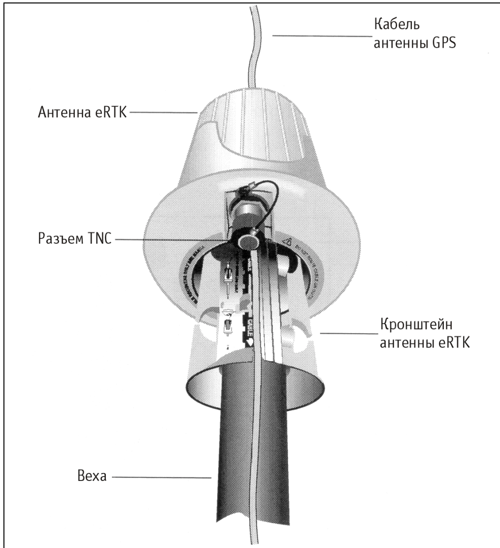
Рис. 2.7 Антенна eRTK на кронштейне
