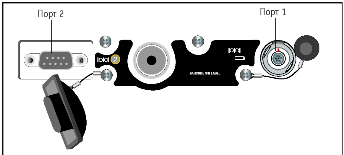
Рис. 18.1. Последовательные порты приемника 5800.
