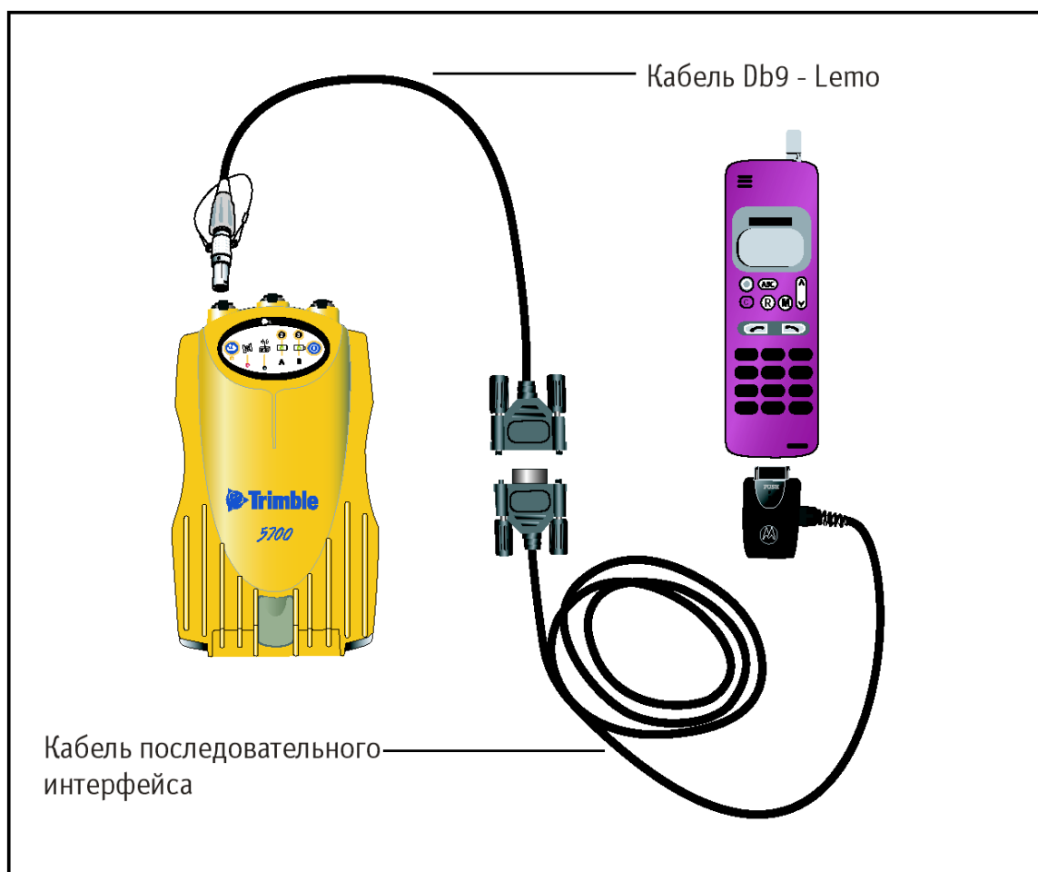
Рис. 2.13 Подключение сотового модема
