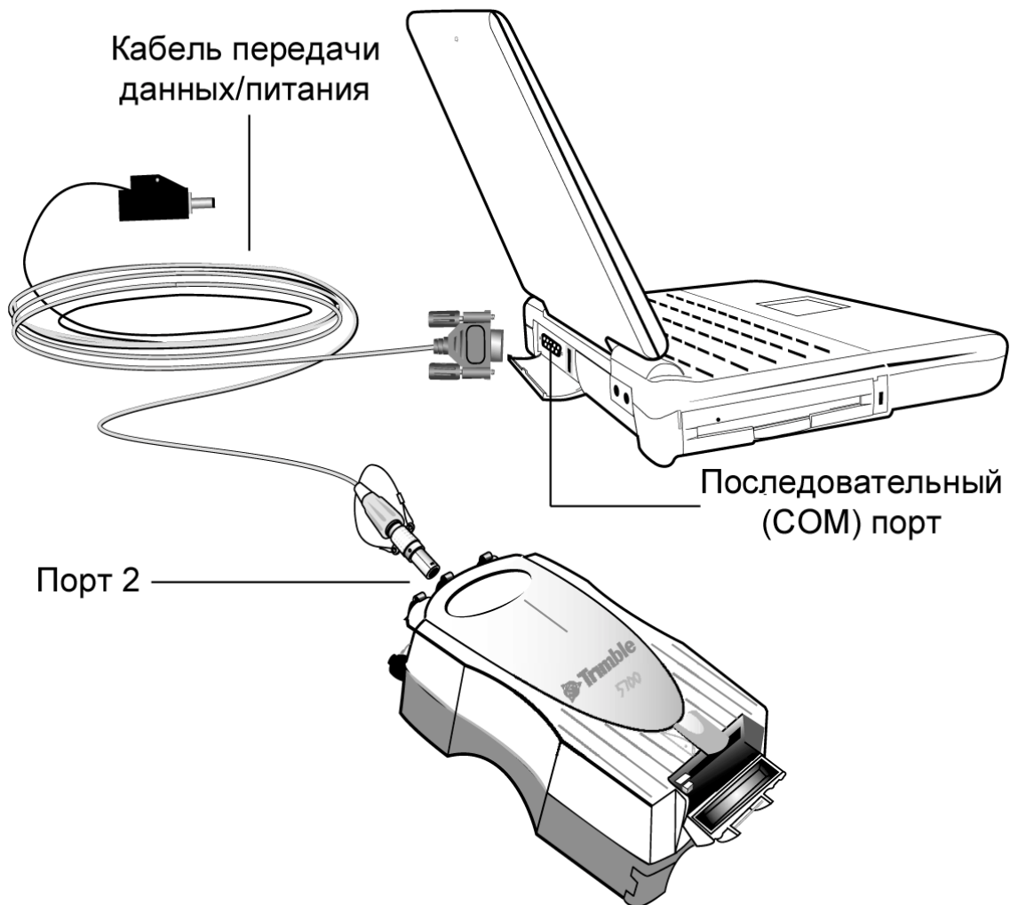
Рис. 5.1. Подсоединение приемника 5700 к компьютеру по последовательному порту
