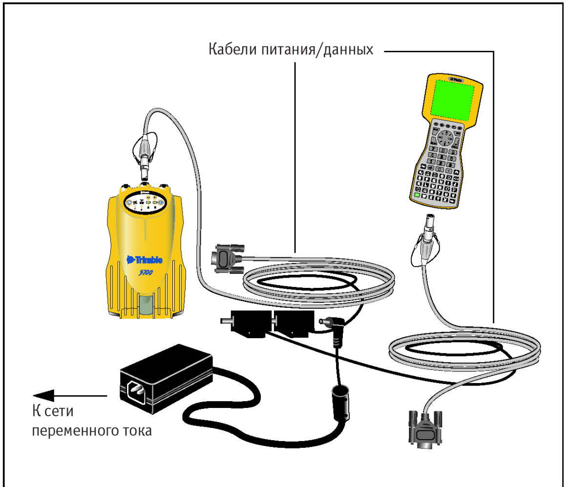
Рис. 3.3 Зарядка внутренних батарей контроллера TCS1/TSCe и приемника
