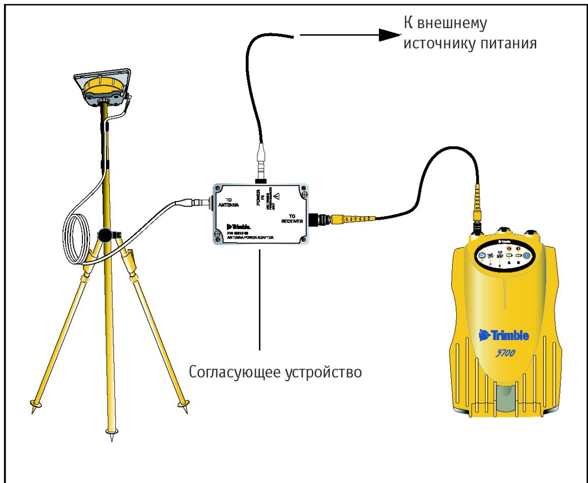
Рис. 2.15 Подключение антенны через согласующее устройство
