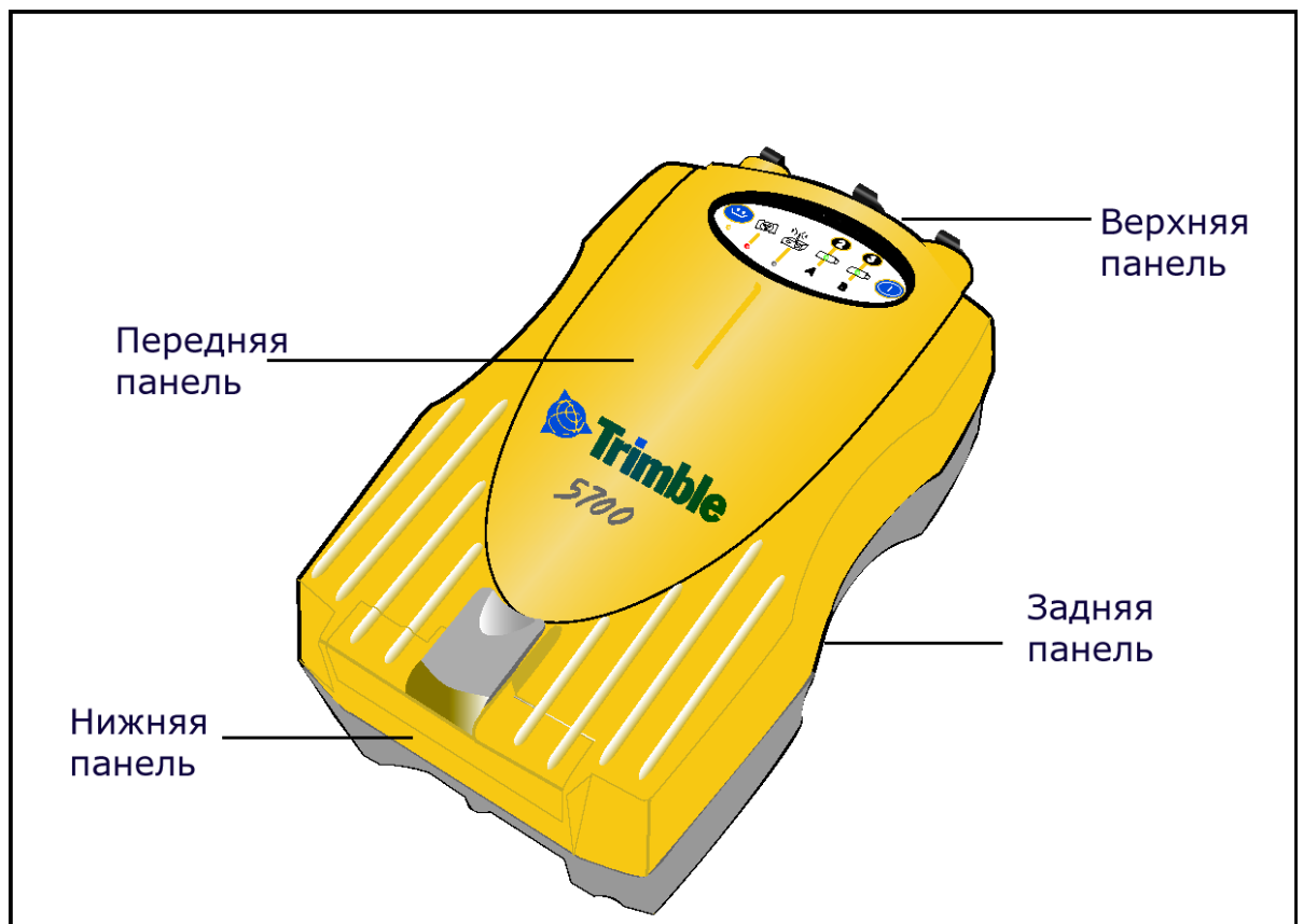
Рис. 2.1 Панели приемника 5700
