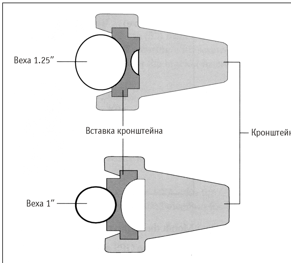
Рис. 2.8 Вставка кронштейна приемника
