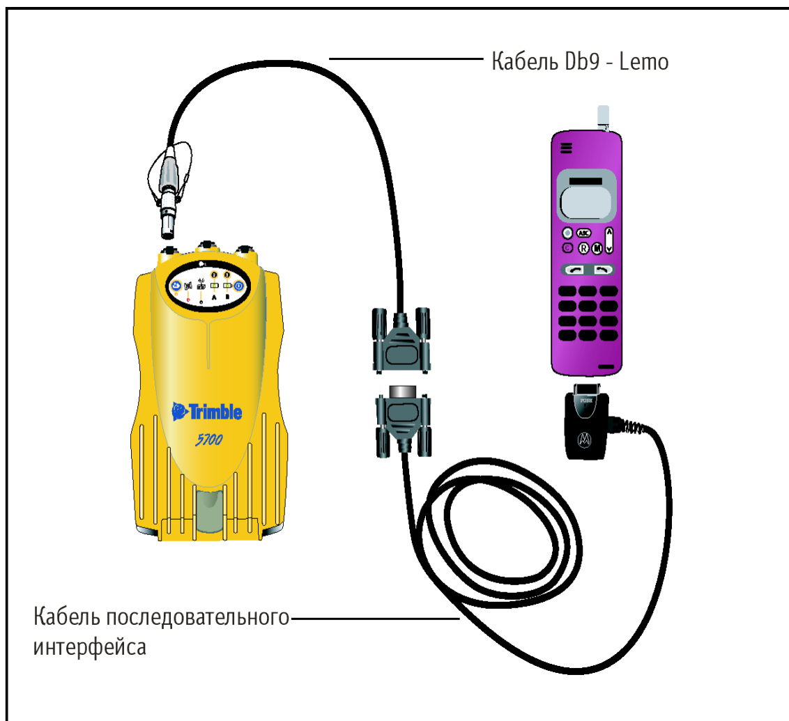
Рис. 2.12 Подключение внешнего модема
