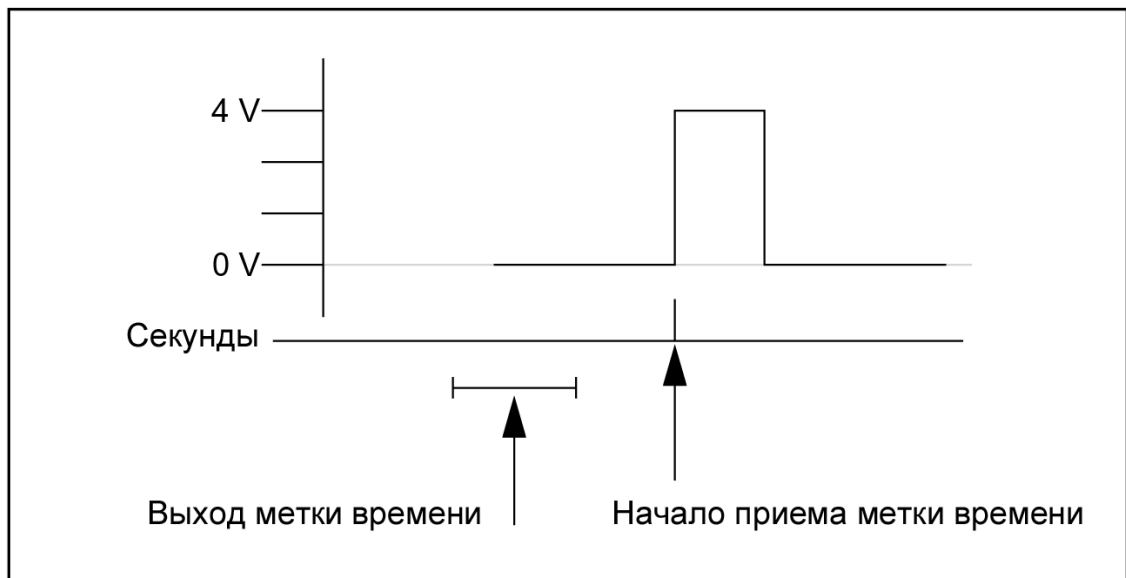
Рис. 13.1 Связь метки времени и синхроимпульса 1 Гц
