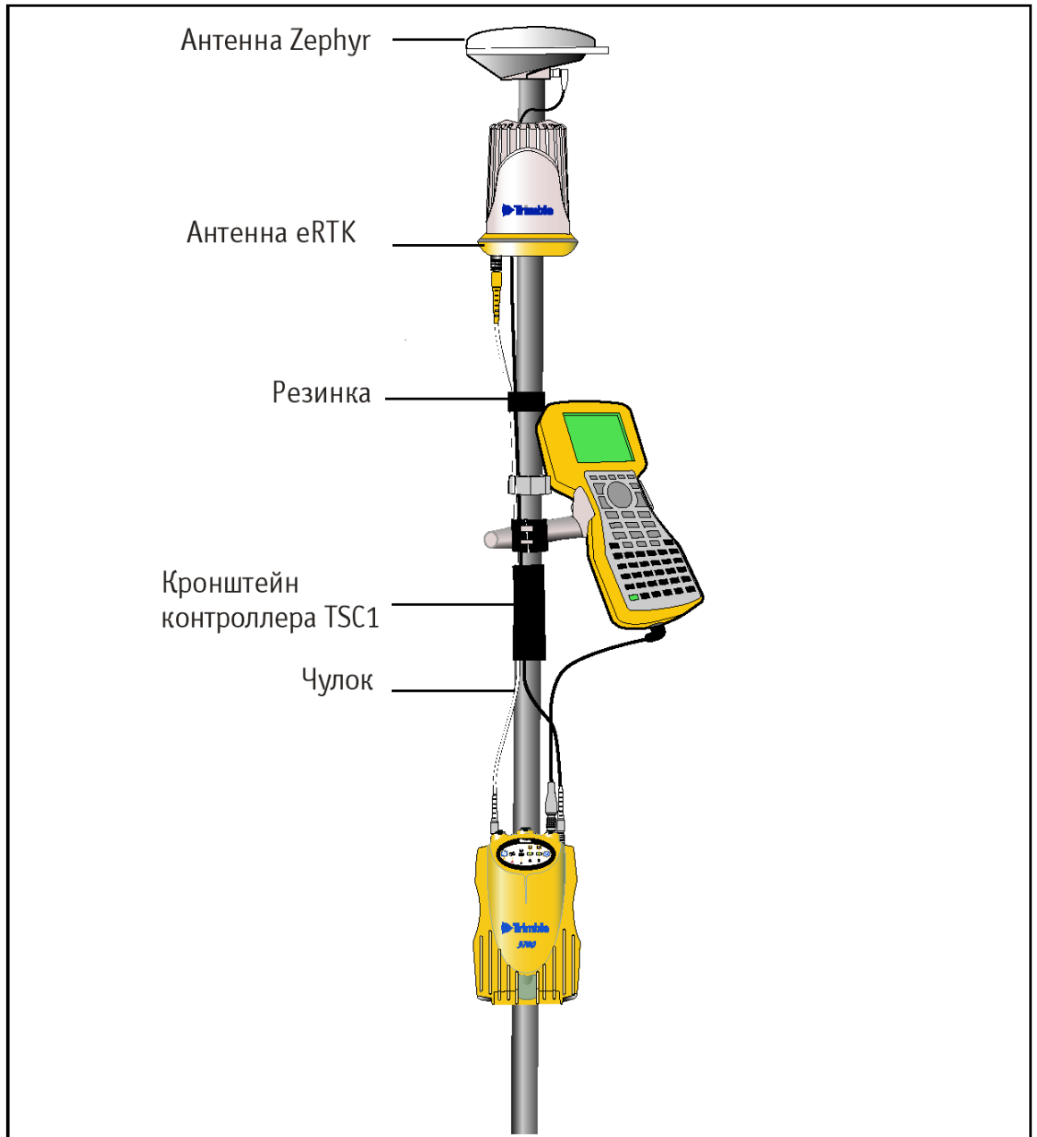
Рис. 2.10 Размещение приемника на вехе
