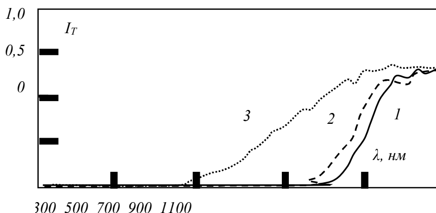
Расм-2. Турли қалинликдаги кремний пластинаси нур ютиш кўрсаткичининг нур тўлқин узунлигига боғланиш графиги: 1- d=200 мкм; 2- d=100 мкм; 3- d=10 мкм.
