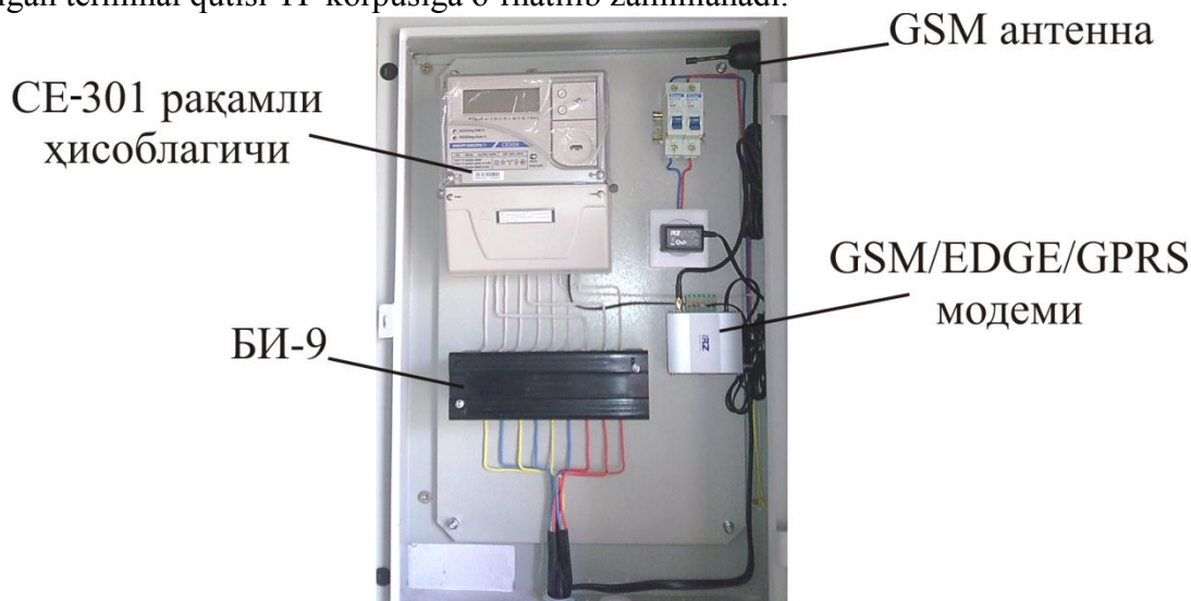
2.-rasm. elektr energiyani xisobga olishniig nazorat qilishdagi avtomatlashtirilgan tizimini hisobga olish terminalini ko'rinishi
