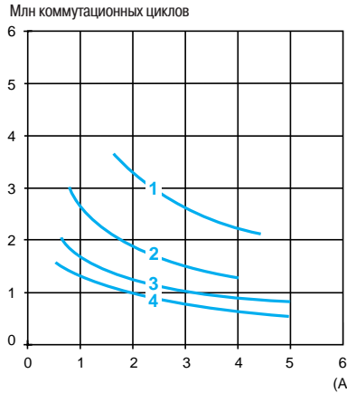
AC-13: управление статическими нагрузками с развязкой посредством трансформатора \cos \varphi \geq 0,65
