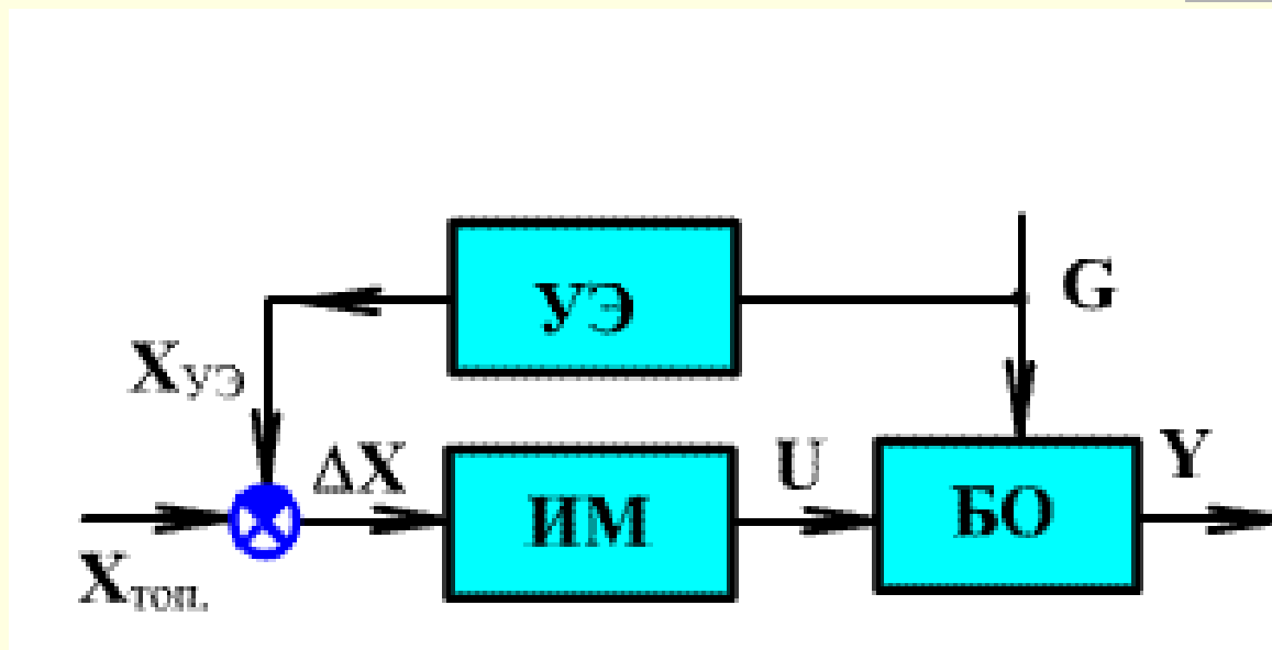
Ўзгармас ток генератори кучланишини тойдирувчи таъсир бўйича ростлашнинг функционал схемаси
