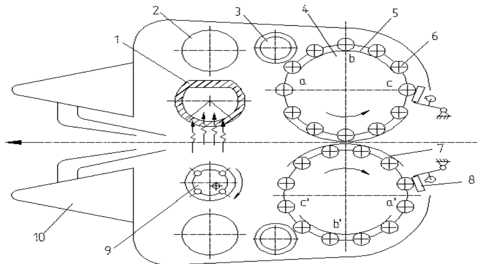
1-расм. Шпиндел сиртидаги нукталар кинематикаси (а) ва тишчаларнинг пахтага ишончли кадалишини асослашга оид схема (б): 1- шпинделли барабан элементи; 2- механик шпиндел; 3- пахта пилтаси.
