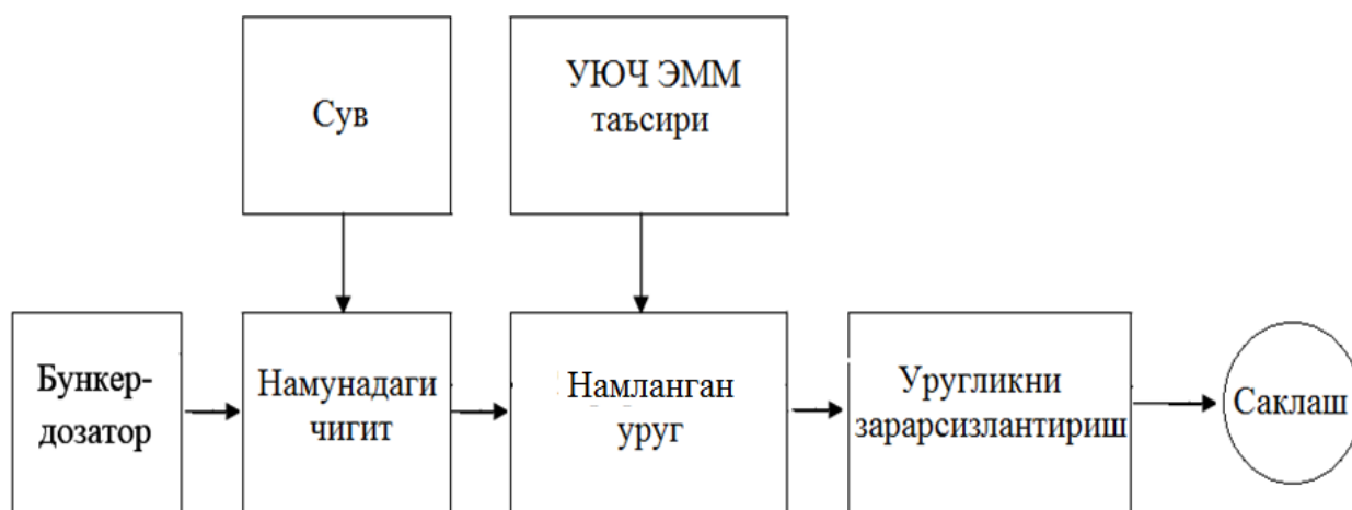
1 – расм. Ўта юқори частотали электромагнит майдон ёрдамида уруғлик чигитни зарарсизлантиришнинг технологик схемаси.
