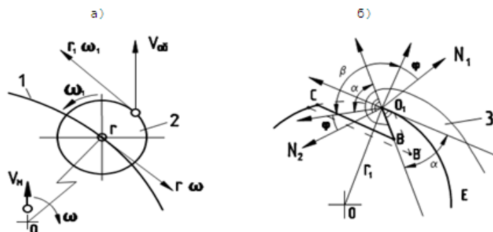
1-расм. Шпиндел сиртидаги нукталар кинематикаси (а) ва тишчаларнинг пахтага ишончли кадалишини асослашга оид схема (б): 1- шпинделли барабан элементи; 2- механик шпиндел; 3- пахта пилтаси.
