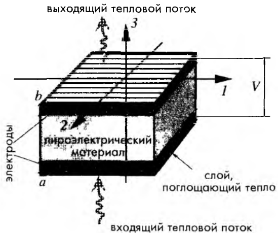
Рис. 3.26 Пирозлектрический датчик имеет два электрода, расположенных на противоположных сторонах кристалла. Тепло поступает снизу вдоль оси 3 и оттекает
