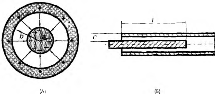
Рис. 3.5 А — цилиндрический конденсатор, В — емкостной датчик перемещения
