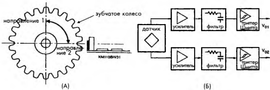
Рис. 7.22. А – оптимальное рабочее положение магниторезистивного модуля. Отметим, что магнит находится за датчиком, Б – принципиальная схема модуля
