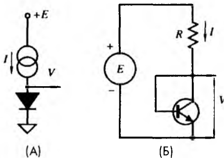
Рис. 16.19. Датчики температуры на основе прямосмещенного р-п перехода: А — диод, Б — транзистор, включенный по схеме диода
