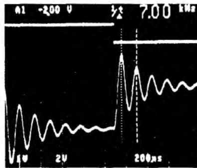
Рис. 14.9. Выходной сигнал фотодиода без использования компенсационной цепи. (Напечатано с разрешения Nitta-matsu Photonics К.К.)
