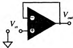
Рис. 5.7. Повторитель напряжений, реализованный на ОУ
