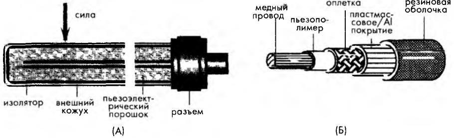
Рис. 8.15. Датчики в виде пьезоэлектрических кабелей. А – устройство кабеля Vibrocaox, Б – полимерная пленка, используемая как компонент, вырабатывающий напряжение [13]
