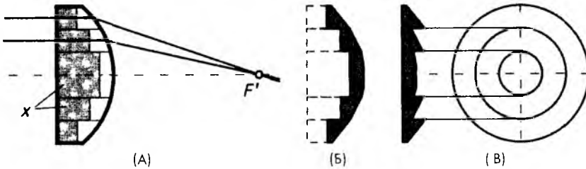
Рис. 4.13 Концепция линз Френеля
