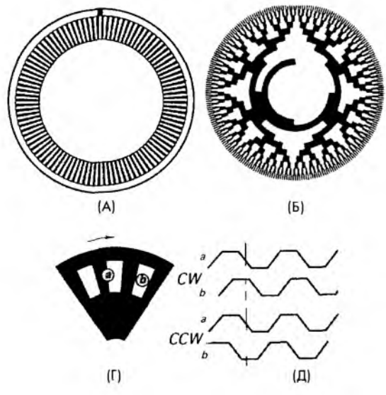
Рис. 7.34. Диски оптических шифраторов перемещений: А – дискретных, Б – абсолютных. При вращении диска по часовой стрелке (CW) сигнал a опережает сигнал b на 90° (В), а при вращении против часовой стрелки (CCW) – сигнал a отстает от b на 90° (Г).
