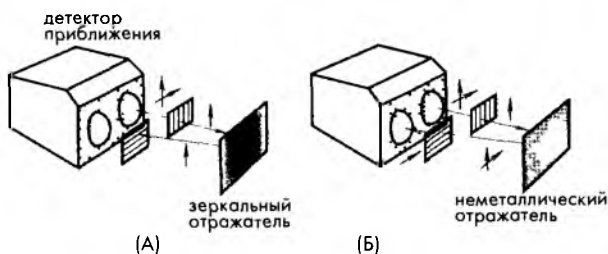
Рис. 7.27. Детектор приближения с двумя поляризационными фильтрами, расположенными под углом 90^\circ друг к другу А – поляризованный свет отражается от металлического объекта, не меняя направление поляризации, Б – диэлектрический объект меняет направление поляризации отраженного света, что позволяет ему пройти через поляризационный фильтр
