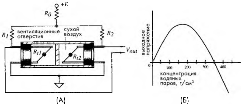
Рис. 13.8. Датчик абсолютной влажности с саморазогревающимися термисторами. А — схема и электрические соединения. Б — зависимость выходного напряжения от влажности
