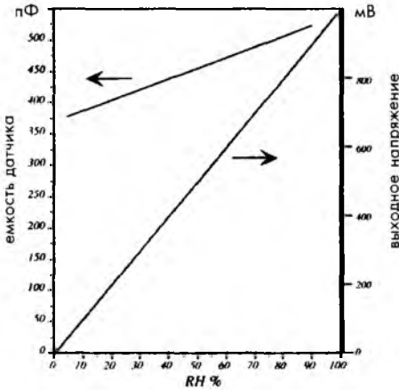
Рис. 13.2. Передаточная функция емкостного датчика и системы
