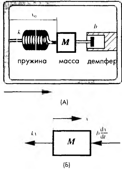
Рис. 3.49. А – механическая модель акселерометра, В – диаграмма сил, действующих на свободное тело массы M
