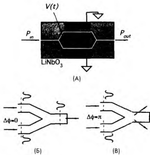
Рис. 4.23. А – каналный интерферометрический модулятор интенсивности излучений, Б – сдвиг фаз равен нулю, выходное излучение двух ветвей суммируется, В – при сдвиге фаз, равному \pi , все излучение уходит в подложку, и выходное излучение равно нулю. (Рисунок взят из [12])
