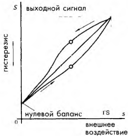
Рис. 2.4 Передаточная функция с гистерезисом
