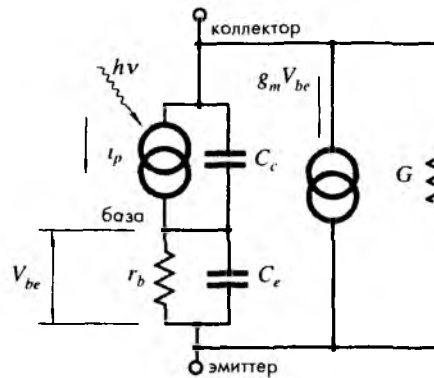
Рис. 14.12. Эквивалентная схема фототранзистора
