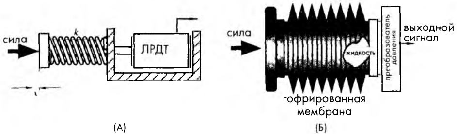
Рис. 9.1. А – датчик силы с нагружаемой пружиной и ЛРДТ, Б – датчик силы на основе преобразователя давления
