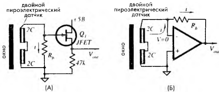
Рис. 14.22. Преобразователи импеданса для пирозлектрических датчиков: А — повторитель напряжений на полевом транзисторе, Б — преобразователь ток-напряжение на ОУ
