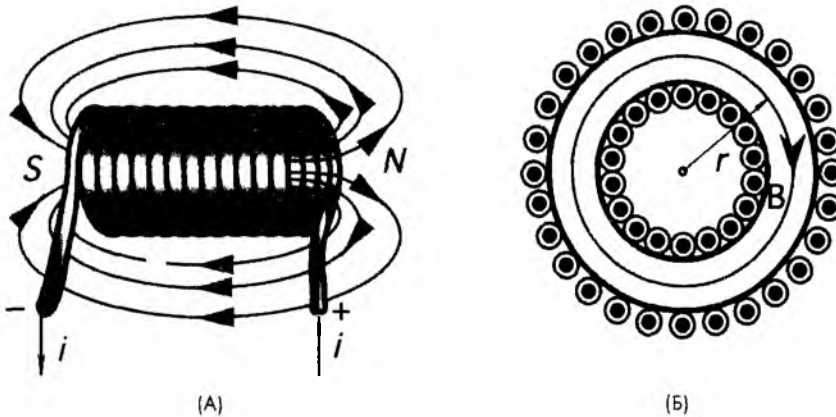
Рис. 3.14. А – соленоид, Б – тороид
