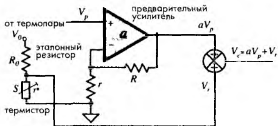
Рис. 16.17. Суммирование сигналов термистора и термопары
