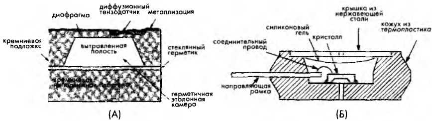
Рис. 10.7. Устройство корпусов датчиков: А — абсолютного, Б — дифференциального давлений (напечатано с разрешения Motorola Inc)
