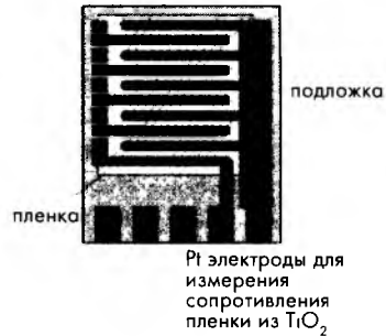
Рис. 17.10. Фотокаталитический газовый микродатчик
