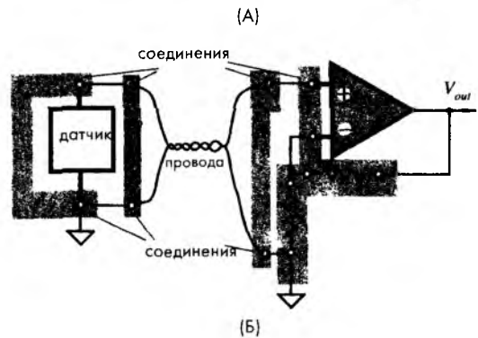
Рис. 5.56. А — эдс Зеебека, генерируемая на соединениях припой — медь [17], Б — поддержание одинаковой температуры соединений снижает термоэдс
