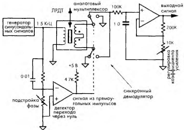
Рис. 7.10. Упрощенная схема датчика перемещений на основе ЛРДТ с интерфейсом
