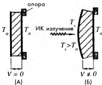
Рис. 6.13. Упрощенная модель пироэлектрического эффекта, как следствия пьезоэлектричества. Первоначально элемент имеет равномерную температуру (А); под действием теплового излучения передняя сторона элемента расширяется, что приводит к появлению на электроде зарядов (Б)
