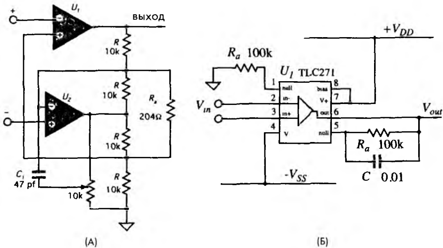
Рис. 5.9. А — измерительный усилитель на двух ОУ, Б — недорогой измерительный усилитель на одном ОУ
