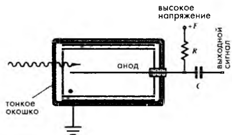
Рис. 15.5. Схема счетчика Гейгера-Мюллера. Символ «•» указывает газ
