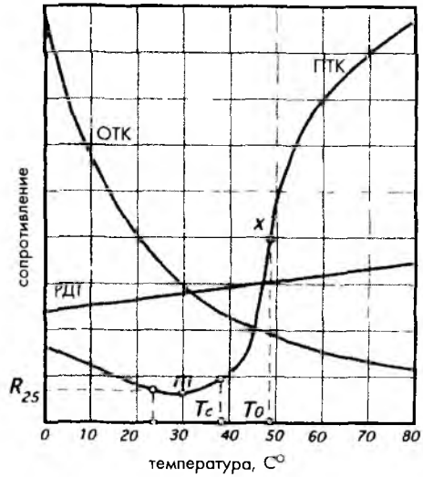
Рис. 16.12. Передаточные функции для термисторов с ОТК, ПТК и РДТ
