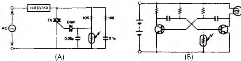
Рис. 14.15. Примеры применения фоторезисторов: А – схема управления включением света, Б – схема маяка.
