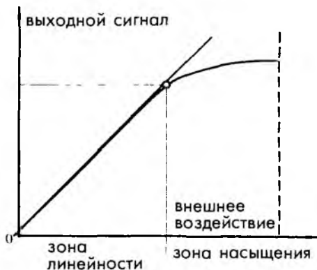
Рис. 2.6 Передаточная функция с насыщением
