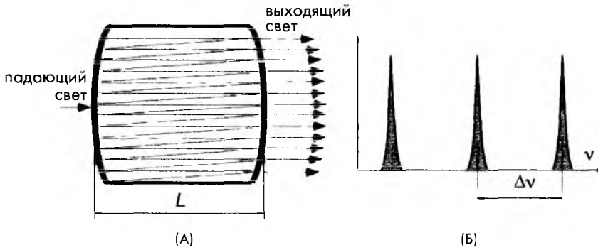
Рис. 7.30. А – многократная интерференция внутри резонатора Фабри-Перо, Б – импульсы света на выходе резонатора
