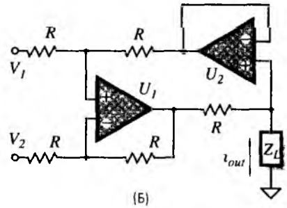
Рис. 5.15. Генератор тока для подключения заземленной нагрузки А – токовый генератор Холленда, В – токовый генератор на двух ОУ
