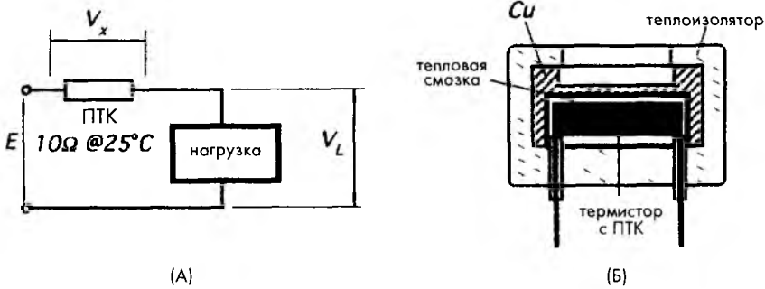
Рис. 16.14. Применение термисторов с ПТК А – в схемах ограничения тока, Б – в микротермостатах
