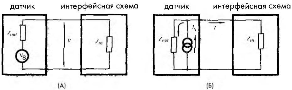
Рис. 2.8 Соединение датчика с интерфейсной схемой А – датчик с выходным сигналом в виде напряжения, Б – датчик с токовым выходом
