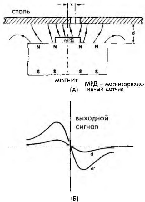
Рис. 7.20. Измерение линейных перемещений при помощи магниторезистивного датчика КМЗ10: А – датчик расположен между постоянным магнитом и металлической пластиной, Б – выходной сигнал при разном расстоянии между магнитом и пластиной.
