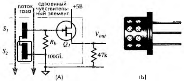
Рис. 11.15. Пьезоэлектрический детектор изменения скорости потока: А – схема датчика, Б – корпус датчика ТО-5
