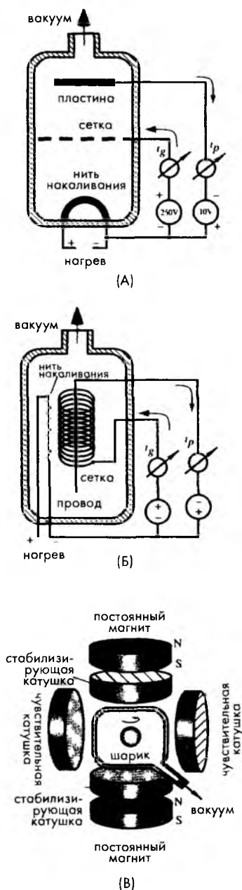
Рис. 10.16. Ионизационный вакуумный датчик (А), измеритель Баярда-Алперта (Б), датчик газового сопротивления (B)
