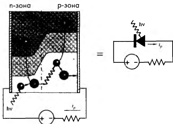
Рис. 14.3. Структура фотодиода
