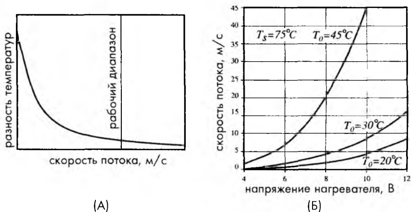
Рис. 11.5. Передаточная функция термоанемометра (А) и калибровочные кривые для детектора температуры термоанемометра с саморазогревом, определенные при трех разных уровнях нагрева (Б)
