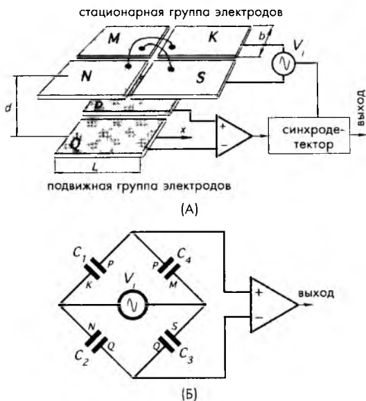
Рис. 7.8. Емкостной датчик мостового типа с параллельными пластинами: А – устройство групп электродов, Б – эквивалентная схема
