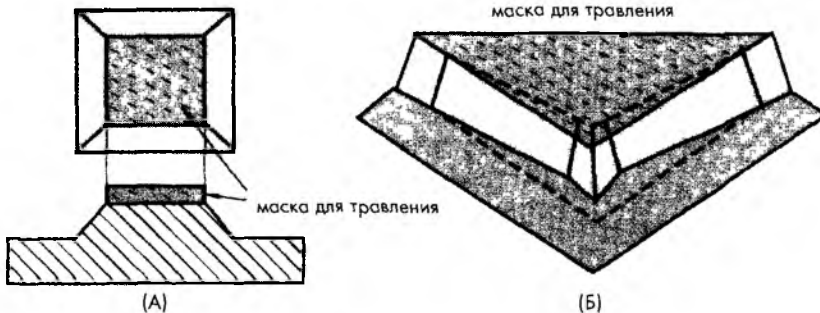
Рис. 18.11. Мезаструктуры
