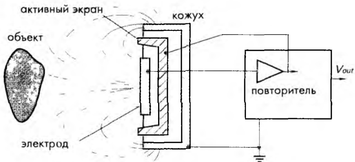
Рис. 7.7. Емкостной датчик, измеряющий расстояние до объекта, с активным экраном вокруг электрода
