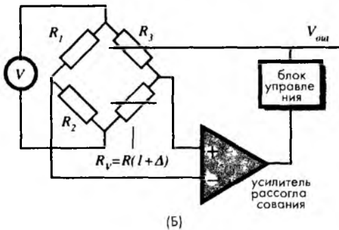
Рис. 5.37. Два способа использования мостовой схемы А – неуравновешанный мост, Б – уравновешенный мост с управляемой ОС
