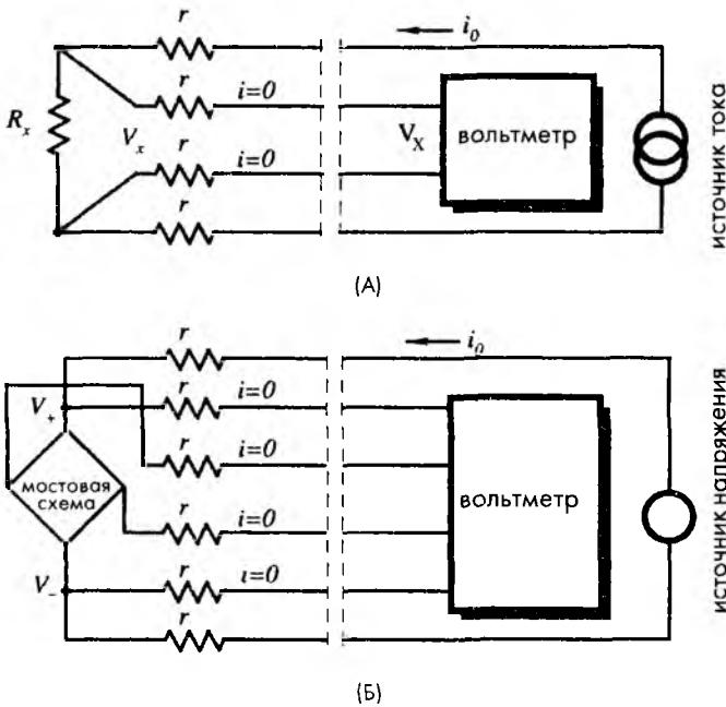
Рис. 5.43. Дистанционное измерение сопротивлений: А-четырёхпроводной метод, Б – шестипроводный метод, применяемый с мостовыми схемами
