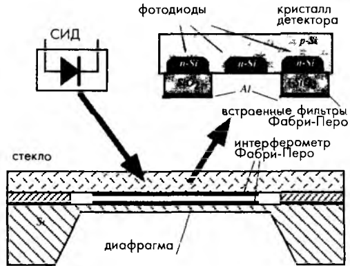
Рис. 10.13. Схема оптоэлектронного датчика давления, использующего принцип интерференции света [12]
