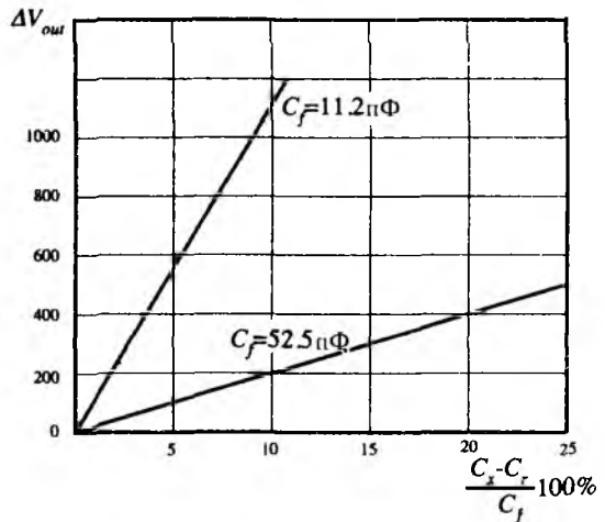
Рис. 5.33. Передаточная функция преобразователя в напряжение при двух значениях интегрирующего конденсатора [6].
