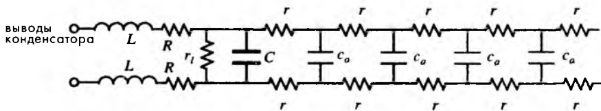
Рис. 5.51. Эквивалентная схема конденсатора
