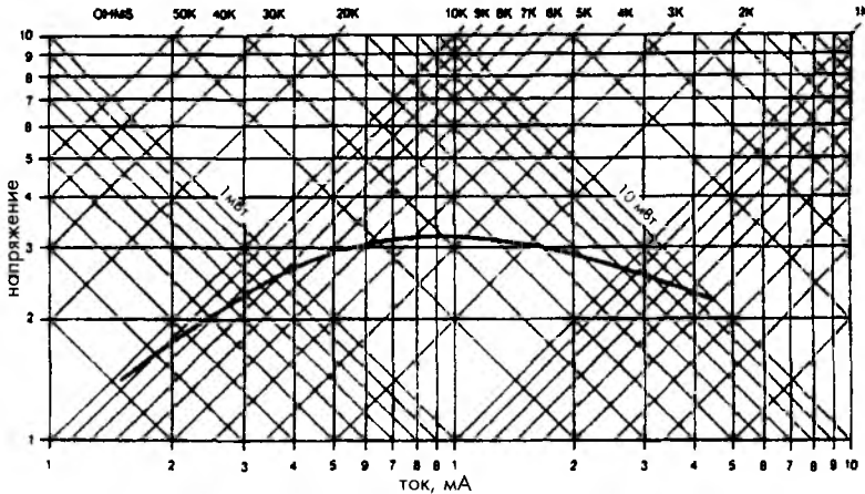
Рис. 16.11. Зависимость напряжения от тока для термисторов с ОТК, работающих в спокойной воздушной среде при температуре 25^\circ\text{C} . Нелинейность характеристики объясняется эффектом саморазогрева
