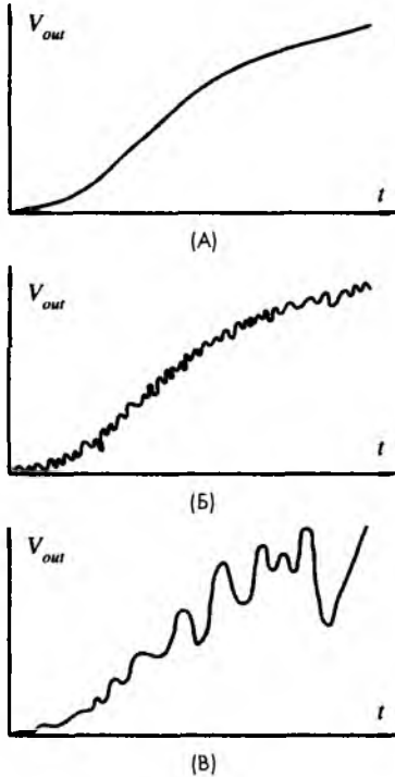
Рис. 5.46. Разновидности помех: А — полезный сигнал, Б — аддитивный шум, В — мультипликативный шум
