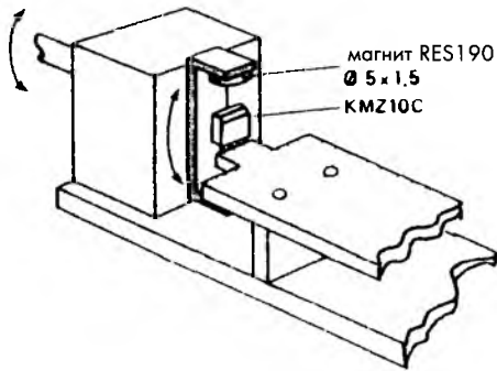
Рис. 7.21. Измерение угловых перемещений при помощи датчика KMZ10C
