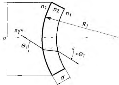
Рис. 4.7. Сферическое окно
