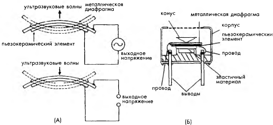
Рис. 7.40. Пьезоэлектрический ультразвуковой преобразователь А – входное напряжение приводит к изгибу элемента, что вызывает генерацию ультразвуковых волн И наоборот, в результате воздействия волн на выходе преобразователя появляется напряжение, Б – ультразвуковой преобразователь с открытой апертурой для работы в воздухе ( напечатано с разрешения Nippon Ceramic, Japan )
