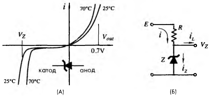
Рис. 5.17. Стабилитрон А – вольт-амперная характеристика, Б – стабилизатор шунтирующего (параллельного) типа
