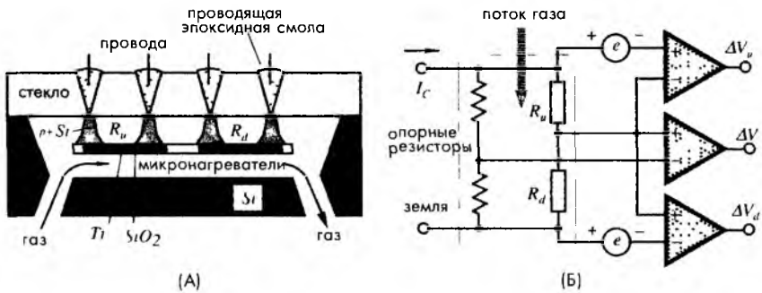
Рис. 11.13. Микротермоанемометр с саморазогревающимися титановыми резисторами А – конструкция датчика, Б – эквивалентная схема датчика с интерфейсом R_u и R_d – сопротивления нагревателей, расположенных выше и ниже по течению потока [7]
