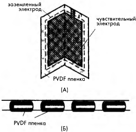
Рис. 12.5. Пьезоэлектрический звукосниматель складного типа (А), устройство гидрофона на основе свернутых PVDF пленок (Б)
