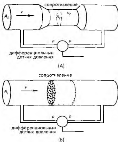
Рис. 11.3. Два типа элементов, оказывающих сопротивление потоку: узкий участок трубки (А) и пористая пробка (Б)
