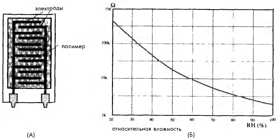
Рис. 3.20 А – схема гигристора, Б – его передаточная функция
