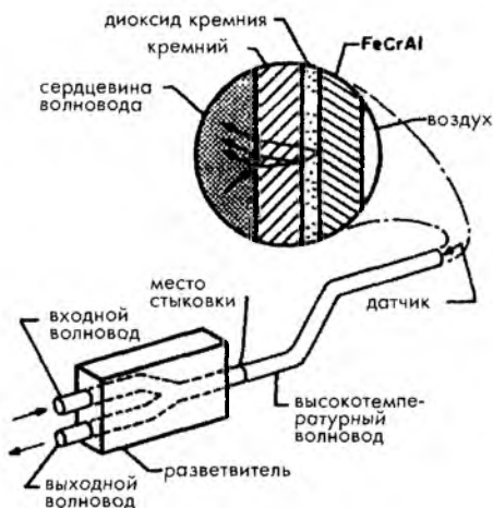
Рис. 16.26. Схема тонкопленочного оптического датчика температуры
