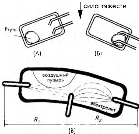
Рис. 7.3. Гравитационные датчики: А — ртутный переключатель в разомкнутом состоянии, Б — ртутный переключатель в замкнутом состоянии, В — электролитический детектор наклона
