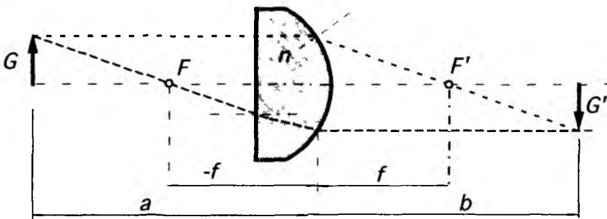
Рис. 4.12. Геометрия плосковыпуклой линзы
