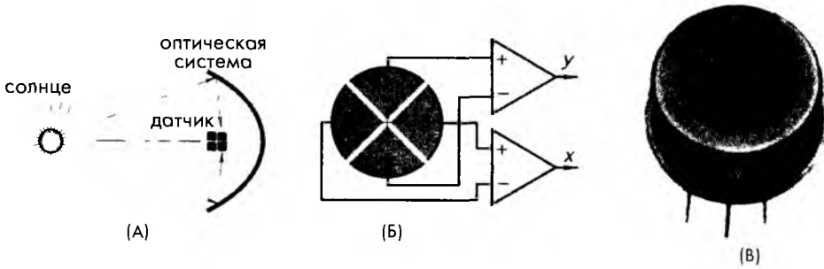
Рис. 7.25. Четырехквadrантный фотодетектор: А – фокусирование объекта на датчик, Б – подключение чувствительных элементов к дифференциальным усилителям, В – внешний вид датчика.
