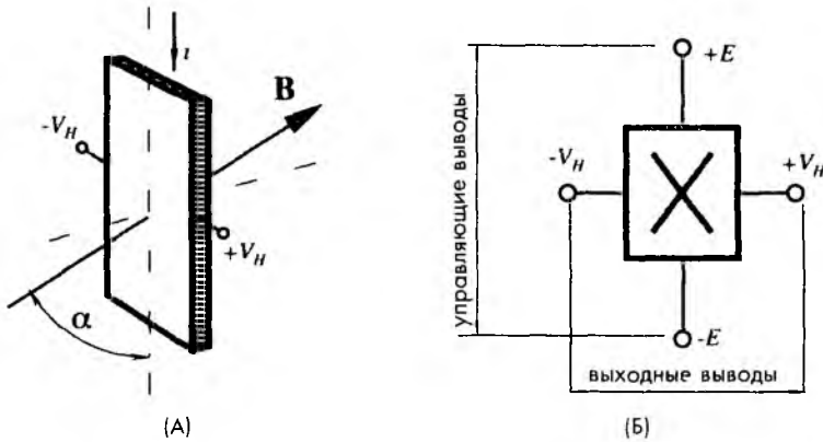
Рис. 3.31. А – выходной сигнал датчика Холла зависит от угла между вектором магнитного поля и плоскостью пластины, Б – четыре вывода датчика Холла
