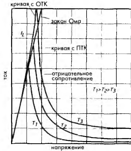
Рис. 16.13. Вольтамперная характеристика детектора с ПТК
