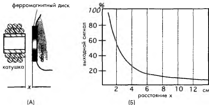
Рис. 7.13. Поперечный датчик приближения с дополнительным ферромагнитным диском (А) и зависимость выходного сигнала от расстояния (Б)
