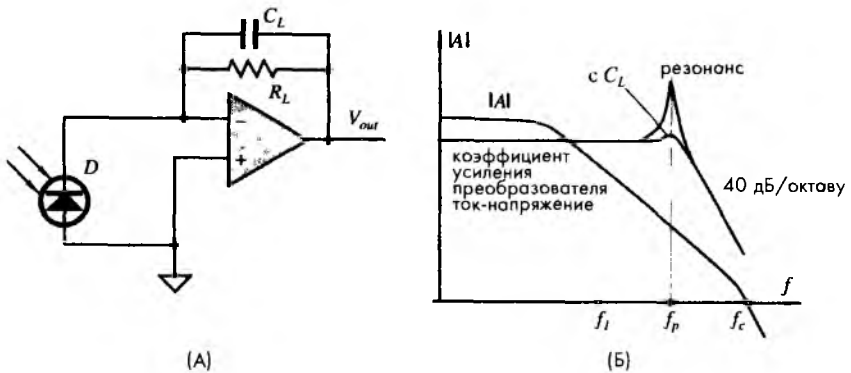
Рис. 14.8. Применение преобразователя тока в напряжение (А) и АЧХ двух схем включения фотодиодов (Б)
