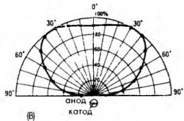
Рис. 14.30. УФ детектор пламени. А – стеклянная трубка, заполненная газом, Б – схема включения, В – угол обзора в горизонтальной плоскости (Напечатано с разрешения Hamamatsu Photonics К.К.)
