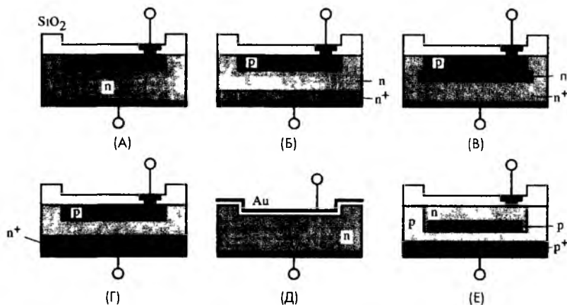
Рис. 14.6. Упрощенные структуры шести типов фотодиодов
