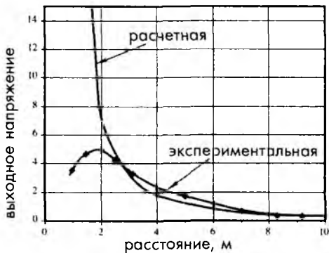
Рис. 6.17. Расчетная и экспериментальная зависимости амплитуды выходного сигнала ПИК детектора движения от расстояния до объекта
