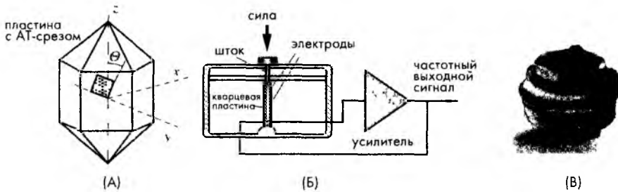
Рис. 9.13. Кварцевый датчик силы: А – АТ срез кварцевого кристалла, Б – структура датчика, В – внешний вид (напечатано с разрешения Quartzcell, Santa Barbara, CA)
