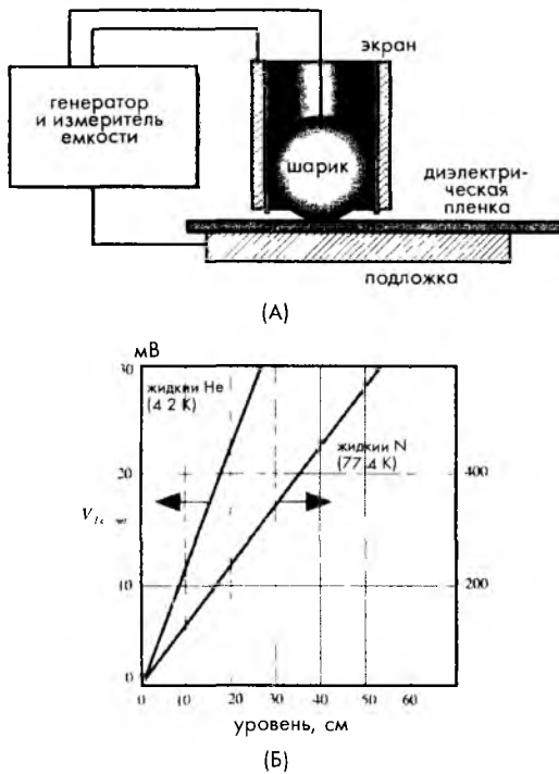
Рис. 7.48. Емкостной датчик для измерения толщины сухой диэлектрической пленки (А) и форма передаточной функции (Б) [16]
