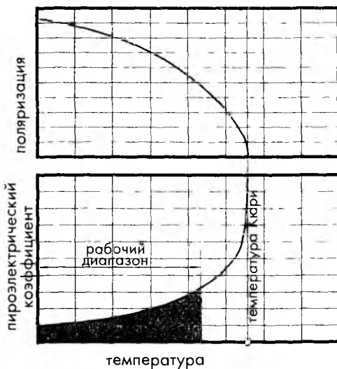
Рис. 3.28. Поляризация пьезоэлектрического кристалла. Датчик должен работать и храниться при температурах, значительно меньших точки Кюри
