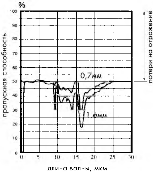
Рис. 4.8. Спектральная пропускная способность кремниевых окон. Отметим, что большая часть потерь связана с отражением от двух поверхностей
