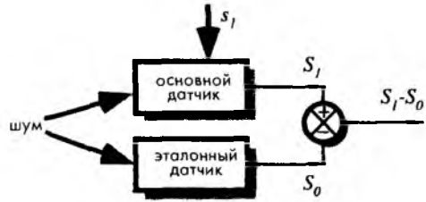
Рис. 5.47. Дифференциальный метод снижения аддитивных помех
