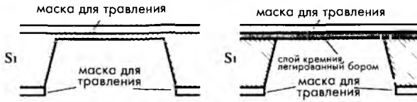
Рис. 18.12. Изготовление диафрагмы или мембраны
