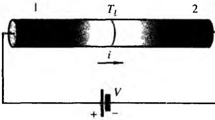
Рис. 3.37. Эффект Пельтье
