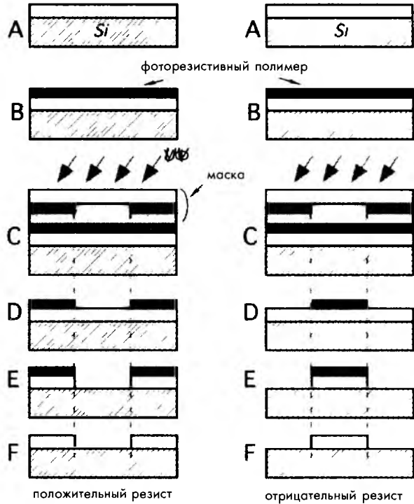
Рис. 18.8. Положительная и отрицательная фотолитография
