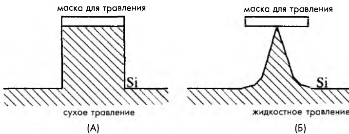
Рис. 18.15. Вытравливание остrokонечных структур
