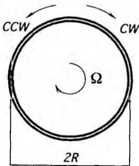
Рис. 8.13. Эффект Саньяка
