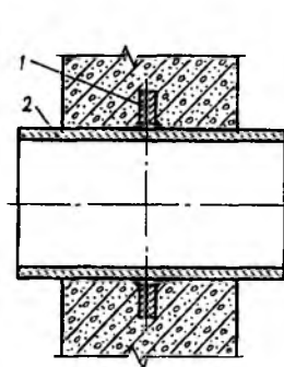
Рис. 6.1. Жесткая заделка трубопровода с применением ребристого патрубка:
