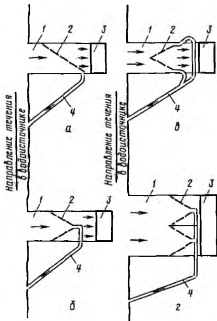
Рис. 2.6. Схемы установки вертикальных плоских экранов (сетчатых) рыбозаградителей на водозборных сооружениях:
