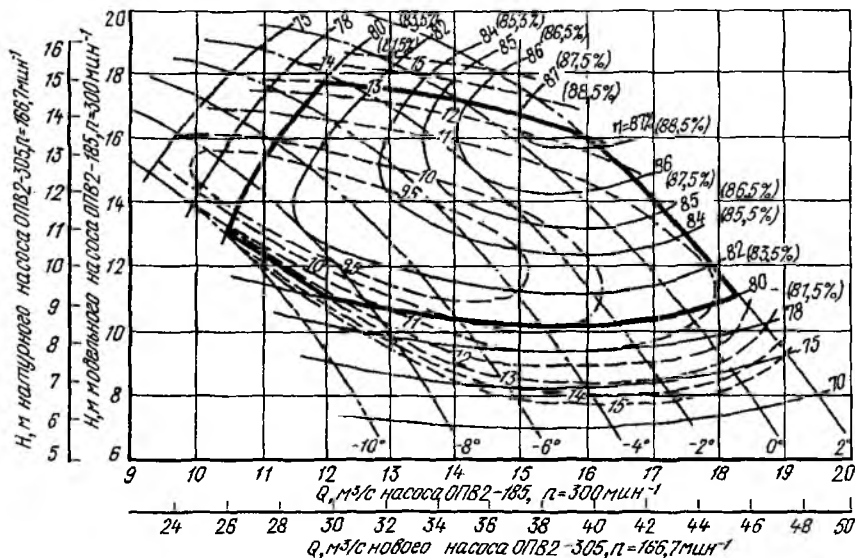
Рис. 4.5. Характеристики модельного насоса ОПВ2-185 при n = 300 \text{ мин}^{-1} и нового ОПВ2-305 при n = 166,7 \text{ мин}^{-1} (в скобках — КПД нового насоса, пунктирные линии — кавитационные характеристики модельного насоса по первому критическому режиму)
