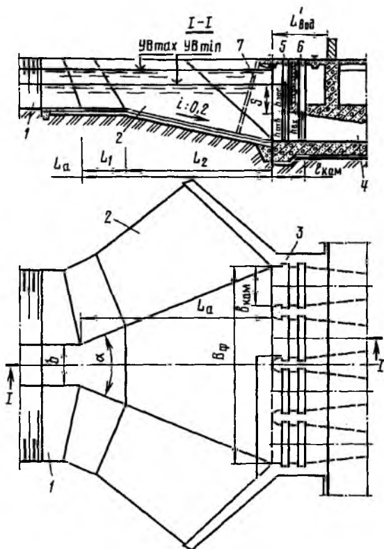
Рис. 3.2. Схема водозаборного сооружения (совмещенная компоновка) насосной станции на тупиковом канале:
