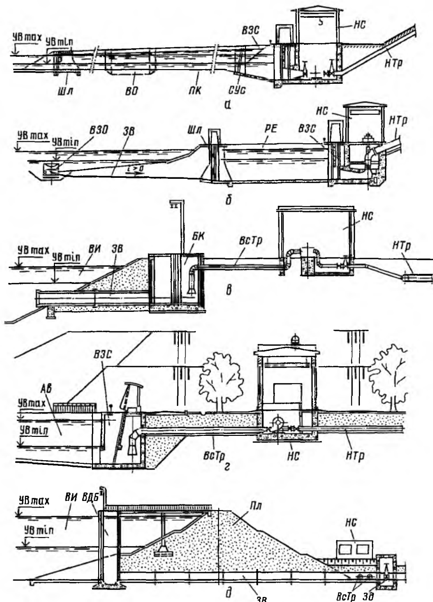
Рис. 1.13. Схемы узлов насосных станций с конструктивным изображением отдельных сооружений (без водовыпускных сооружений) при заборе воды: а — из реки через шлюз и подводный канал с водоотстойником; б — через донные оголовки при наличии регулирующей емкости перед зданием насосной станции; в — с береговым колодцем; г — из тупикового канала; д — при расположении здания насосной станции в нижнем бьефе водохранилища; Зд — задвижка. (Остальные обозначения см. рис. 1.6 и 1.10.)
