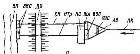
Для осушительных систем. 1. С забором воды из открытого канала-коллектора (рис. 1.10, а).
