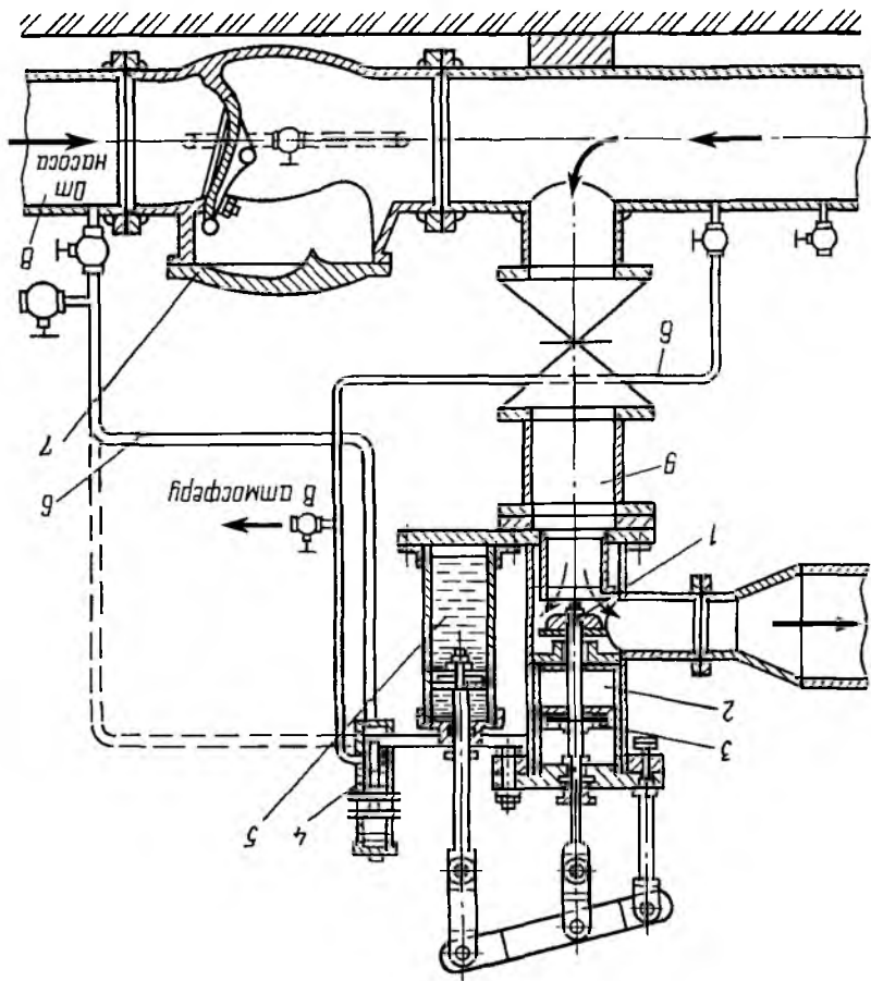
Рис. 7.13. Клапан-распределитель Укрводтео:
