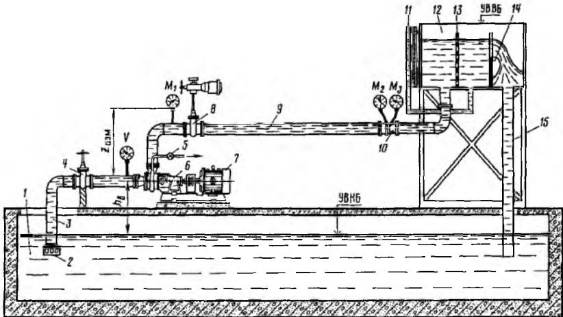
Рис. 10.8. Схема стэнда для испытаний насосов:
