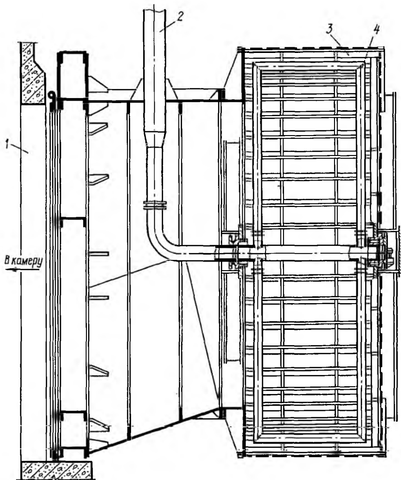
Рис. 2.8. Сетчатый струереактивный рыбозаградитель:
