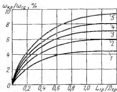
Рис. 8.10. График зависимости
