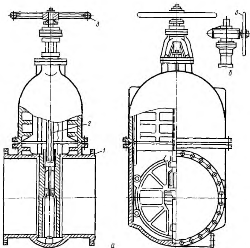
Рис. 6.11. Параллельные задвижки с неподвижным шпинделем на давлении p_y = 1 МПа:
