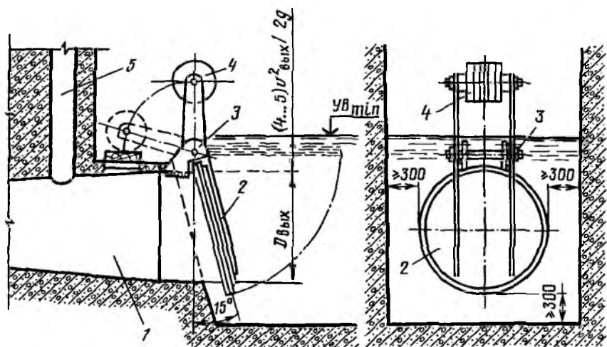
Рис. 8.2. Клапан-захлопка:
