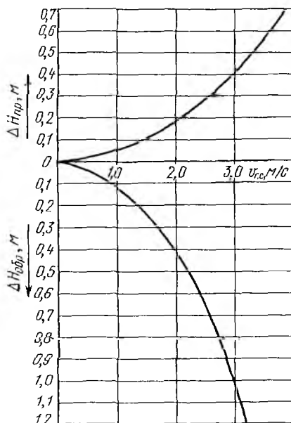
Рис. 8.9. График зависимости \Delta H = f(v_{гс})
