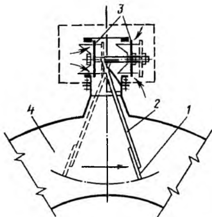
Рис. 8.8. Схема гидромеханического клапана срыва вакуума (конструкция Союзгипроводхоза):
