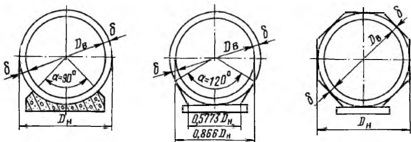
Рис. 7.4. Рекомендуемые сечения труб из монолитного железобетона
