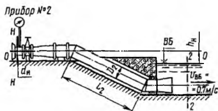
Рис. 11.3. Расчетная схема напорной линии насосной установки для определения показаний прибора № 2 (см. рис. 11.1)
