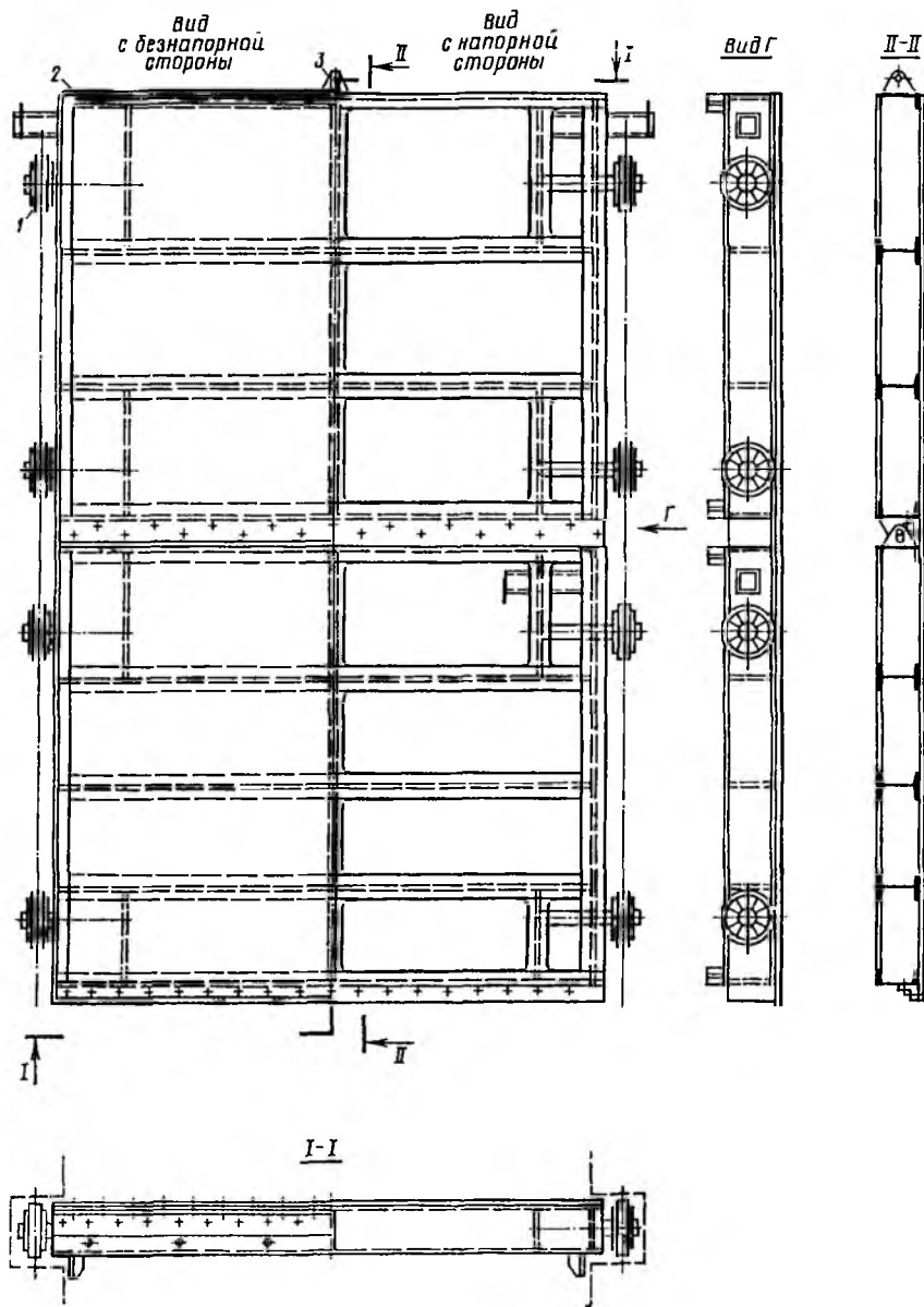
Рис. 4.12. Схема плоского ремонтного колесного затвора:
