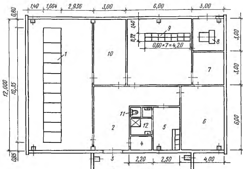
Рис. 5.15. Схема компоновки электромашинных помещений насосных станций, оборудованных шестью насосами ДБ300-27 с электродвигателями мощностью 630 кВт (размеры в м):
