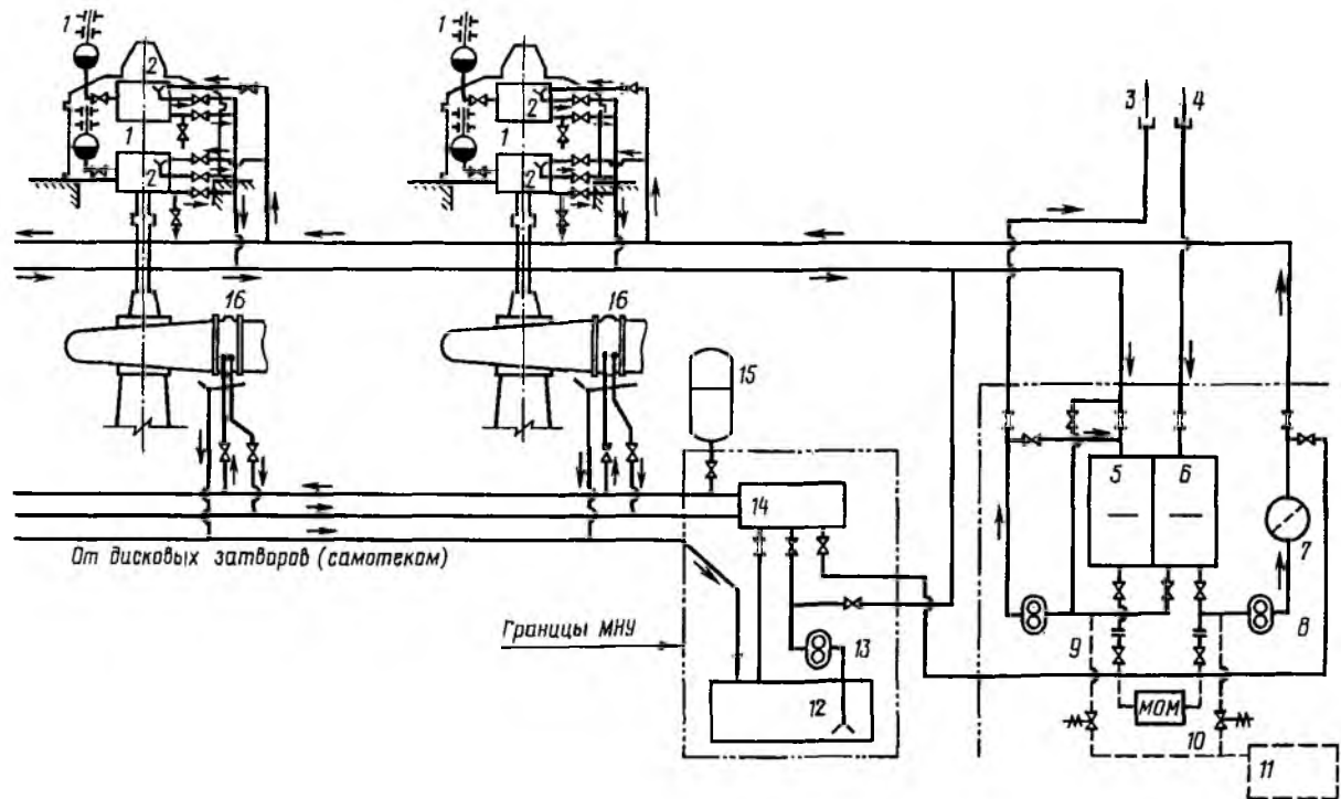
Рис. 4.11. Схема маслоснабжения крупной насосной станции, оборудованной центробежными насосами и дисковыми затворами с гидроприводом:
