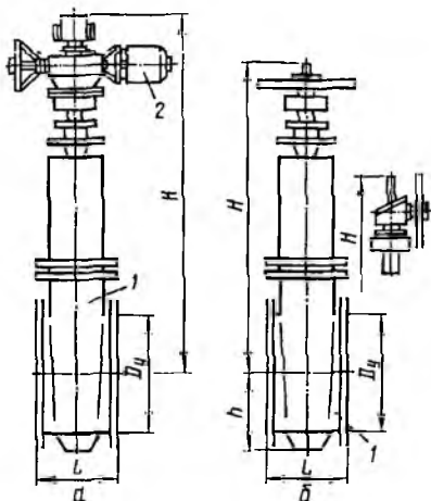
Рис. 6.14. Клиновая задвижка с невыдвигным шпинделем фланцевая укороченной длины на давление 0,25 МПа:
