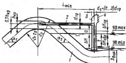
Рис. 8.7. Схема гидравлического клапана срыва вакуума (конструкция Укргипроводхоза):
