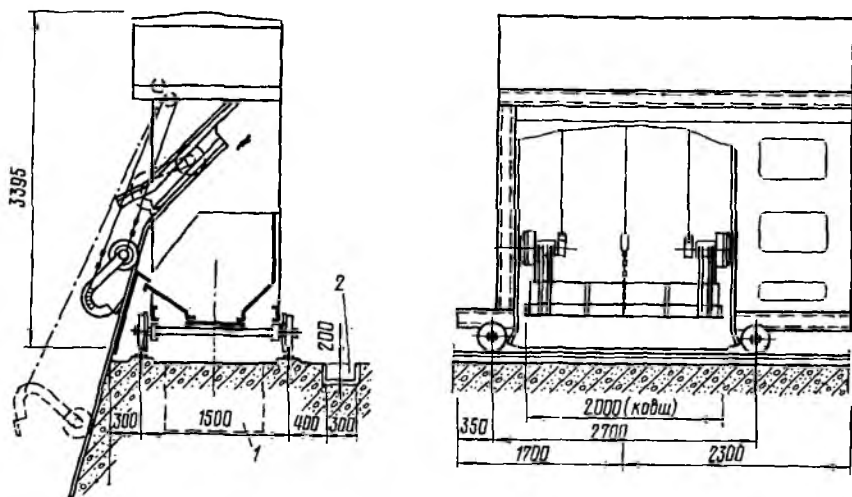
Рис. 4.14. Схема решеткоочистительной машины РН-2000:
