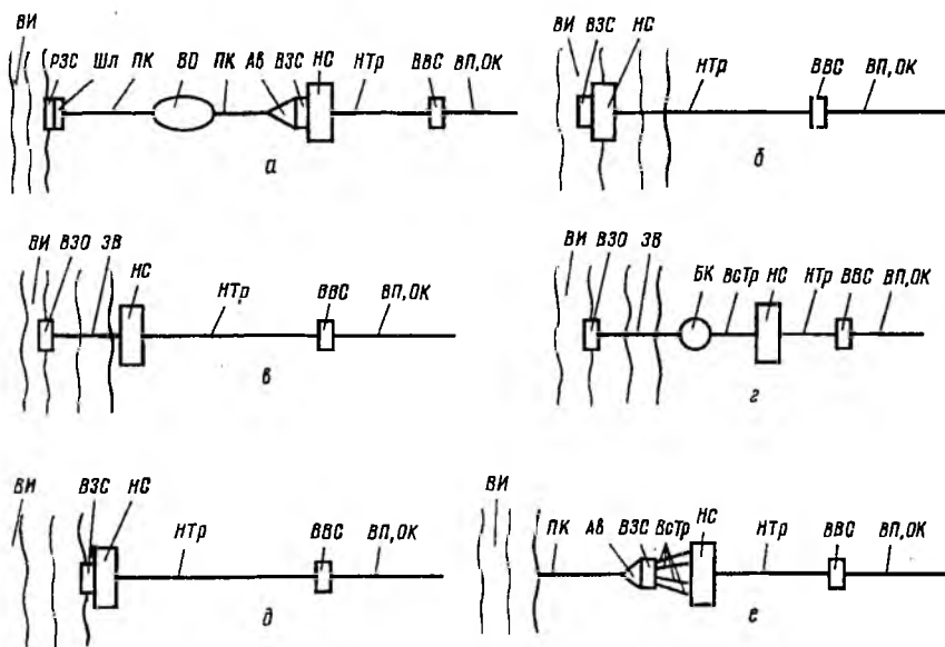
Рис. 1.6. Схемы узлов насосных станций для оросительных систем:
