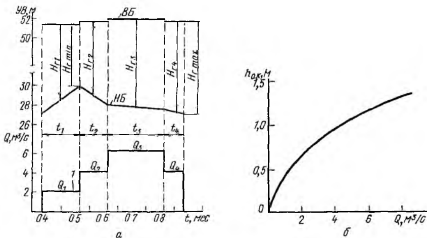
Рис. 4.1. Совмещенный график колебаний (а) и зависимость глубины воды в отводящем канале h_{ок} от пропускаемого через него расхода воды Q (б):
