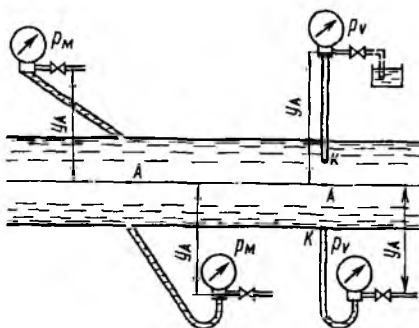
Рис. 10.2. Схемы измерения давления и вакуума
