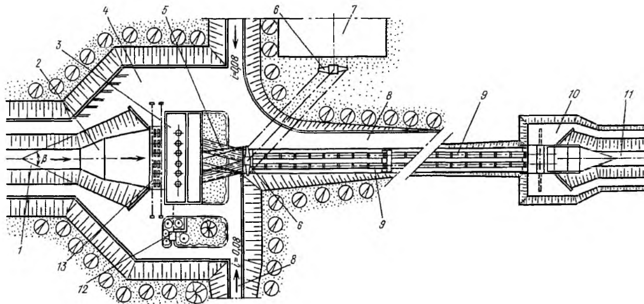
Рис. 1.3. Генеральный план насосной станции на тупиковом канале:
