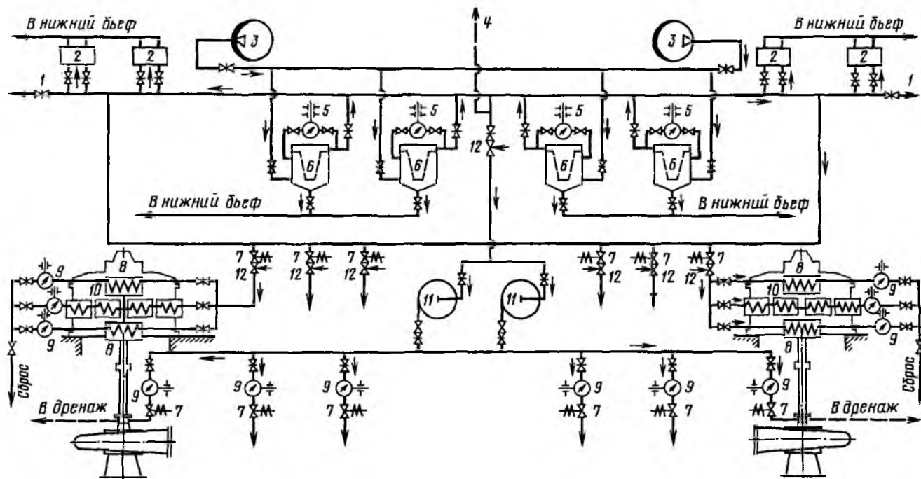
Рис. 4.10. Схема ТВС для крупной насосной станции:
