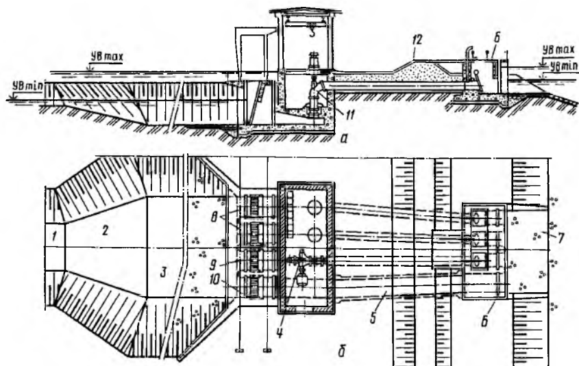
Рис. 5.7. Осушительная насосная станция на коллекторе:
