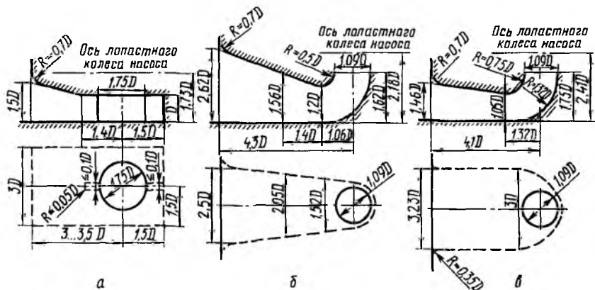
Рис. 6.8. Схемы подводящих труб с камерным (а) и коленчатым (б — форма 1, суженная в плане, в — форма 2, расширенная в плане) подводом воды ( D — диаметр входного патрубка центробежного насоса или диаметр рабочего колеса осевого насоса)
