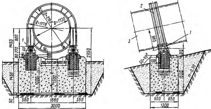
Рис. 7.8. Промежуточная опора каткового типа:
