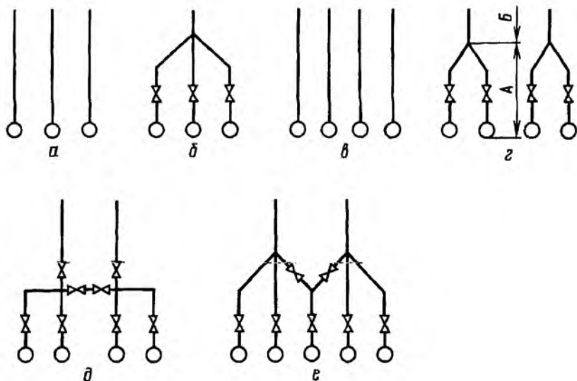
Рис. 9.1. Схемы соединения насосов с напорными трубопроводами
