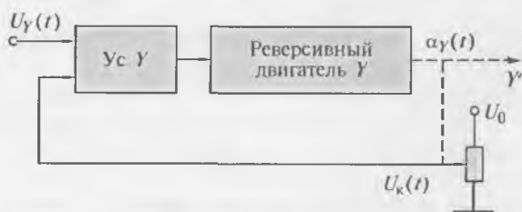
Рис. 5.3. Реализация отрицательной обратной связи
