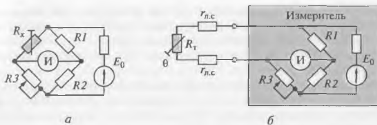
Рис. 8.3. Включение ТС в мостовую схему:
