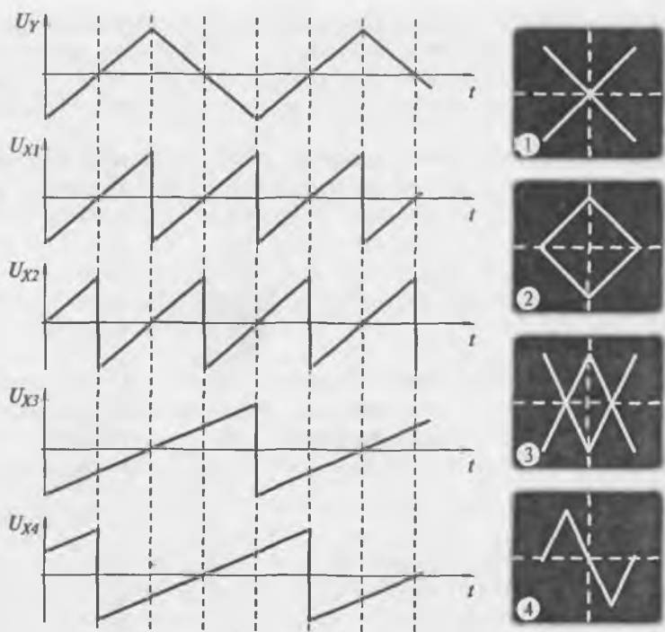
Рис. 4.7. Формирование изображения на экране
