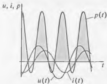
Рис. 2.7. Мощность — функция времени p(t)
