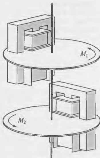
Рис. 3.19. Двухэлементный трехфазный счетчик
