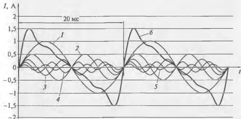
Рис. 2.16. Суммирование пяти гармоник
