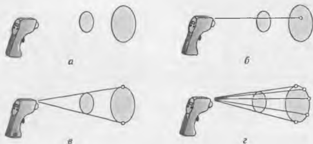
Рис. 8.17. Варианты организации лазерных указателей: а — без указателя; б — один луч; в — два луча; г — 8 лучей
