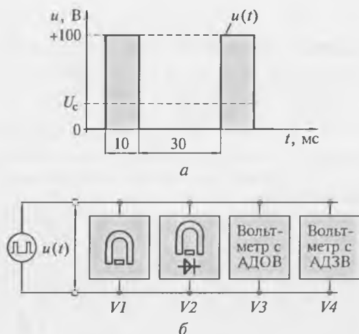
Рис. 3.30. Реакция и показания различных приборов: а — входной сигнал; б — схема включения приборов
