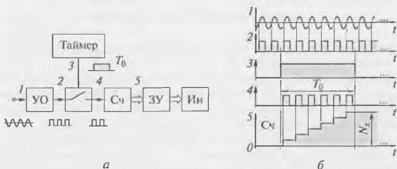
Рис. 6.3. Режим измерения частоты:
