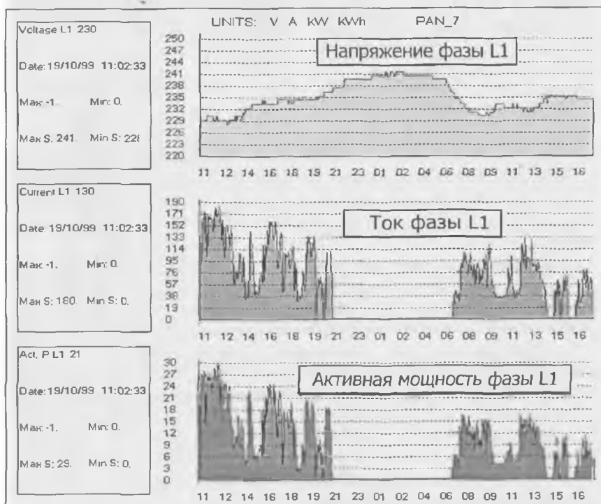
Рис. 7.20. Пример регистрации фазных напряжения, тока и мощности
