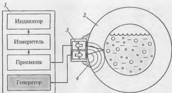
Рис. 8.36. Принцип действия УЗ-толщиномера:
