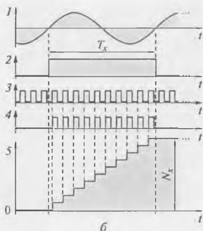
Рис. 6.7. Режим измерения периода (интервала времени): а — упрощенная структура ЦЧ; б — временные диаграммы
