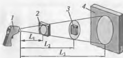
Рис. 8.15. Соотношение размеров объектов и мишени:
