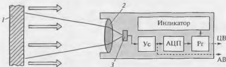
Рис. 8.12. Упрощенная структура ИК-термометра:
