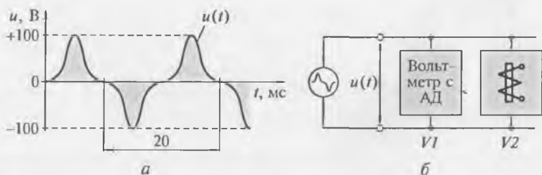
Рис. 3.29. Реакция и показания приборов:
