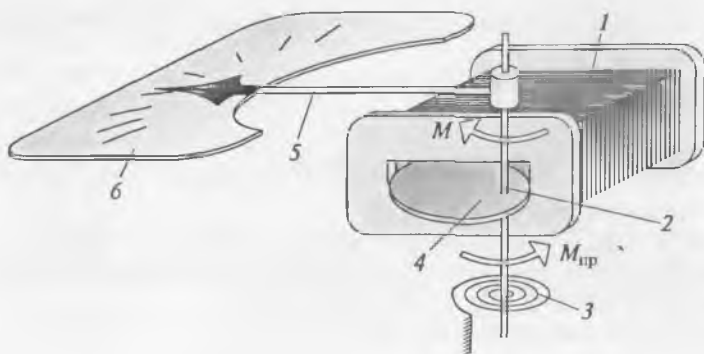
Рис. 3.7. Устройство электромагнитного механизма:
