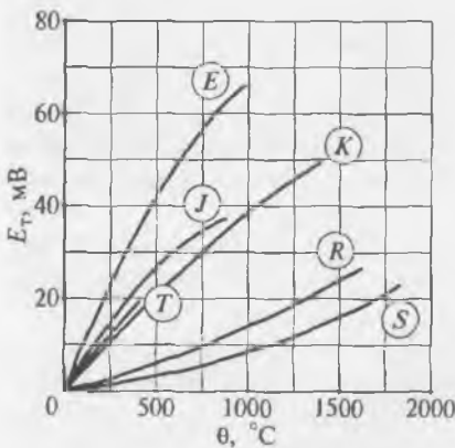
Рис. 8.6. Характеристики некоторых типов ТП:
