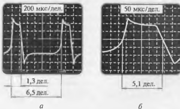
Рис. 4.28. Выбор коэффициента отклонения по оси X (скорости развертки):
