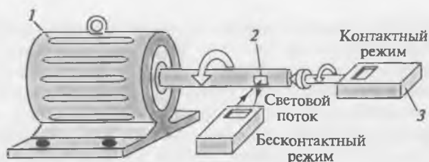
Рис. 8.34. Контактный и бесконтактный режимы измерения частоты вращения:
