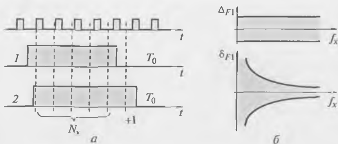
Рис. 6.4. Аддитивная погрешность в режиме измерения частоты: a — возникновение; б — абсолютная и относительная погрешности
