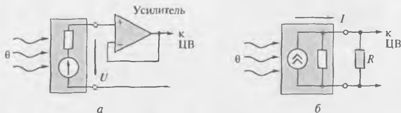
Рис. 8.7. Подключение интегральных полупроводниковых датчиков: а — напряжения; б — тока
