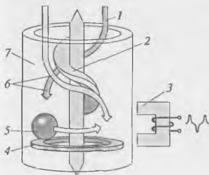
Рис. 8.31. Тахометрический шариковый расходомер:
