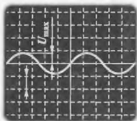
Рис. 4.29. Измерение амплитуды сигнала:
