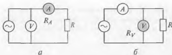
Рис. 1.13. Возникновение методической погрешности при различном подключении приборов:
