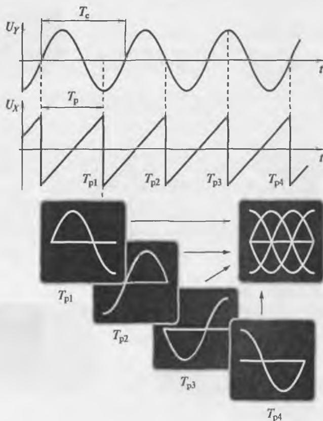
Рис. 4.6. Случай неравенства периодов сигнала и генератора развертки
