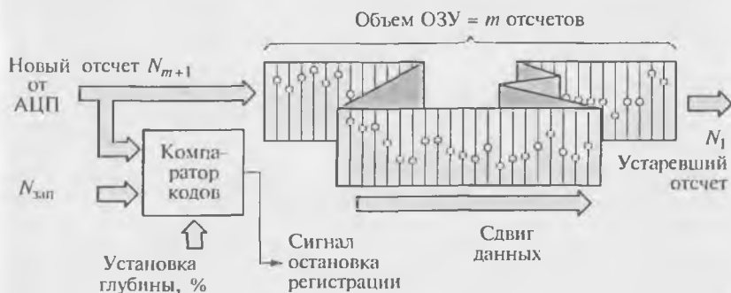
Рис. 7.7. Организация предзапуска
