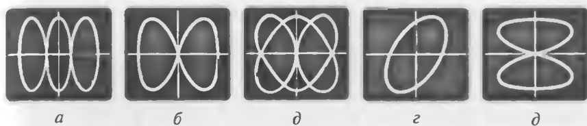
Рис. 4.14. Фигуры Лиссажу при соотношении частот f_y/f_x равном:
