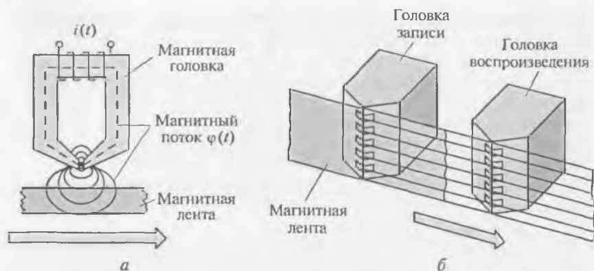
Рис. 5.11. Магнитная запись:
