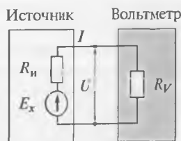
Рис. 1.14. Погрешность взаимодействия вольтметра и источника напряжения
