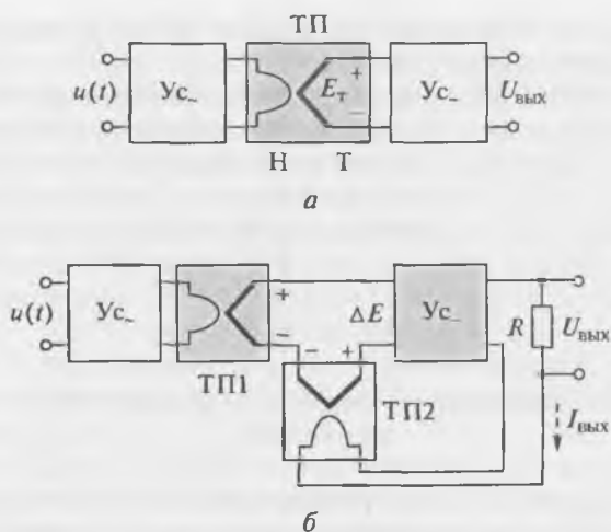
Рис. 3.27. Варианты (а и б) устройства термоэлектрического детектора
