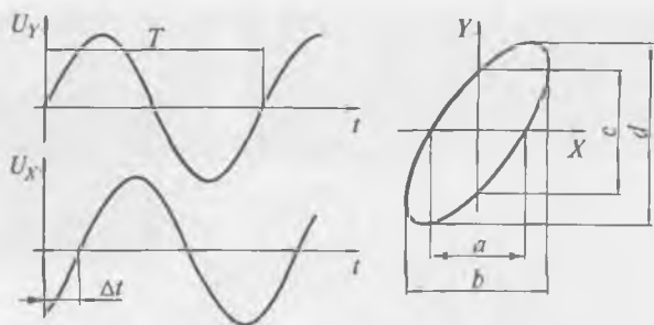
Рис. 4.10. Определение значения фазового сдвига
