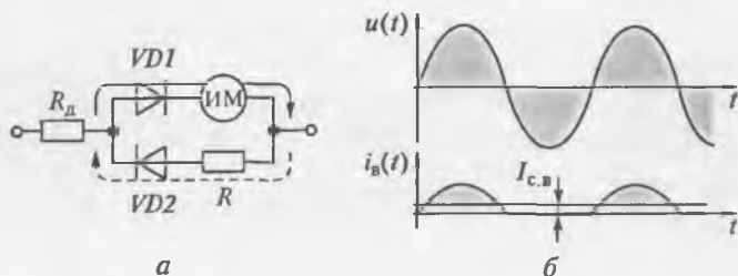
Рис. 3.5. Схема вольтметра с однополупериодным выпрямителем ( a ), временные диаграммы ( б )
