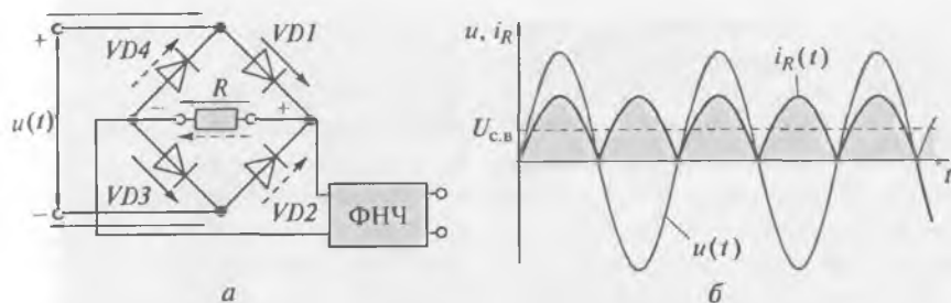
Рис. 3.25. Детектор среднего выпрямленного значения: а — схема; б — временная диаграмма
