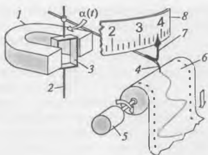
Рис. 5.1. Упрощенное устройство электромеханического СП:
