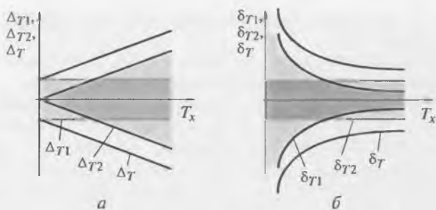
Рис. 6.9. Суммарные абсолютная (а) и относительная (б) погрешности
