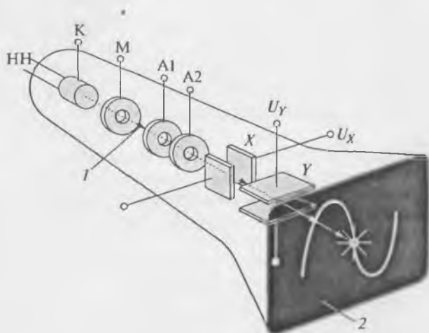
Рис. 4.2. Устройство ЭЛТ:
