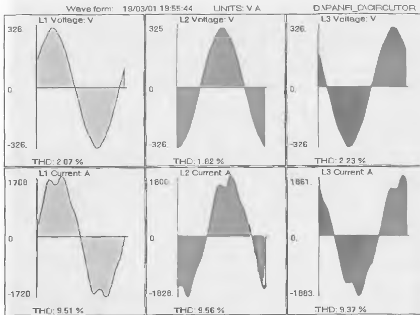
Рис. 7.22. Оценка несинусоидальности фазных напряжений и токов
