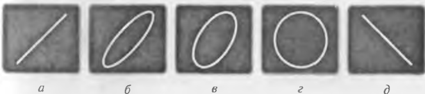
Рис. 4.11. Изображения на экране в методе эллипса для разных значений фазового сдвига:
