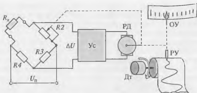
Рис. 5.4. Автоматический мост
