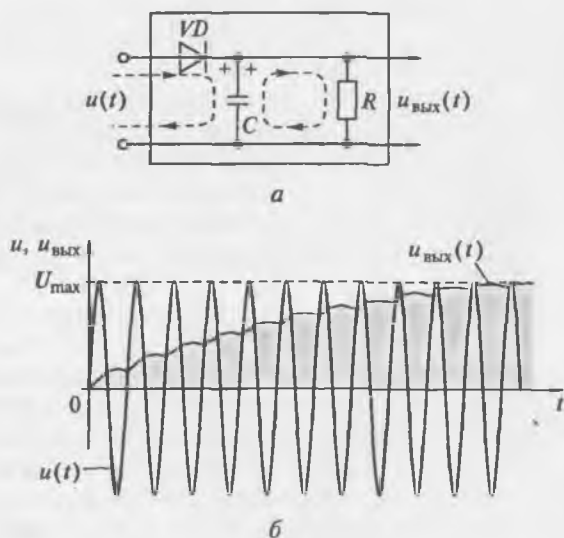
Рис. 3.21. Амплитудный детектор с открытым входом:
