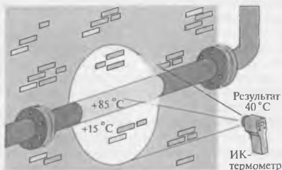
Рис. 8.14. Влияние температуры фона
