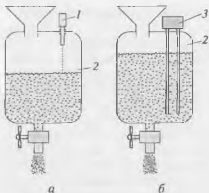
Рис. 8.33. Расходомеры на основе измерения уровня:
