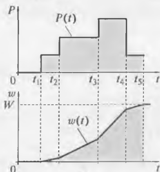
Рис. 2.9. Мощность и энергия:
