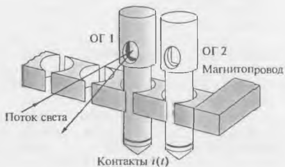
Рис. 5.9. Расположение гальванометров в магнитопроводе
