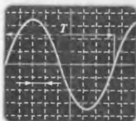
Рис. 4.30. Измерение периода сигнала:
