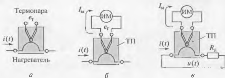
Рис. 3.6. Схемы термоэлектрических приборов:
