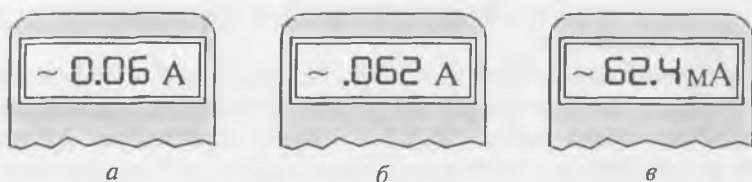
Рис. 6.15. Результаты измерений на трех диапазонах: a — 0...10 А; б — 0...1,0 А; в — 0...100 мА
