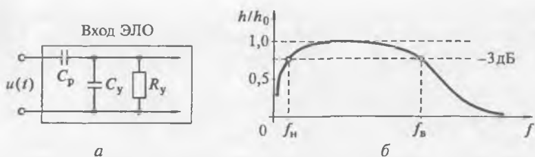
Рис. 4.26. Режим закрытого входа (а) и его АЧХ (б)
