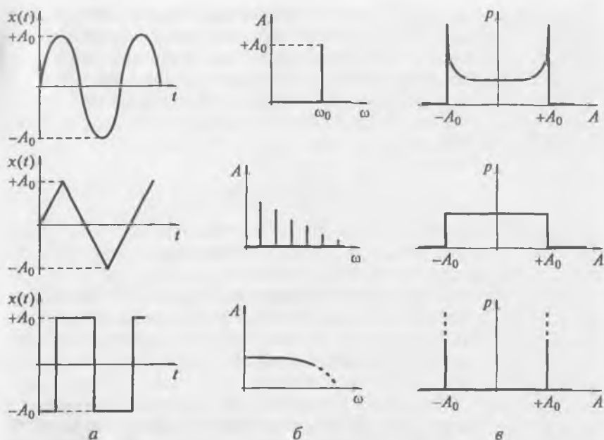
Рис. 7.9. Примеры представления сигналов в различных областях: a — во временной области; б — в частотной области; в — в амплитудной области
