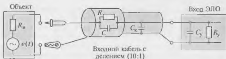
Рис. 4.22. Подключение входного кабеля с делением
