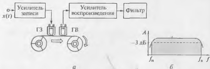
Рис. 5.12. Магнитограф с прямой записью:
