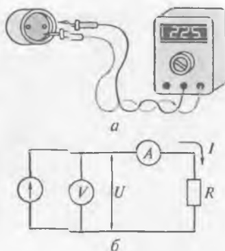
Рис. 1.2. Виды измерений: а — прямое, б — косвенное
