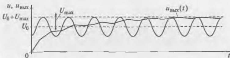
Рис. 3.22. Реакция АДОВ на сумму переменного и постоянного сигналов
