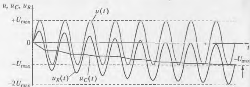
Рис. 3.24. Реакция амплитудного детектора с закрытым входом
