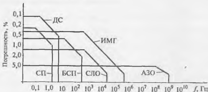
Рис. 5.14. Диаграмма «быстродействие — точность» для аналоговых регистраторов. По оси абсцисс в логарифмическом масштабе — полоса частот (верхняя граница). По оси ординат, также в логарифмическом масштабе, — относительная погрешность
