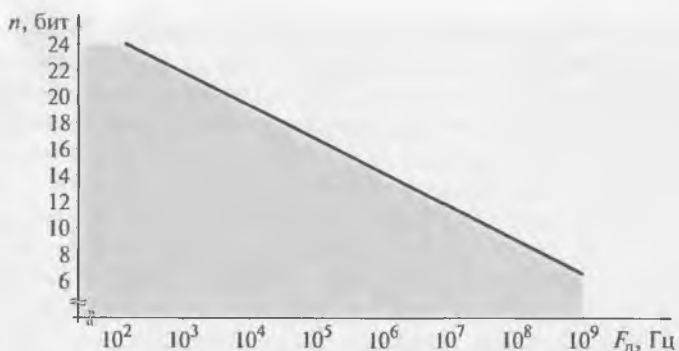
Рис. 6.2. Связь точности (разрядности АЦП) и быстродействия
