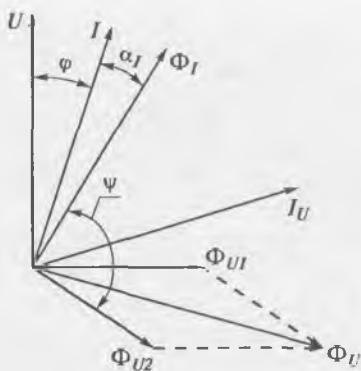
Рис. 3.17. Векторная диаграмма
