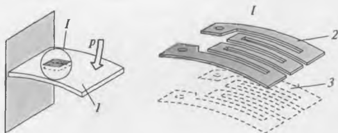
Рис. 8.26. Тензометрический эффект:
