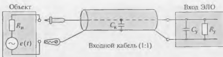
Рис. 4.21. Подключение входного кабеля без деления (1:1)
