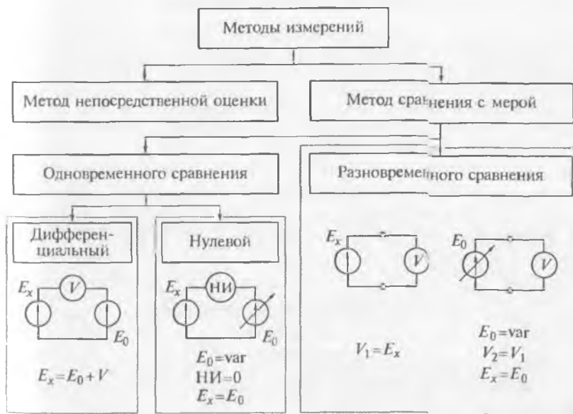
Рис. 1.3. Методы измерений
