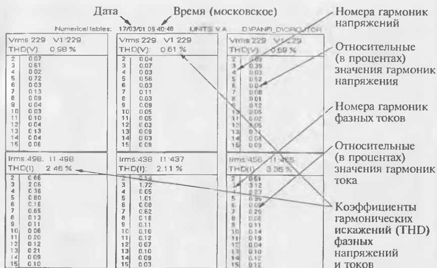
Рис. 7.24. Табличное представление спектрального состава напряжений и токов
