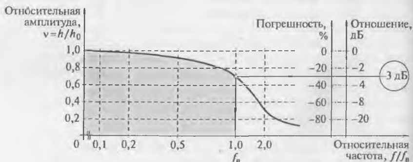
Рис. 4.18. Амплитудно-частотная характеристика канала Y
