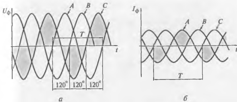
Рис. 2.11. Временные диаграммы:
