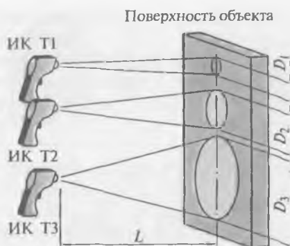
Рис. 8.13. Отношение расстояние/диаметр
