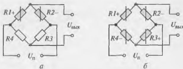
Рис. 8.27. Варианты мостовых схем:
