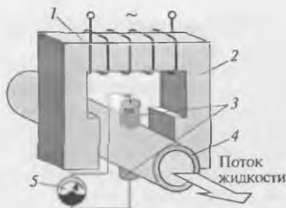
Рис. 8.32. Электромагнитный (индукционный) расходомер:
