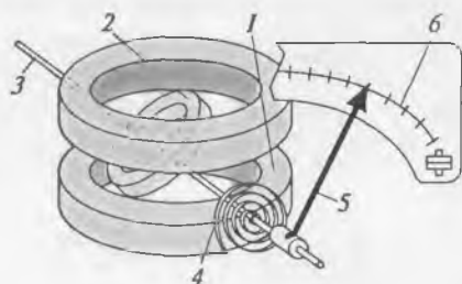
Рис. 3.9. Конструкция электродинамического измерительного механизма:
