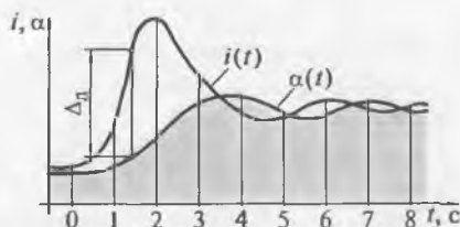
Рис. 1.17. Динамическая погрешность
