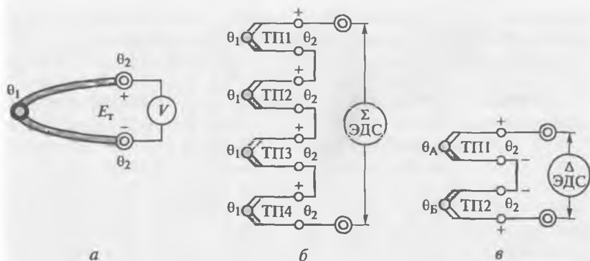
Рис. 8.5. Термоэлектрические преобразователи (термопары):
