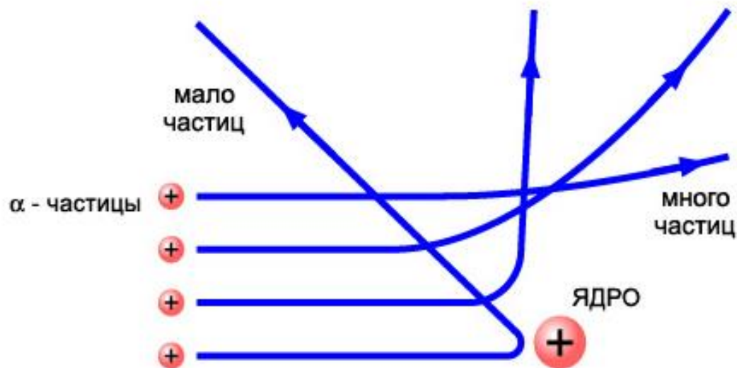
СХЕМА ВЗАИМОДЕЙСТВИЯ \alpha - ЧАСТИЦ С ЯДРОМ
