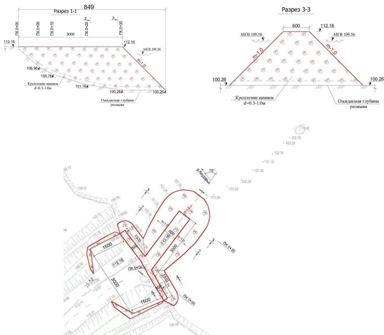
Рис.1. Конструкция шпору № 19 на реке Амударья.
