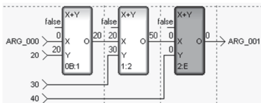
Рис. 2.32. Диаграмма FBD-программы с входными и выходными параметрами
