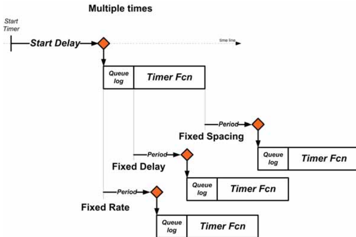
Рис. 3.19. Режимы многократного выполнения объекта таймера (временная диаграмма)
