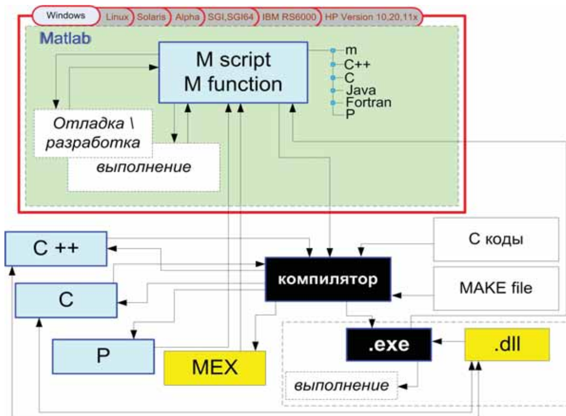
Рис. 3.9. Сводная схема алгоритмов программирования в среде Matlab
