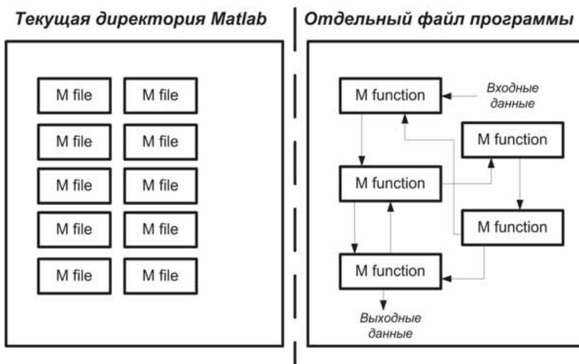
Рис. 3.10. Архитектура М-программы: совокупность М-файлов (слева), один М-файл программы (справа)
