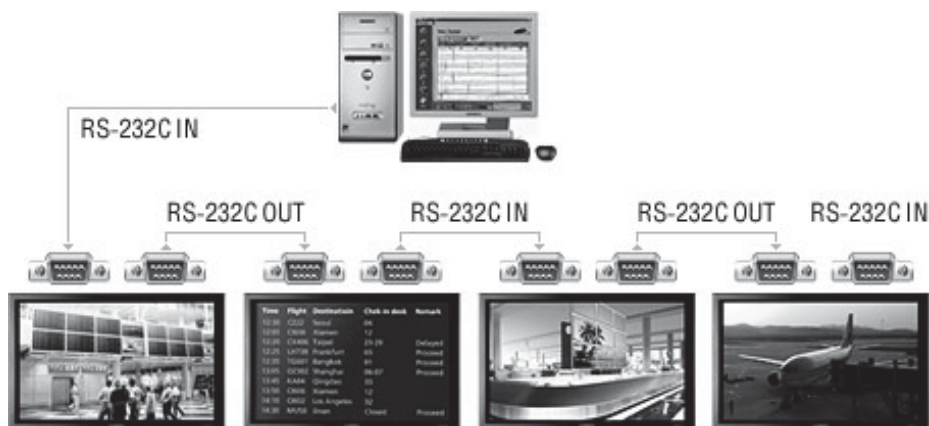
Рис. 1.2. Архитектура канала управления LCD-дисплеями
