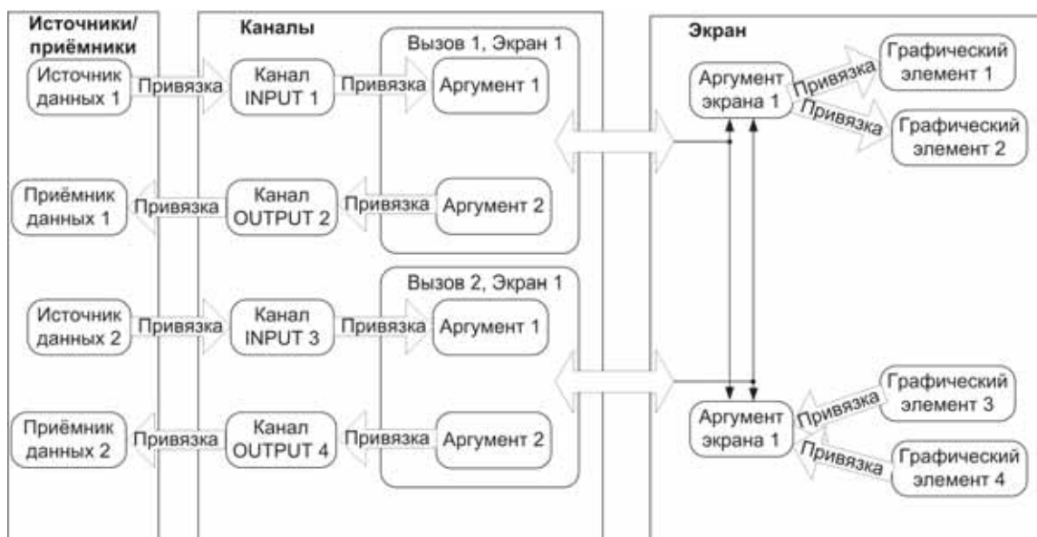
Рис. 2.2. Схема информационных связей, стандартный стиль разработки
