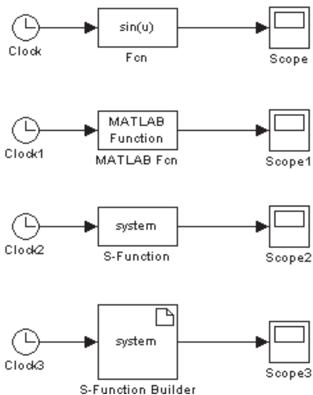
Рис. 3.25. Блоки User-Defined-Function Simulink
