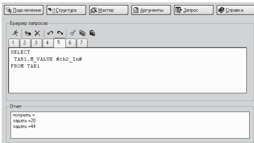
Рис. 2.14. Видеограмма окна мастера создания SQL-запросов в TRACE MODE. Данное окно снабжено типовыми инструментами создания/удаления запросов и работы с буфером обмена
