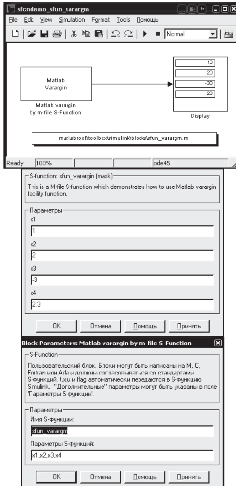
Рис. 3.26. Видеограмма модели, блок ввода параметров S-функция
