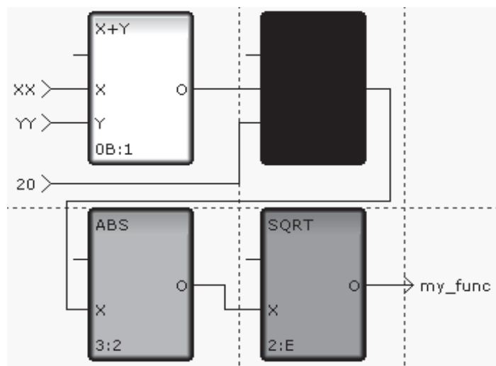
Рис. 2.29. Пример FBD программы
