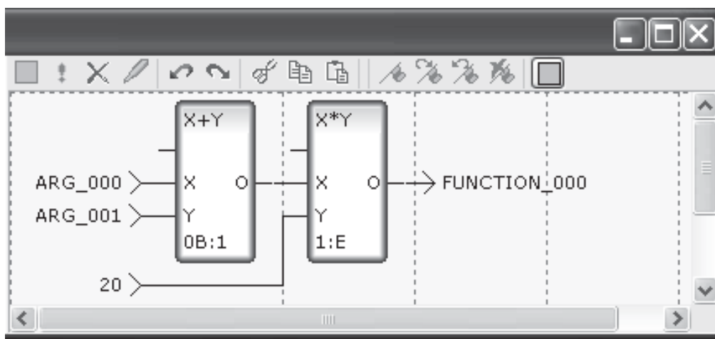
Рис. 2.25. Видеogramма рабочей области редактора FBD схем в TRACE MODE
