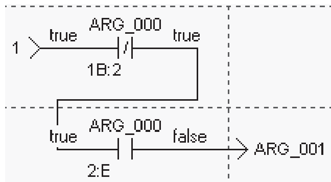
Рис. 2.33. Диаграмма LD-программы с входными и выходными параметрами
