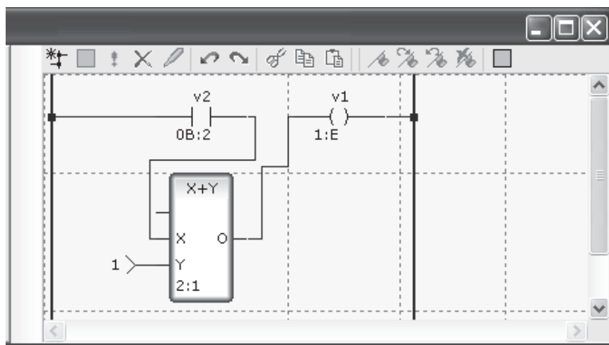
Рис. 2.26. Видеодиаграмма рабочей области редактора LD схем в TRACE MODE
