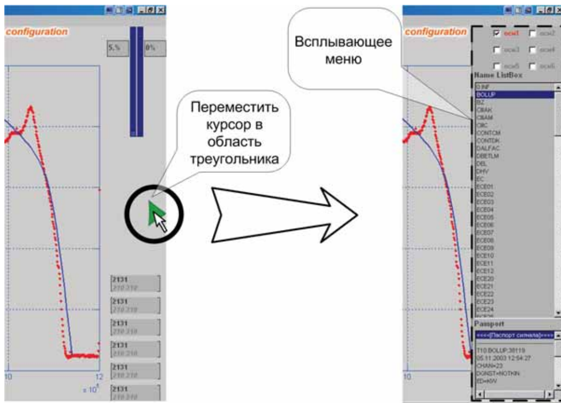
Рис. 3.14. Пример видеogramмы графической формы «Всплывающее меню»
