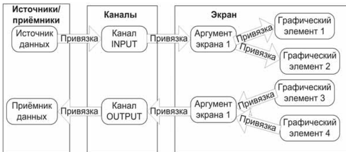
Рис. 2.1. Схема информационных связей, простой стиль разработки
