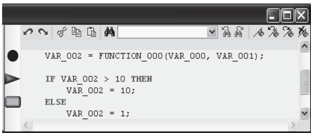
Рис. 2. 28. Видеограмма окна отладчика программ в TRACE MODE
