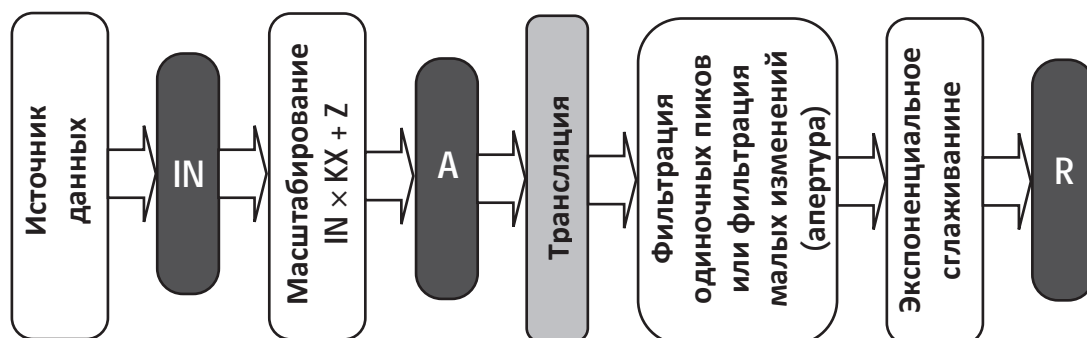
Рис. 2.3. Схема обработки информации в канале типа INPUT
