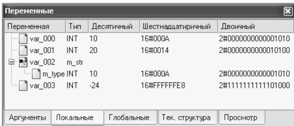
Рис. 2.31. Видеogramма окна редактора переменных в TRACE MODE
