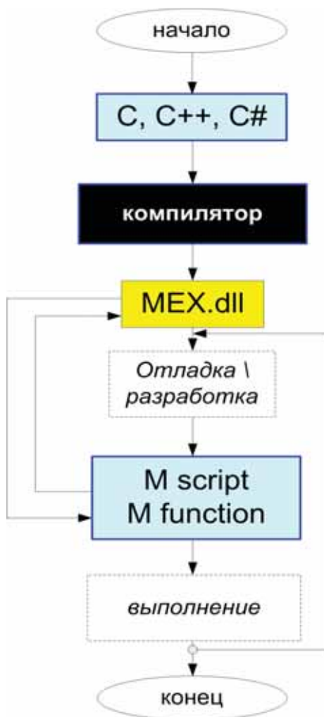
Рис. 3.8. Алгоритм интеграции С-код в М-код с последующим использованием
