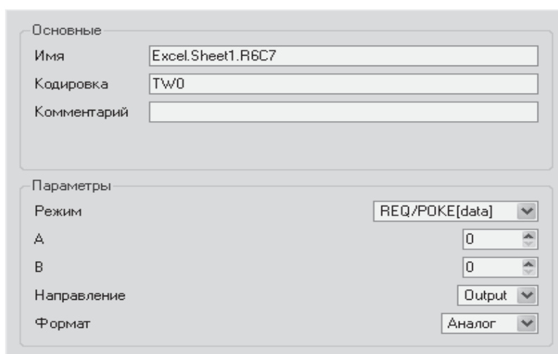
Рис. 2.16. Видеограмма окна настройки DDE обмена между MPB и Excel (режим request)
