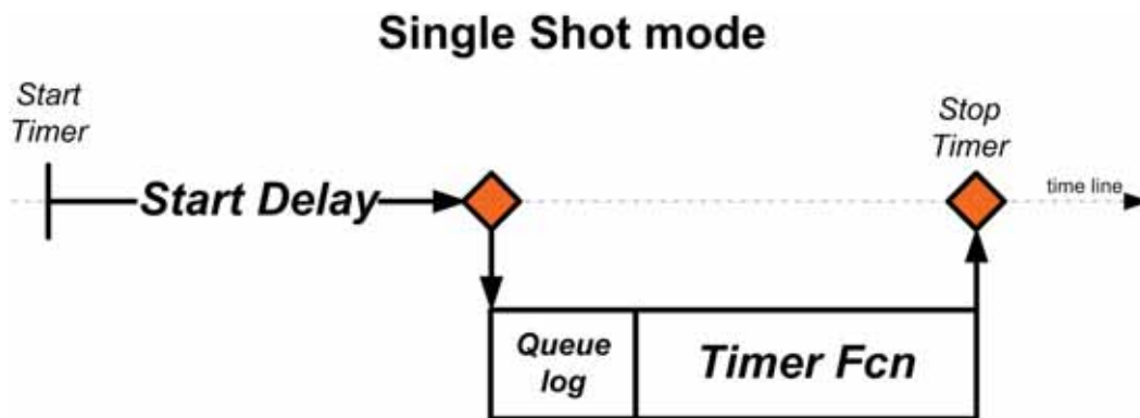
Рис. 3.18. Режим выполнения таймера singleShot (временная диаграмма)
