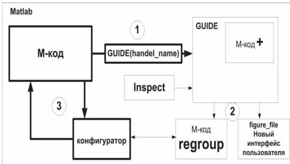
Рис. 3.16. Структурная схема технологии проектирования графических интерфейсов комбинированным способом
