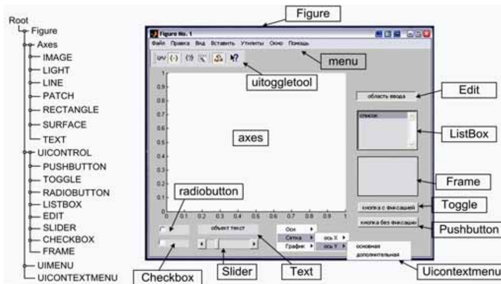
Рис. 3.12. Графические классы Matlab 6.5
