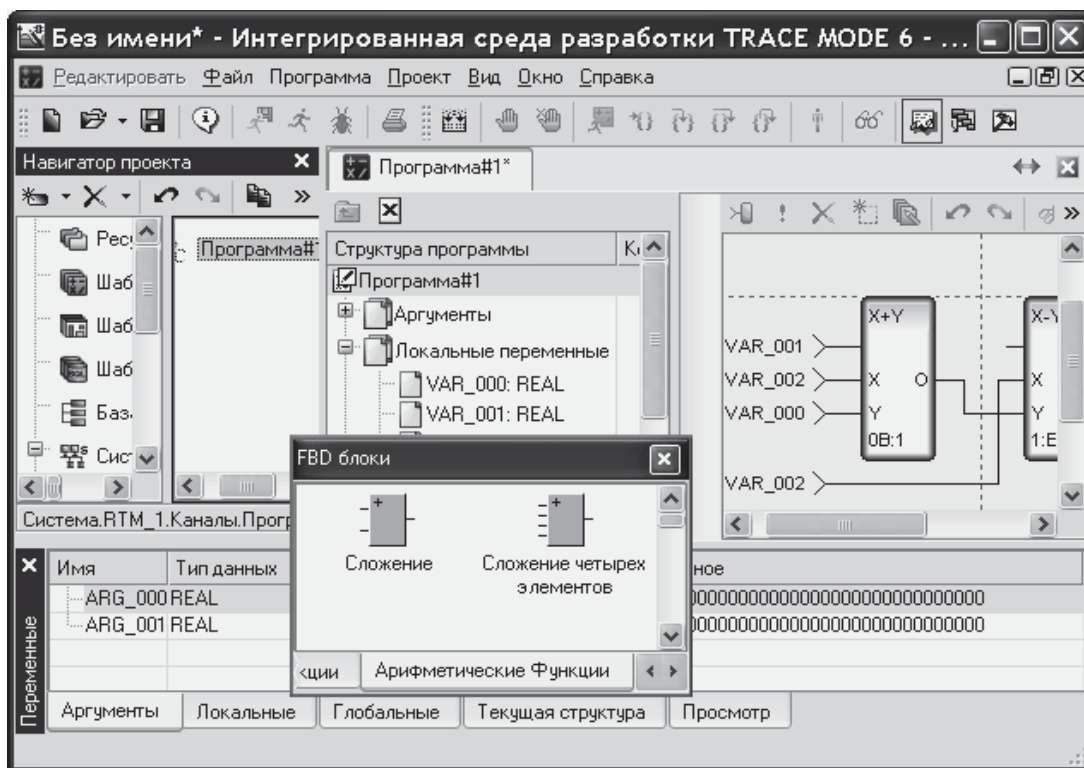
Рис. 2.23. Вид интегрированной среды разработки при редактировании программ
