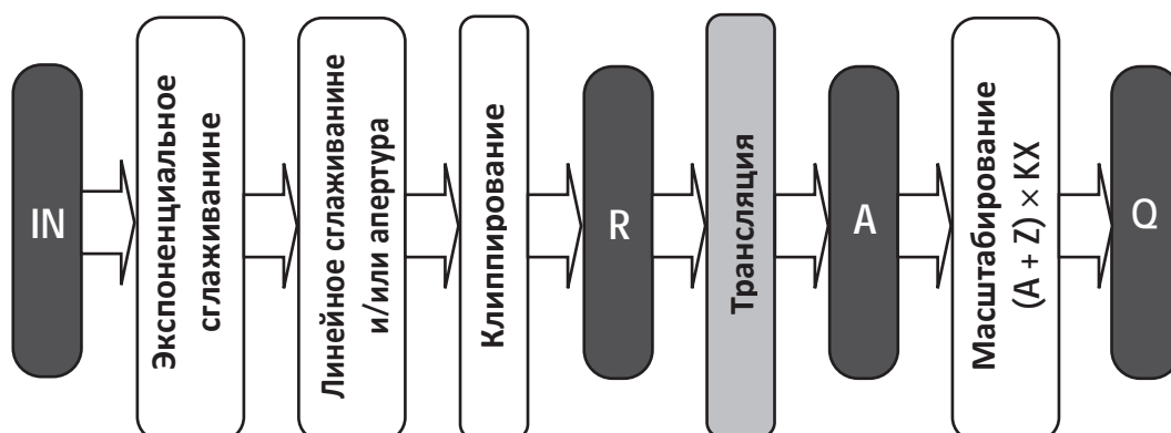
Рис. 2.4. Схема обработки информации в канале типа OUTPUT
