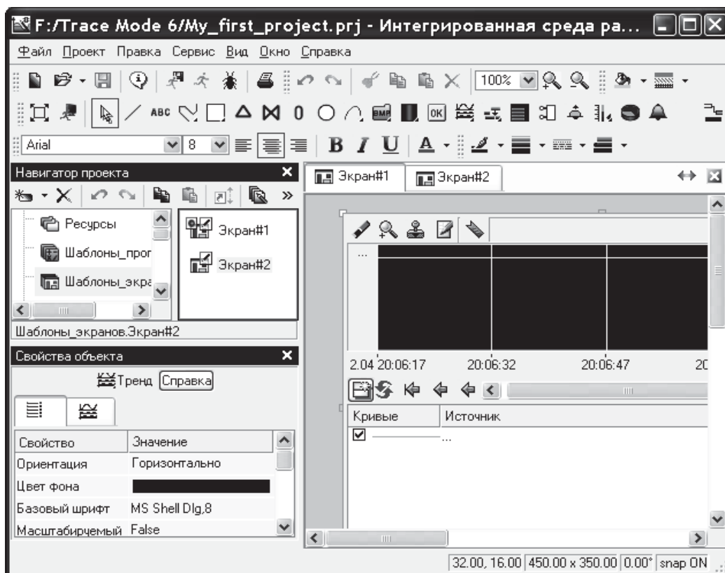
Рис. 2.11. Видеограма рабочего окна редактора представления данных
