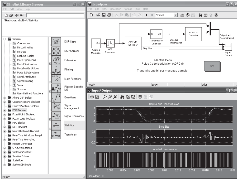
Рис. 3.21. Видеограмма графического пользовательского интерфейса визуального проектирования пакета Simulink
