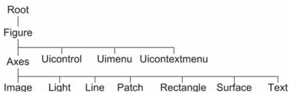
Рис. 3.11. Структура графических классов в Matlab
