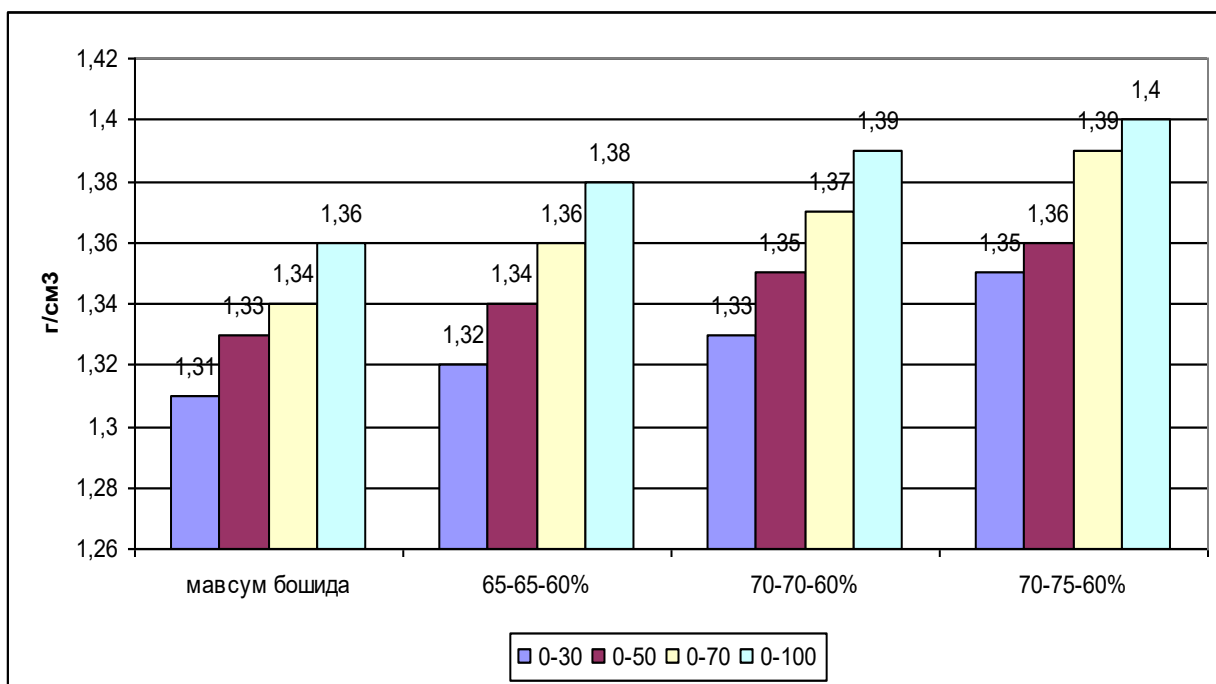
3.2.1.1- расм. Турли суғориш ва озиклантириш тартибларининг тупроқ ҳажм массасининг ўзгаришига таъсири, г/см 3 (2009 й)
