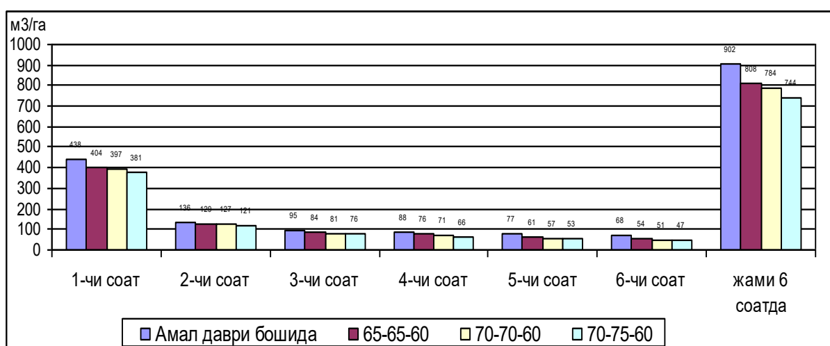
3.2.2.3- расм. Турли сув-озиқа меъёрлари ва суғориш тартибининг тупроқ сув тказувчанлигига таъсири, м 3 /га (2010 й)
