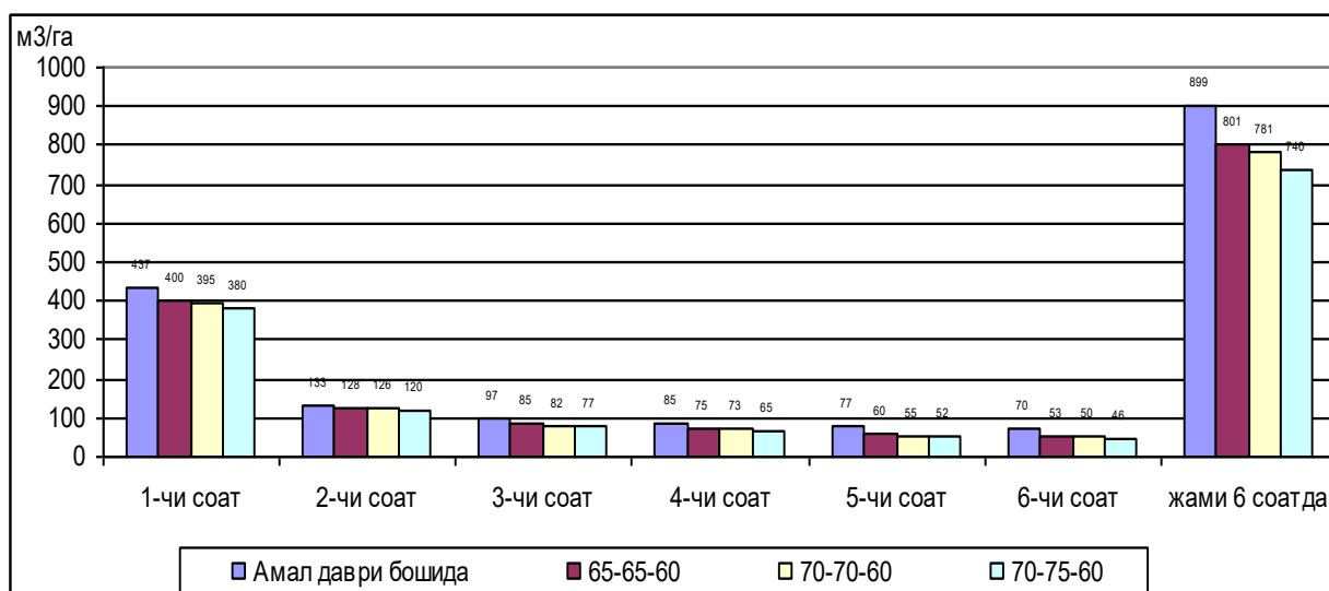
3.2.2.4- расм. Турли сув-озиқа меъёрлари ва суғориш тартибининг тупроқ сув ўтказувчанлигига таъсири, м 3 /га (2011 й)
