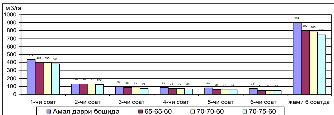
3.2.2.2- расм. Турли сув-озиқа меъёрлари ва суғориш тартибининг тупроқ сув ўтказувчанлигига таъсири, м 3 /га (2009 й)
