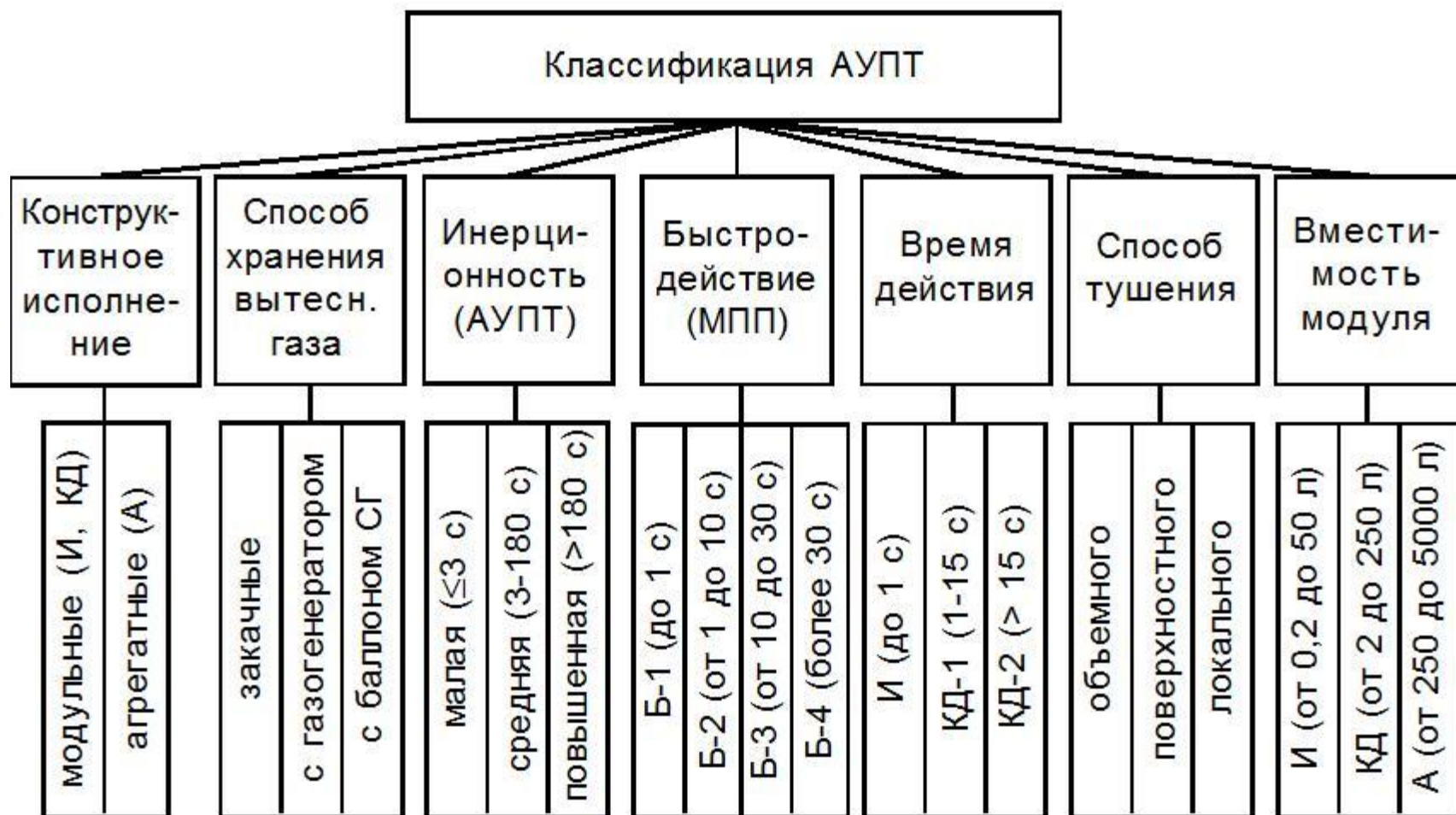
Рис. 2.5. Классификация автоматических установок порошкового пожаротушения по ГОСТ Р 51091-97
