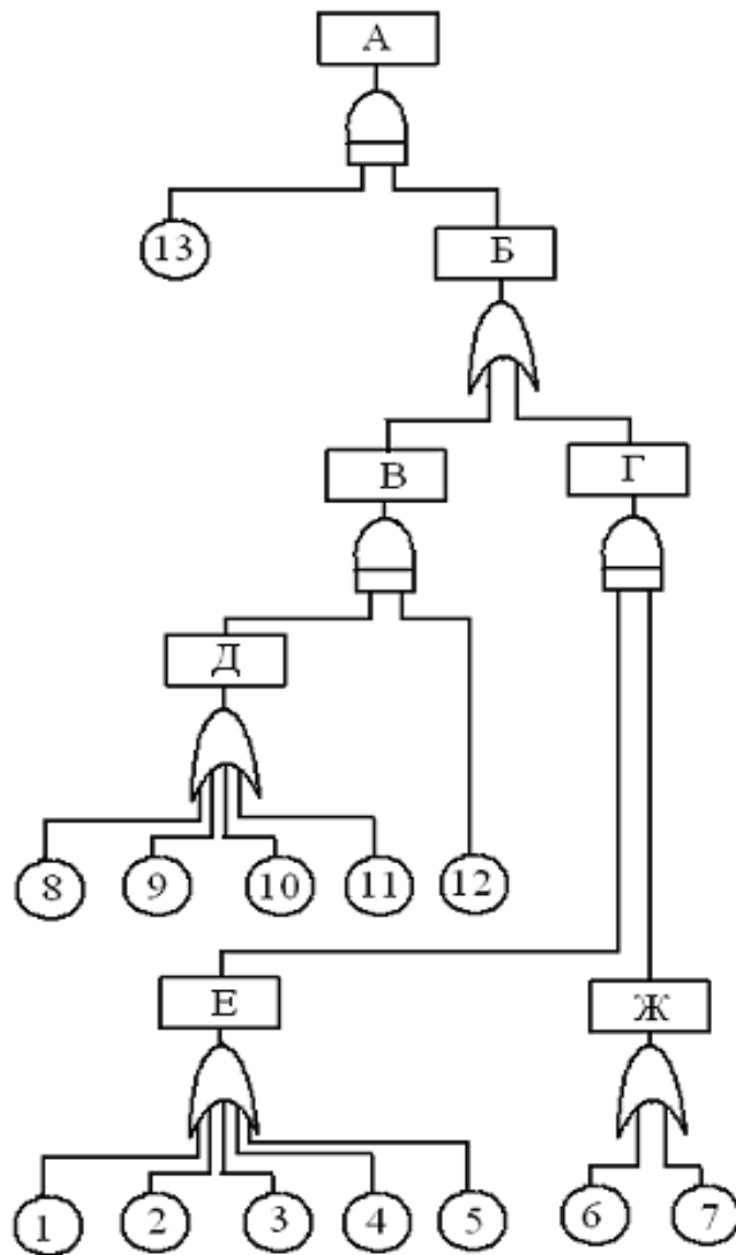
7-расм. Кимёвий реакторда портлаш содир бўлишини таҳлил қилишнинг "сабаблар ва хавфлар дарахти" (№1 химоя занжирى).
