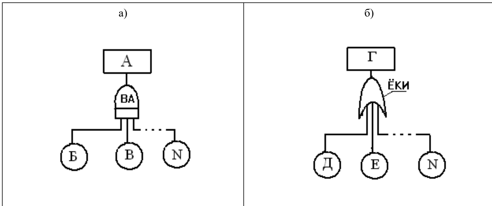
8-расм. Хавфсизликни таҳлил қилишда қўланиладиган «BA» ҳамда «ЁКИ» мантиқий амаллари («бузилишлар дарахти» усулида)
