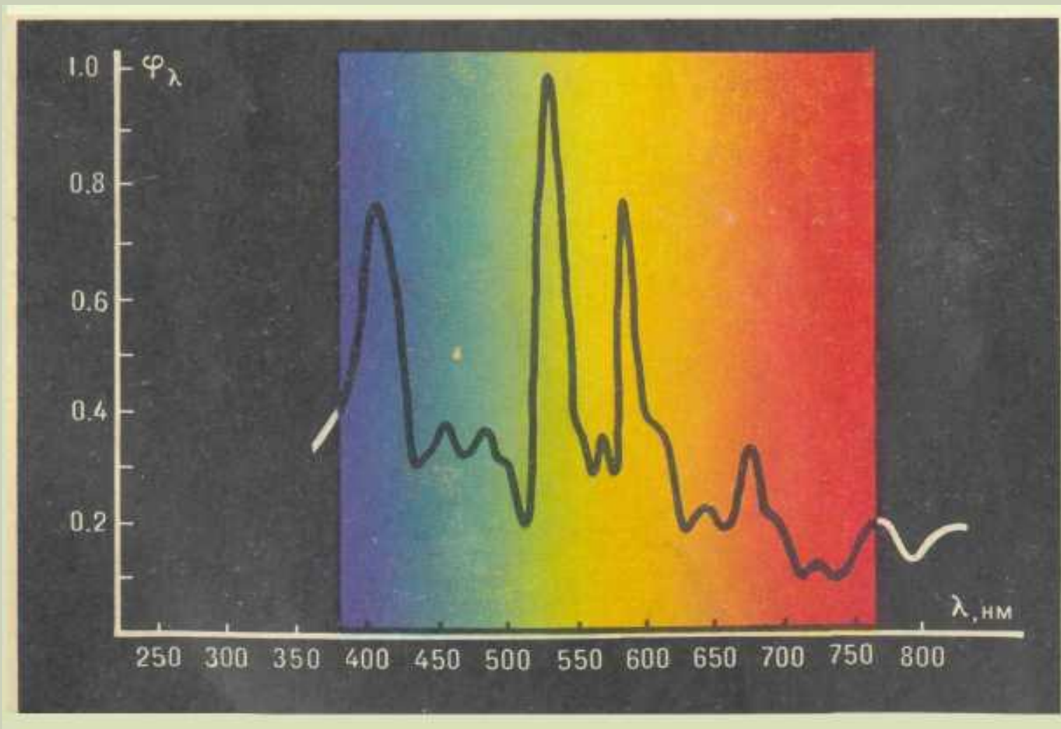
8.7.1-рaсм. ДРИ лампaсининг спектр зичлиги.
