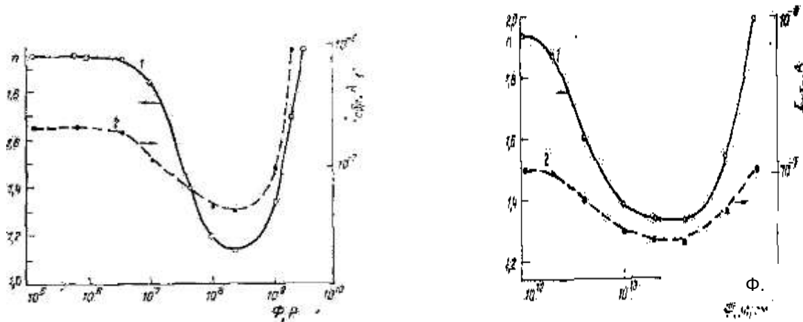
Рис.1. Дозовые зависимости фактора идеальности (1) и I_{обр} при U_{обр}=5 В (2) диода Шоттки Au-n- n^+ -GaP: а - облученные \gamma -квантами ^{60}\text{Co} ; б - облученные электронами с энергией 2 МэВ [5].
