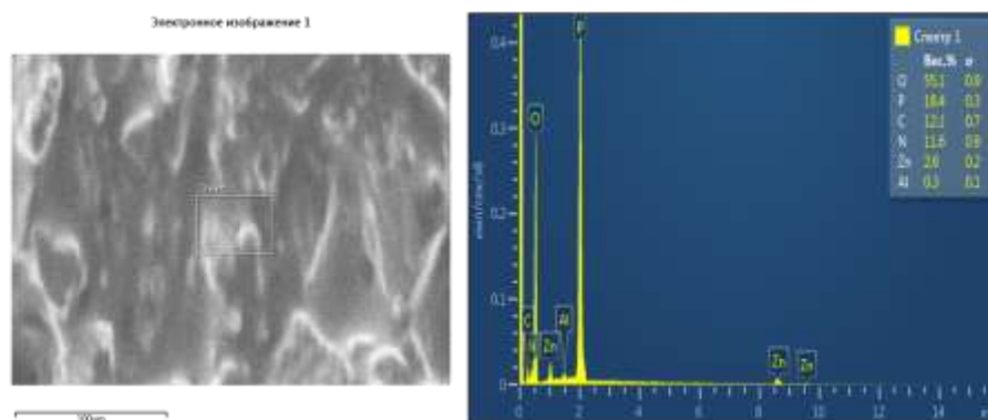
Рис. 1. Данные сканирующего электронного микроскопа и элементный анализ антипирена марки SA41.
