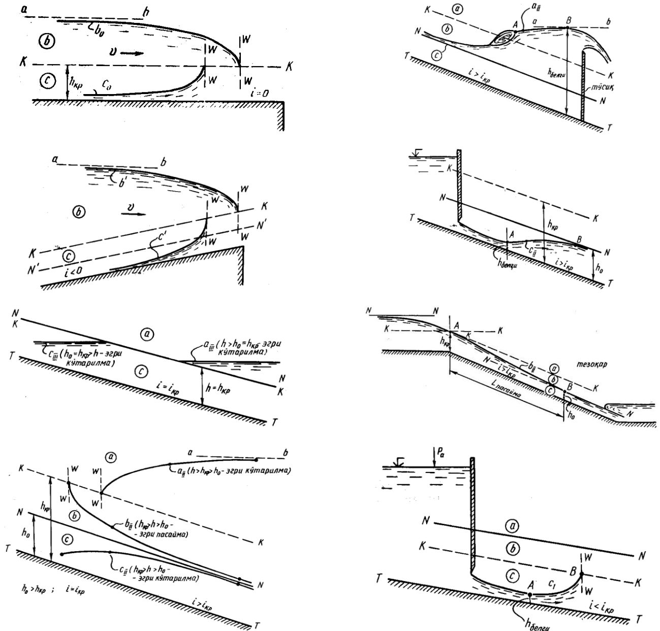
14.1-rasm - Ochiq o'zandagi suvning notekis harakatiga misollar.
