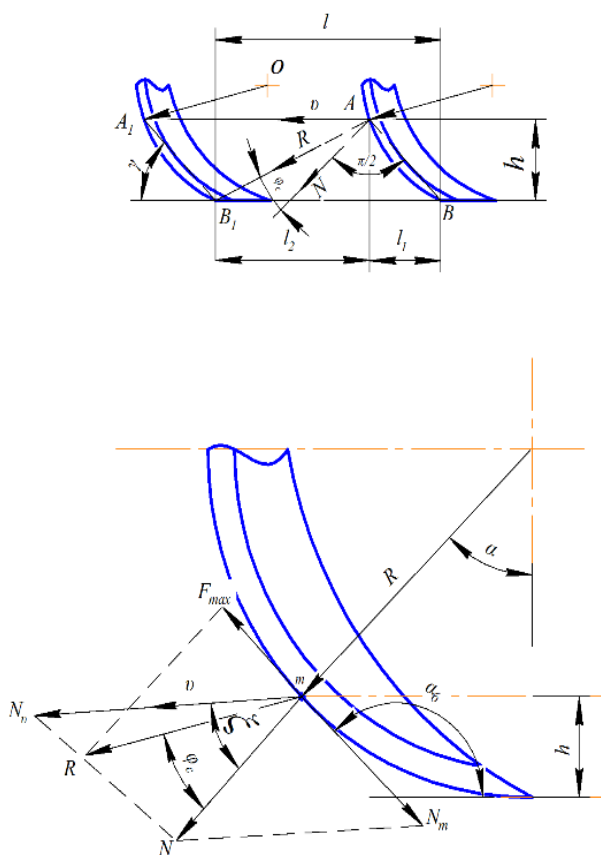
Рис. 6. Схема определения оптимального угла погружения дугообразного лезвия в почву
