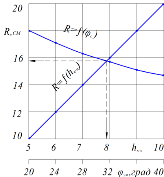
Рис. 6. График зависимости радиуса кривизны сектора ножа от глубины погружения в грунт и угла трения
