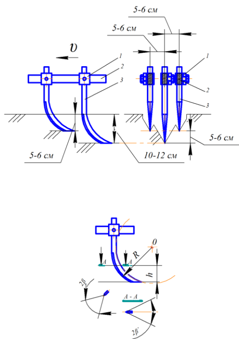
Рис. 3. Схема нового рабочего органа, размягчающего почву, в форме дугообразного ножа: 1 – замок; 2 – грядил; 3 – дугообразный нож
