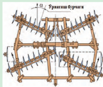
2-рasm. БДН-3 осма дискли тирма
