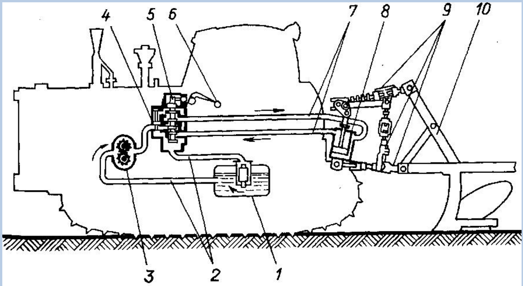
Алоҳида агрегатланган гидравлик тизимни схемаси 1-мой баки; 2 –мой ўтказиш қувирлари (паст босимли); 3 –мой насоси; 4 –таксимлагич; 5 –золотник; 6 –бошқариш ричаги; 7 –мой ўтказиш қувирлари (юқори босимли); 8 –куч цилиндри; 9 –осма механизми тортқилари.
