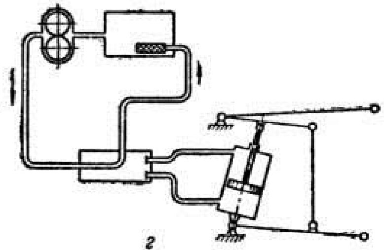
Алоҳида агрегатланган гидравлик тизимни ишлаш жараёни а-кўтариш; б-мажбурий тушириш; в-сузувчан ҳолат; г-нейтрал ҳолати.
