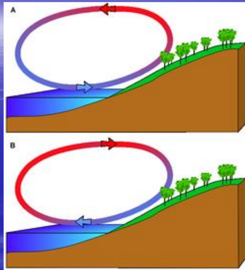
A: кундузги бриз B: тунги бриз.
