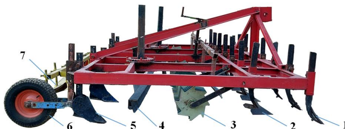
2-расм. Комбинациялашган агрегатнинг кўриниши
