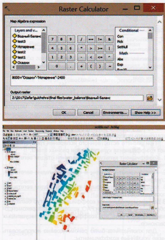
Рис.4. Расчет водного баланса
