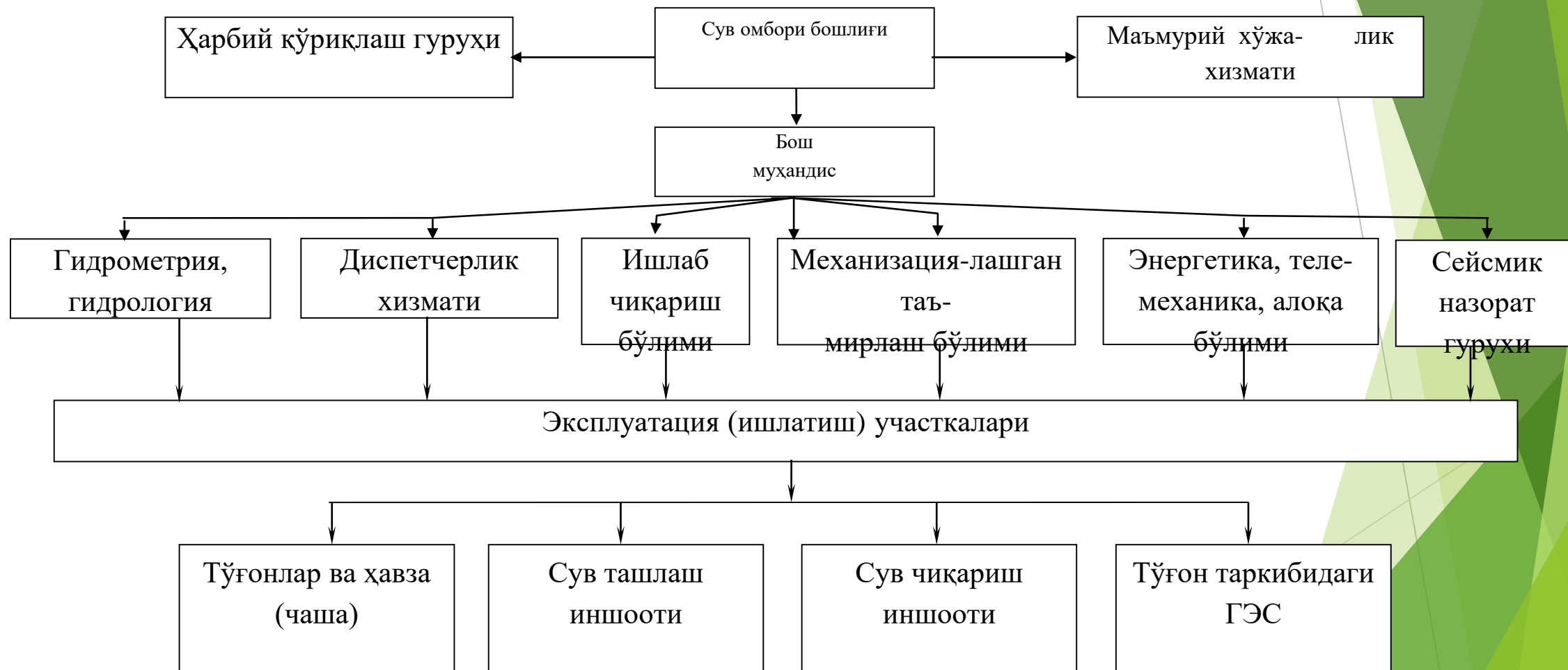
1.4-расм. Сув омборининг ташкилий схемаси.
