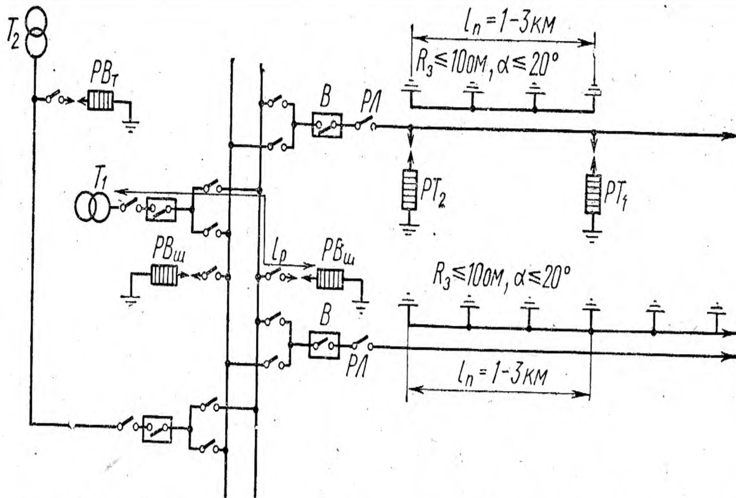
Рис. 14.6. Типовые схемы грозозащиты подстанций высокого напряжения
