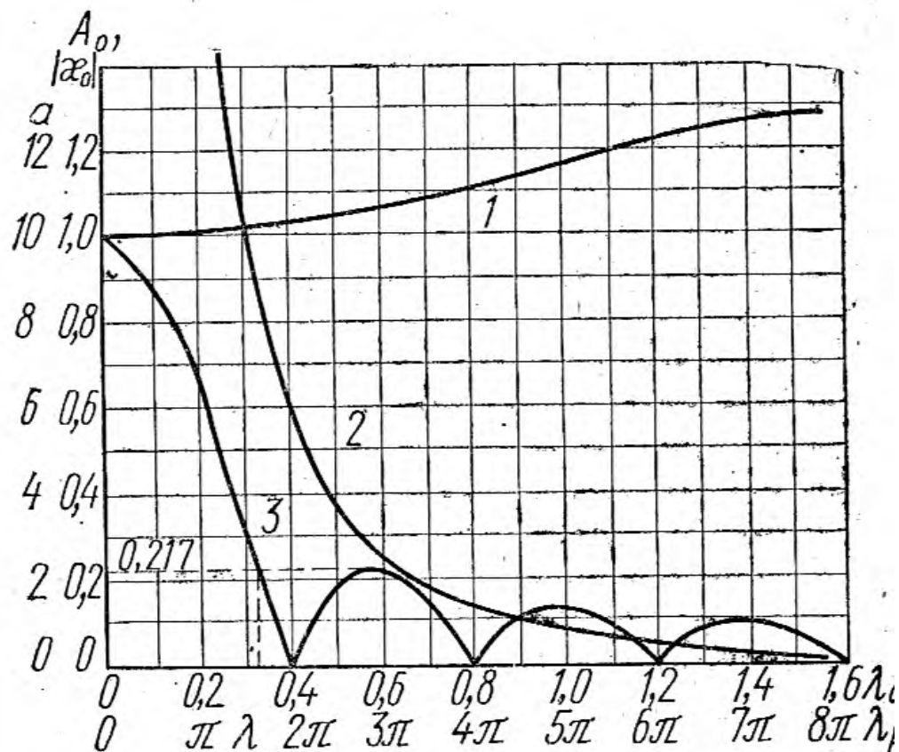
Рис. 14.10. Зависимость амплитуды A_0 основной гармонии колебаний (кривая 1) и соотношения емкостей a = C_T/C_1 (кривая 2) от волновой длины \lambda_0 = \beta_0 t_{12} , а также зависимости коэффициента сглаживания |\kappa_0| (кривая 3) от \lambda_p = \beta_0 \tau_p
