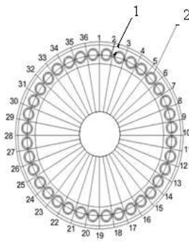
2-расм. Статор
