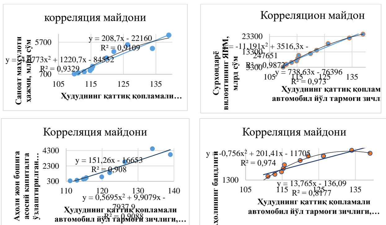
1-расм. Йўл тармоғи зичлигининг кўрсаткичларга боғлиқлик графиги.
