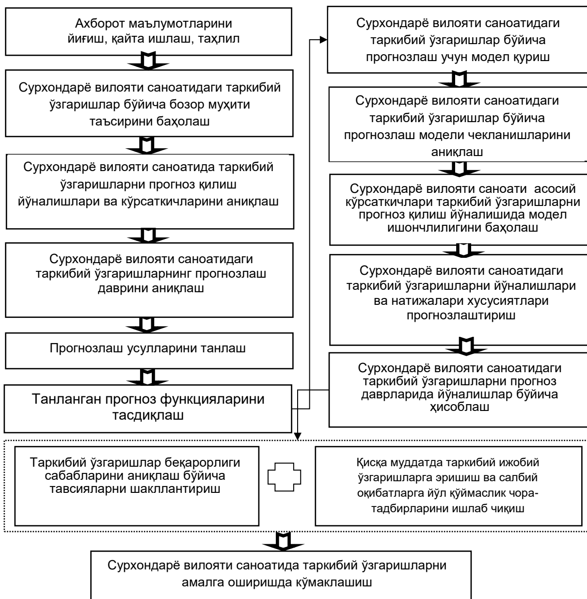
1-расм. Сурхондарё вилояти саноатида таркибий ўзгаришларни прогноз модели қуриш йўли билан моделлаштириш кетма-кетлиги 1
