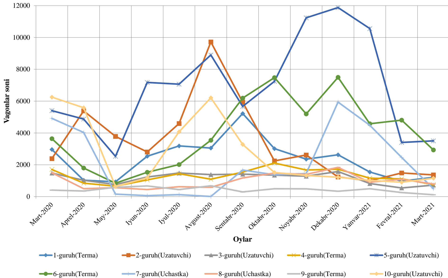
2-rasm. "Ch" stansiyasi poyezd tuzuvchi yo'nalishlar vagon oqimlari nomutonosibligi
