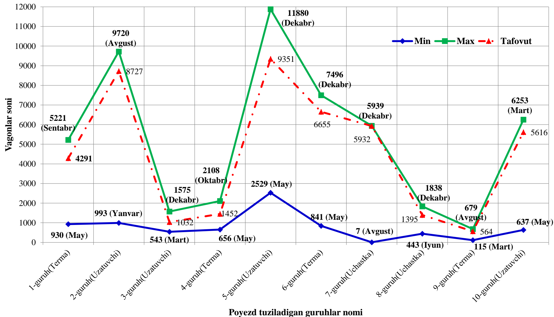
3-rasm. "Ch" stansiyasi poyezd tuzuvchi yo'nalishlar vagon oqimlarining o'rtacha oylik tofovuti
