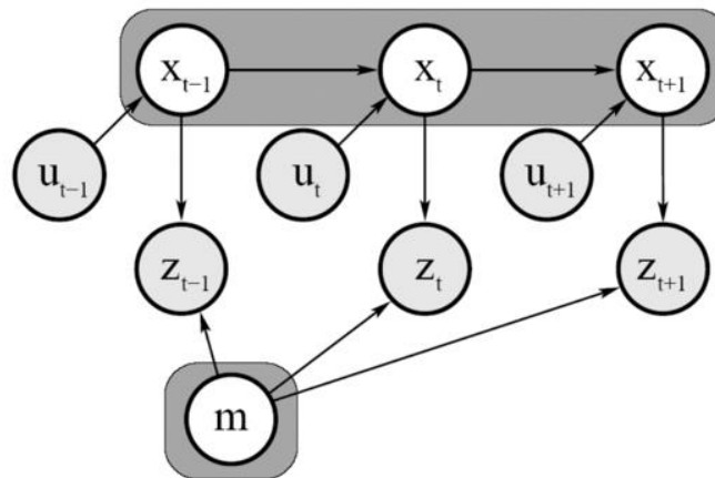
Рис. 6. Графическая модель SLAM подхода [7].
