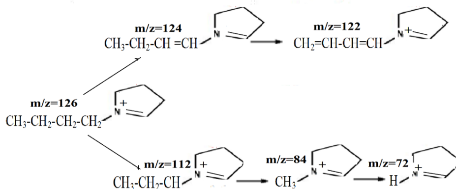
Рисунок 3.- Гетерогенные реакции диссоциации при адсорбции молекул \alpha -PVP гетероатомом азота
