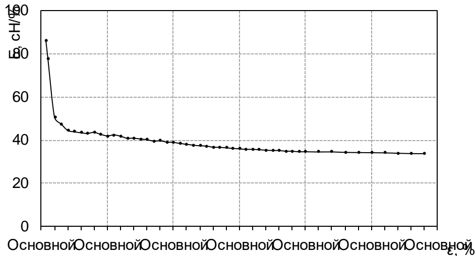
Рис.2. Зависимости E(\epsilon) полученные для хлопковой пряжи с линейной плотностью 20 текс
