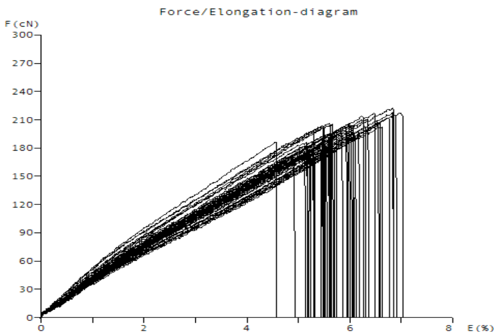
Рис.1. Экспериментальные зависимости F(s) полученные для хлопковой пряжи с линейной плотностью 20 текс
