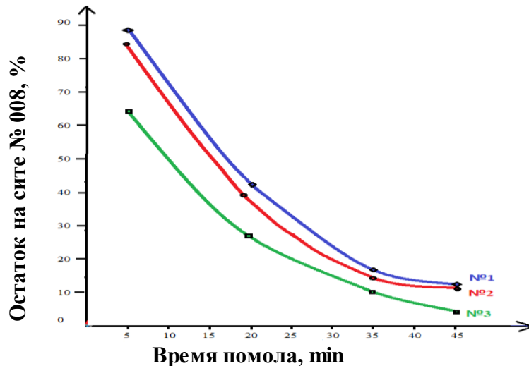
Рисунок 2. Тонкость помола сырьевых смесей с применением диабаз-порфиринов месторождения «Чимкурган-Писталитау»
