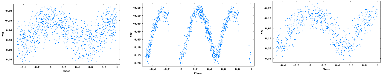
Рис. 1 Фазовые кривые блеска некоторых переменных звезд, обнаруженных в области скопления NGC 7419.
