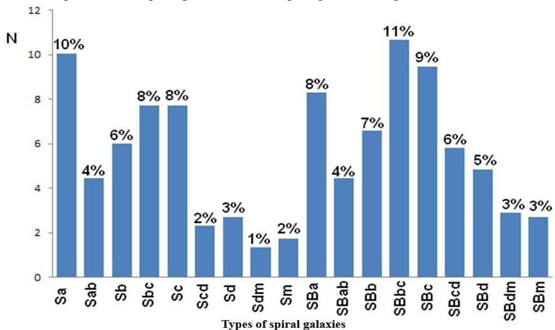
Рис. 1. Гистограмма распределения лопсайдных спиральных галактик по закрученности рукавов.
