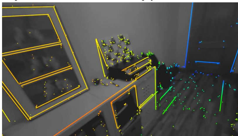
Рис. 3. Создание геометрической карты из точек или плоскостей в дополненной реальности.
