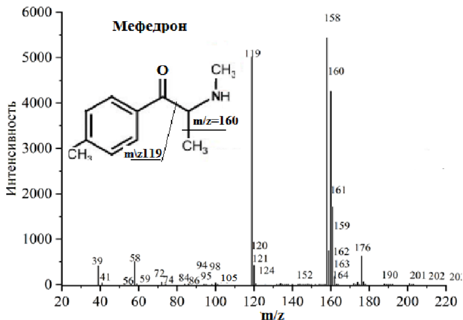
Рисунок 2.- Масс-спектр ТИ Мефедрона, ток накала ячейки I_a=100\text{mA} , T_e=950\text{K}
