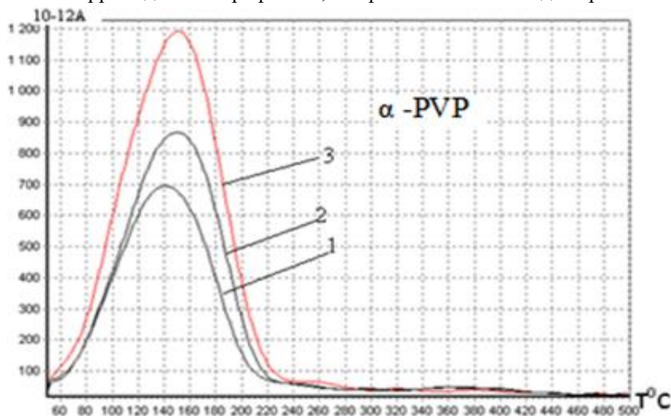
Рисунок 4. - ТДИ спектры катиона \alpha -PVP при количествах вещества: 1-100 ng, 2-150 ng, 3-250 ng
