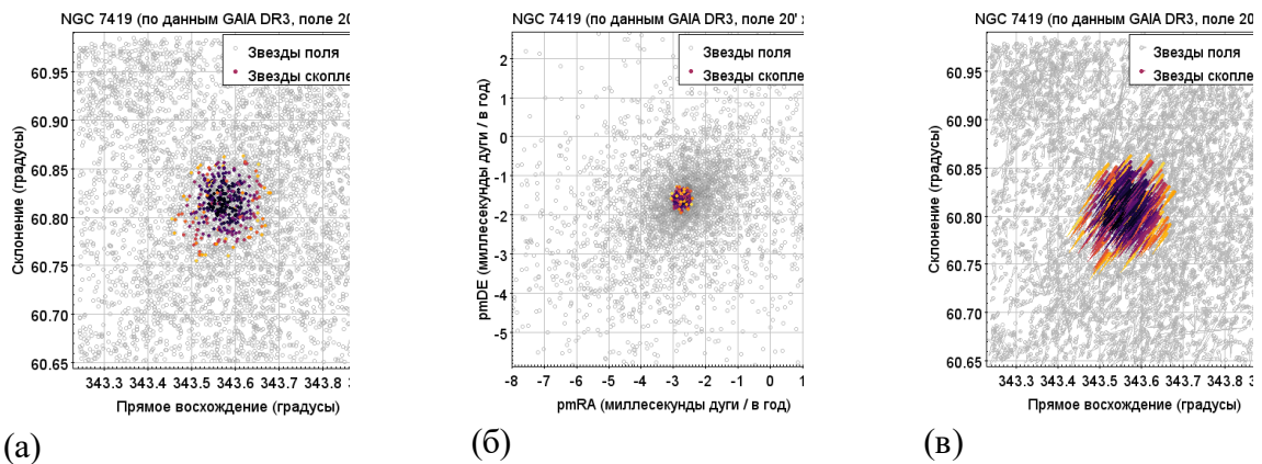
Рис. 1. а) Поле в окрестностях NGC 7419 с выделенными вероятными звездами скопления.; б) Диаграмма собственных движений звезд поля (серым) и вероятных звезд скопления области NGC 7419 (цветным); в) Векторы движения звезд поля (серым) – хаотично, и вероятных звезд скопления (цветным) – согласованно.
