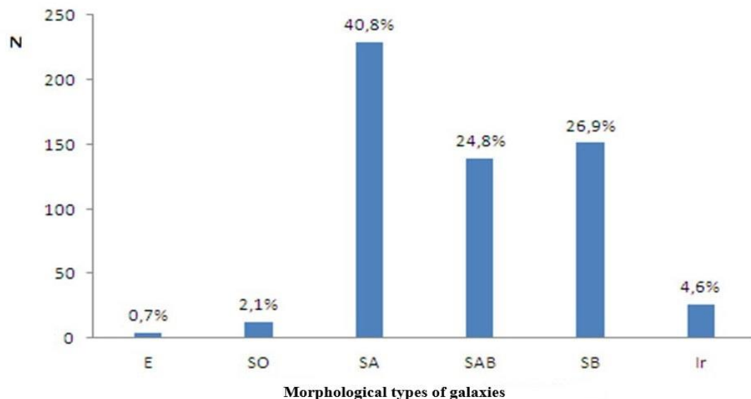
Рис.2. Гистограмма распределения лопсайдности по морфологическим типам галактик.
