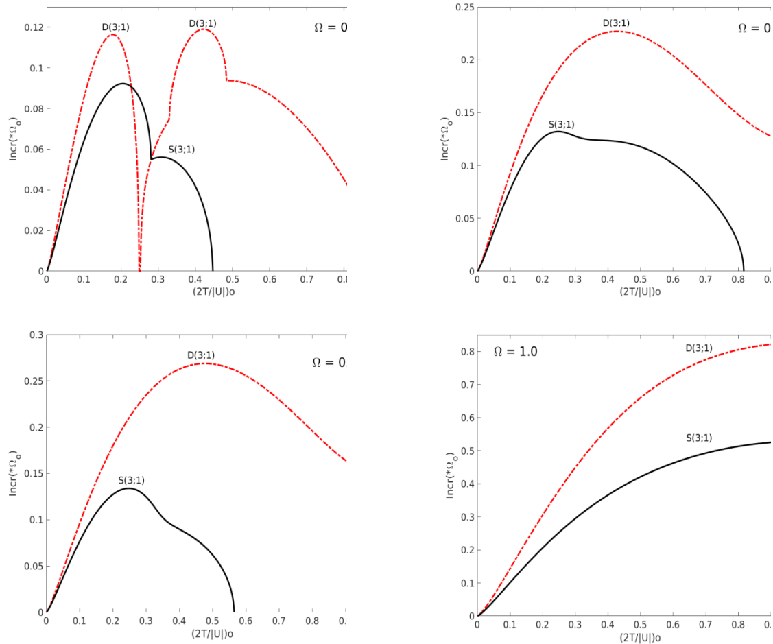
Рис. 3. Сравнение инкрементов неустойчивостей лопсайдалной моды (3;1) на фоне нелинейно нестационарных дисковой [10] и сферической [9] моделей для различных значений параметра вращения \Omega .
