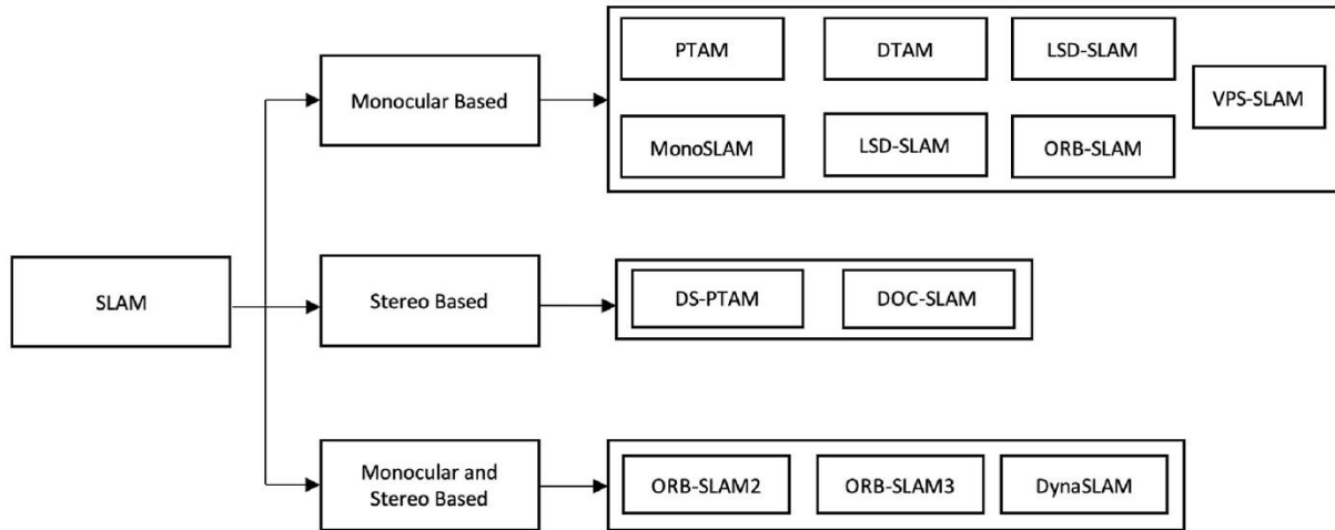
Рис. 4. Классификация алгоритмов Visual SLAM.
