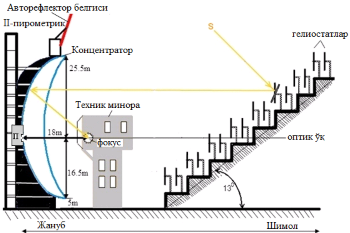
1.5-расм. Катта қуёш печининг асосий компонентлари – гелиостат майдони, минора, бойитиш фабрикаси.
