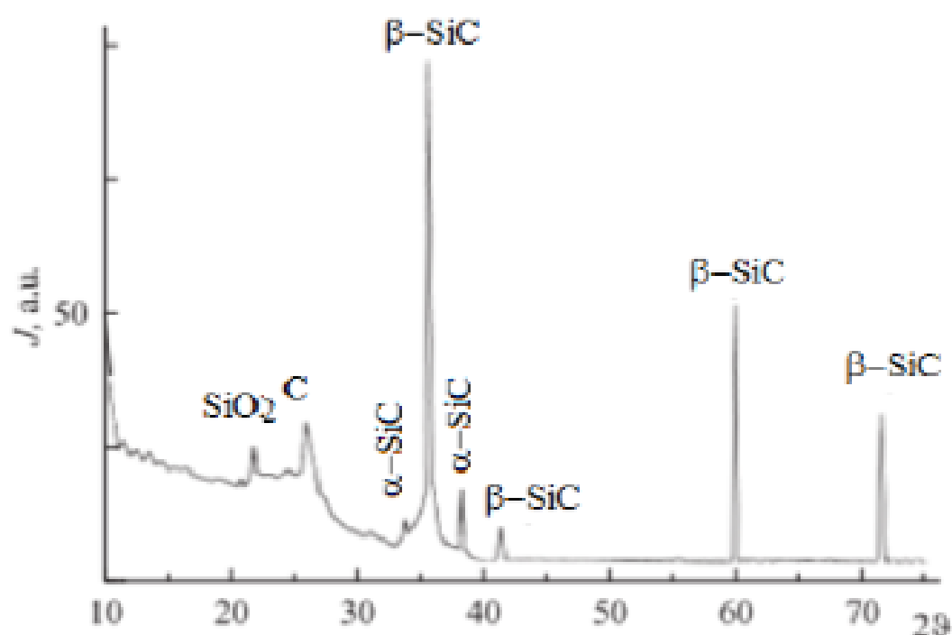
Рис.1. Рентгенограмма золы рисовой шелухи после термообработки на графитовом тигле при 1650 °С
