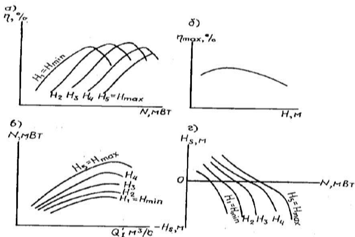
Rasm 2.9. H=f(N) , \eta_{max}=f(H) , N=f(Q'_1) va H_s=f(N)
