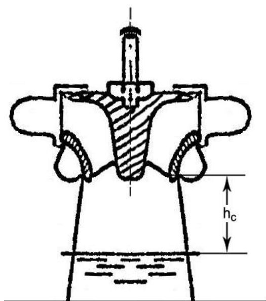
Rasm 1.2. Nasoslarning geometrik so'rish balandligi. a-gorizonta; b-tik o'qiy; c-markazdan qochma tik; d-porshenli.
