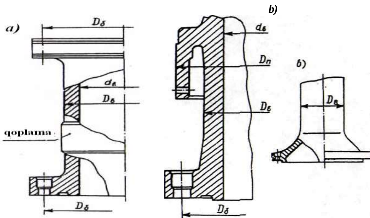
Rasm 2.36. Valni po'lat qoplamasi sxemasi
