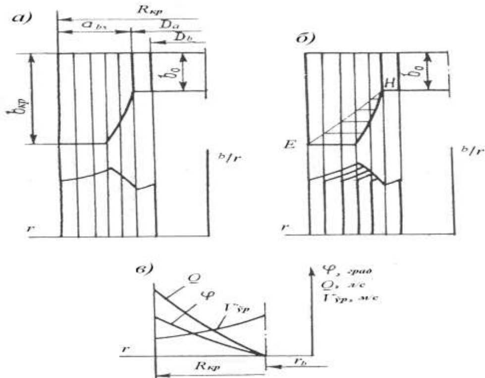
Rasm 2.13. Betonli spiral kamerani grafoanalitik usuliga ko'ra hisoblash
