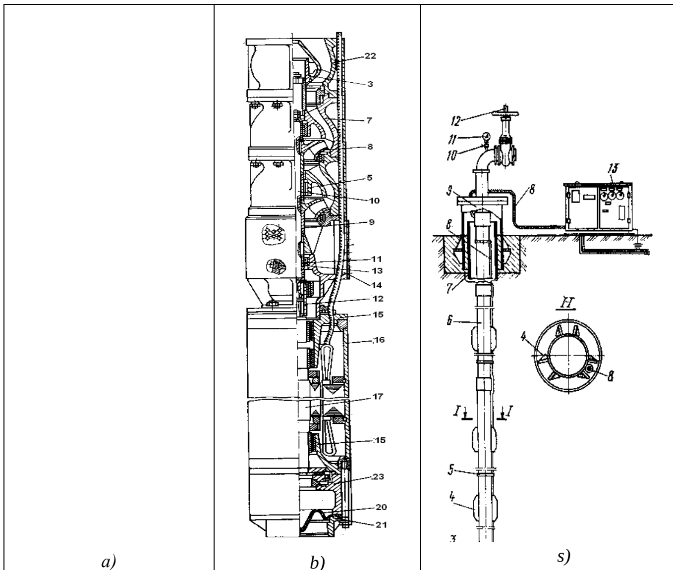
Rasm 1.16. ЭЦВ турдagi nasoslarning konstruksiyasi va o'rnatish sxemasi.
