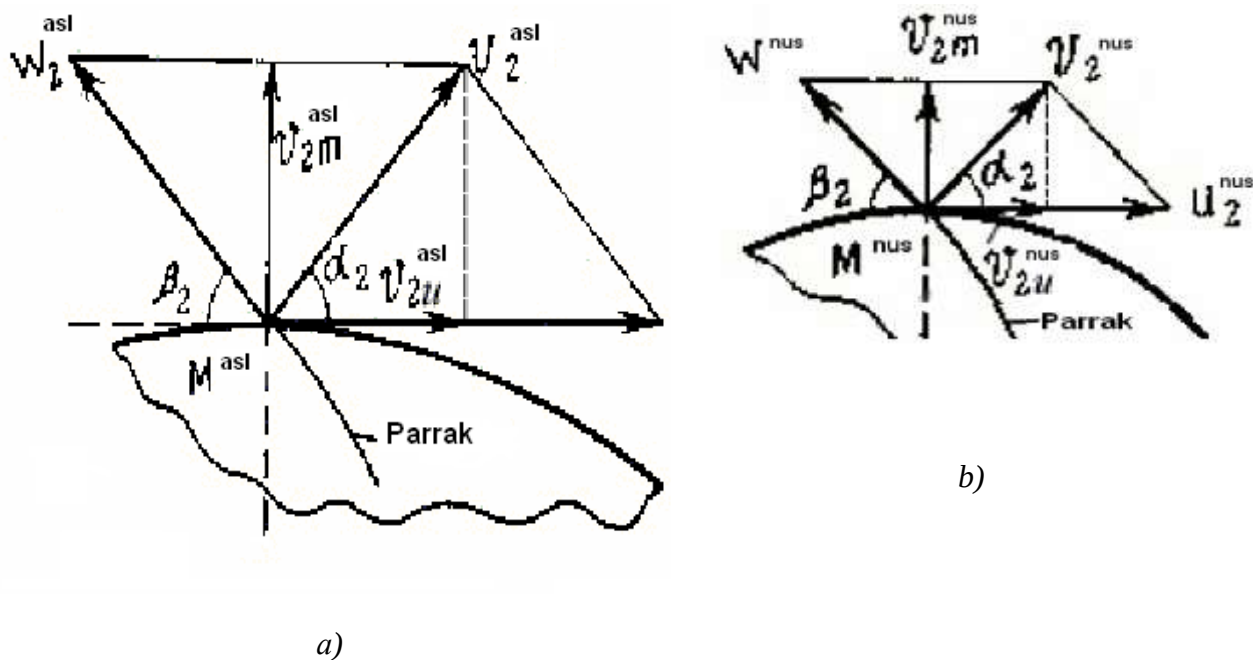
Rasm 1.38. Kinematik o'xshash asl (a) va nusxa (b) ish g'ildiraklaridan chiqishdagi tezlik uchburchaklari.
