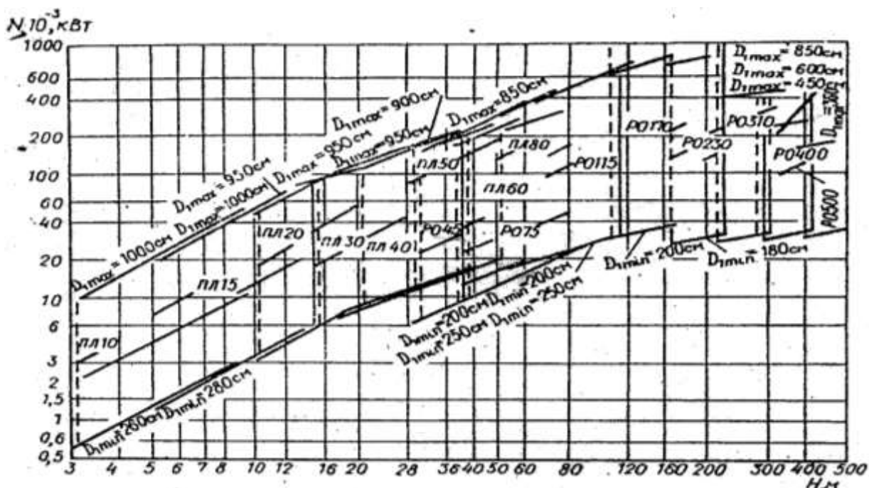
Rasm 2.2. Hidroturbina nomenklaturasi.
