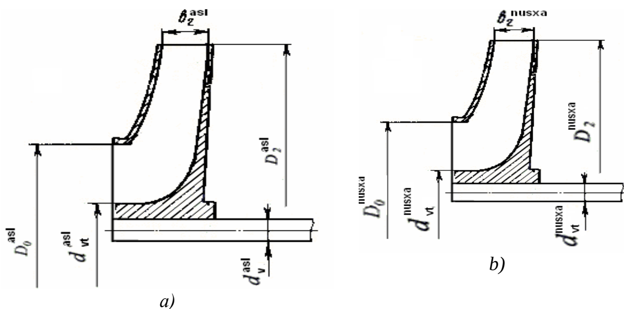
Rasm 1.37. Geometrik o'xshash asl (a) va nusxa (b) nasoslarning ish g'ildiraklari.
