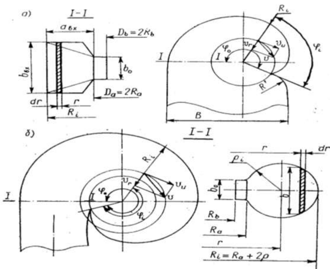
11-rasm. Spiral kameralarni gidromexanik hisoblashda V_r radial tezlikni bir hilligini ta'minlash sharti
