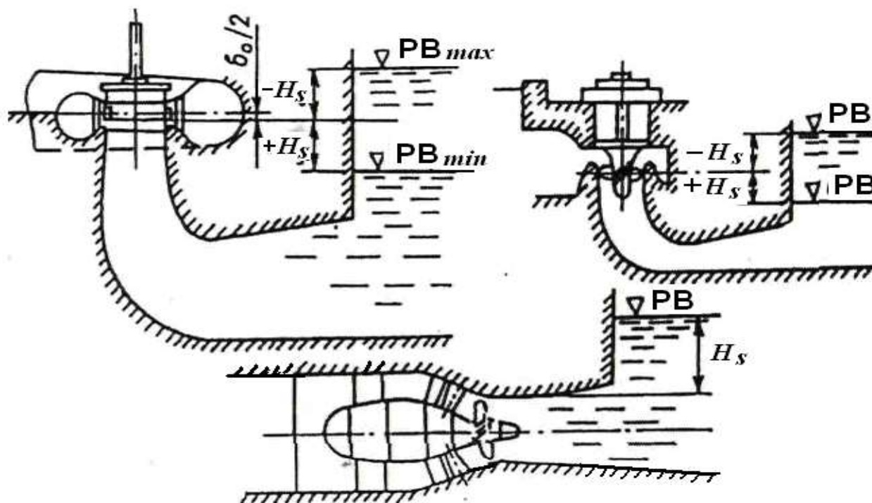
Rasm 2.5. Gidroturbina turiga qarab so'rish balandligi h_s ni berilishi.
