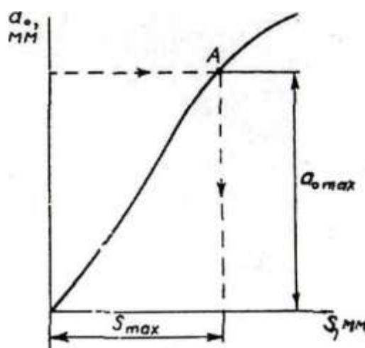
Rasm 2.22 a_{0max} ochilish darajasiini ta'minlashda servomotor porshenini maksimal yurish yo'li S_{MAX} ni aniqlash grafigi.
