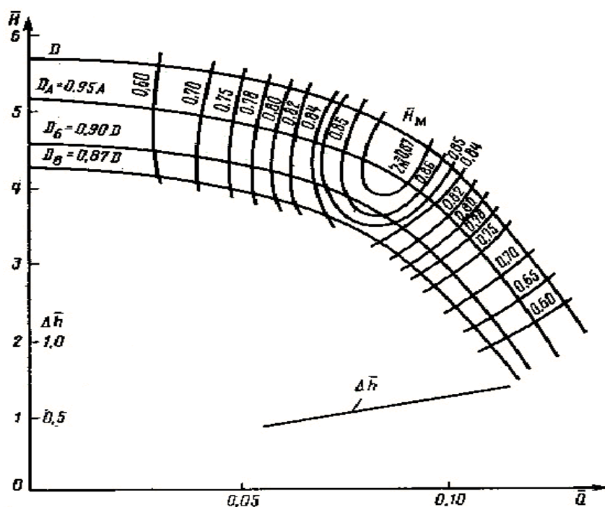
Rasm 1.43. Markazdan qochma nasosning o'lchov birliklarisiz xarakteristikalarini.
