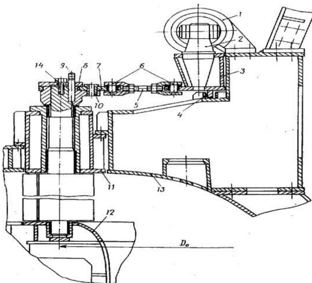
18-rasm. Yo'naltiruvchi apparat kurakcharini boshqa elementlar bilan birikish sxemasi
