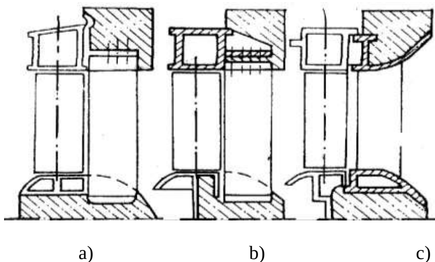
Rasm 2.15. Statorni beton bilan bog'liq, bo'lgan kolonnalarini ko'rinishi
