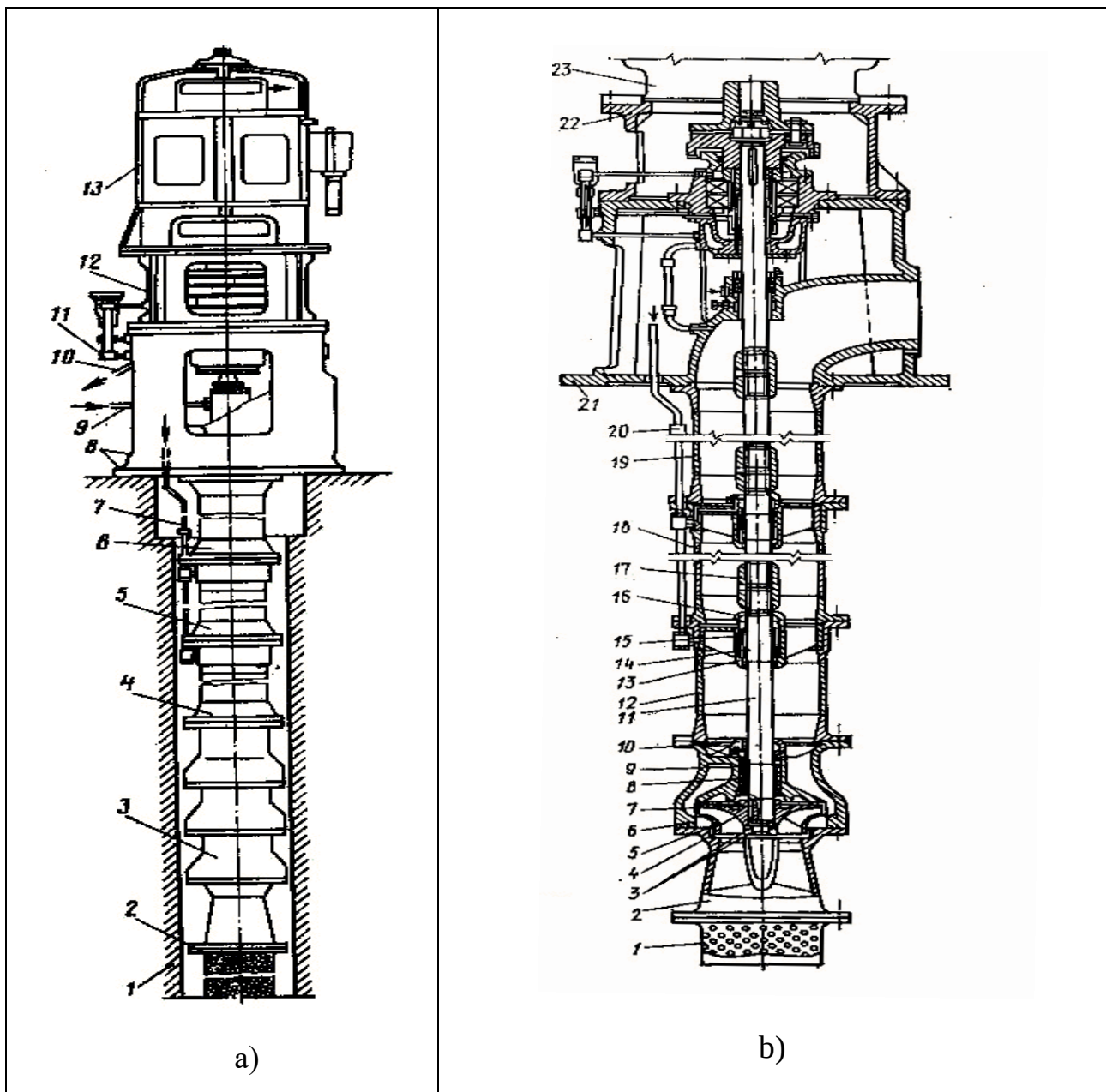
Rasm 1.15. A turdagi transmissiyali nasos qurilmalari konstruksiyasi.
