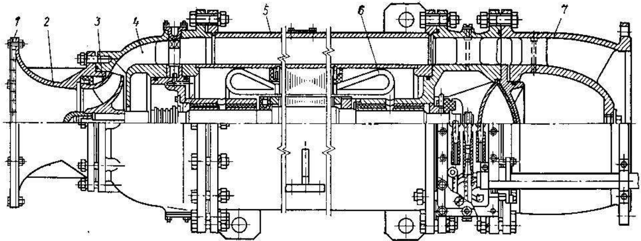
Rasm 1.12. Suyuqlikka cho'ktirilib ishlatiladigan markazdan qochma monoblokli nasosning konstruksiyasi
