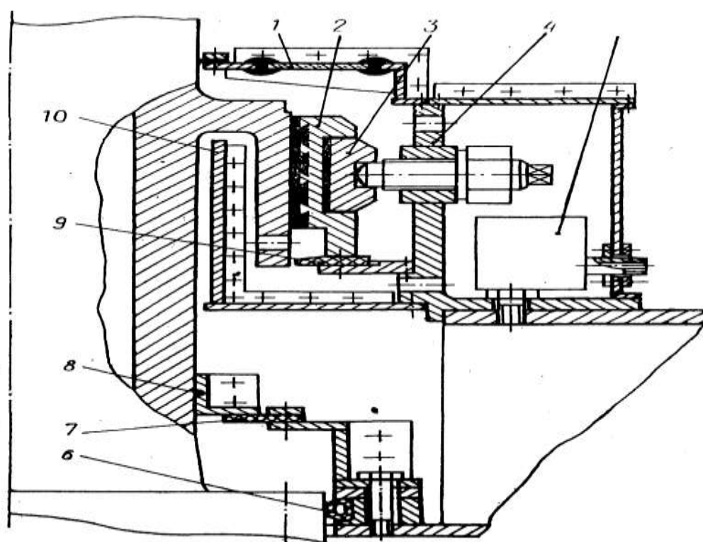
Rasm 2.40. Moy bilan ishlaydigan podshipnik konstruksiyasi
