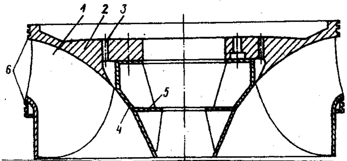
Rasm 2.32. H=175-230\text{ m} naporlar oralig'ida ishlovchi radial-o'qli gidroturbina konstruksiyasi
