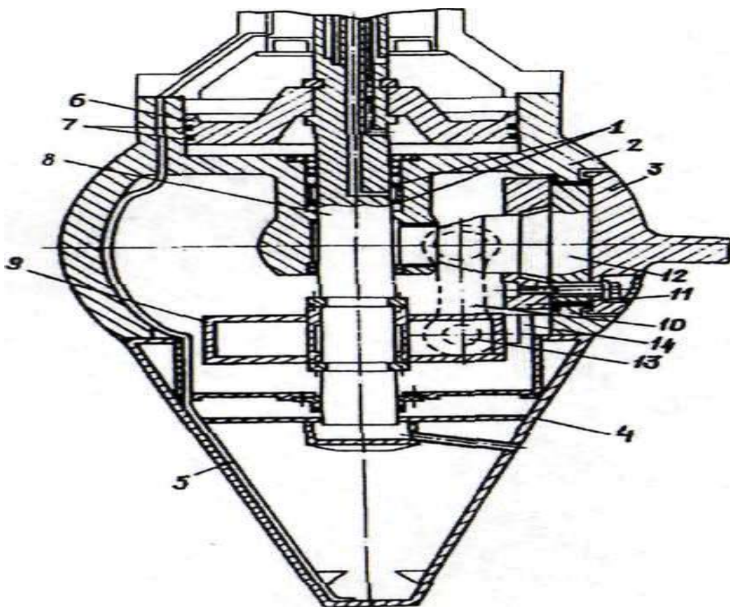
Rasm 2.34. Burama kurakli gidroturbina ishchi g'ildiragini konstruksiyasi.
