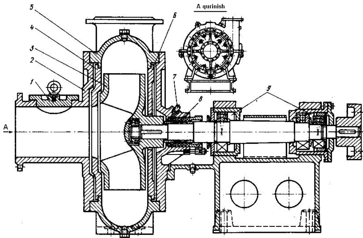
Rasm 1.11. Zirxli diskli, tuprok suruvchi nasosning konstruksiyasi.
