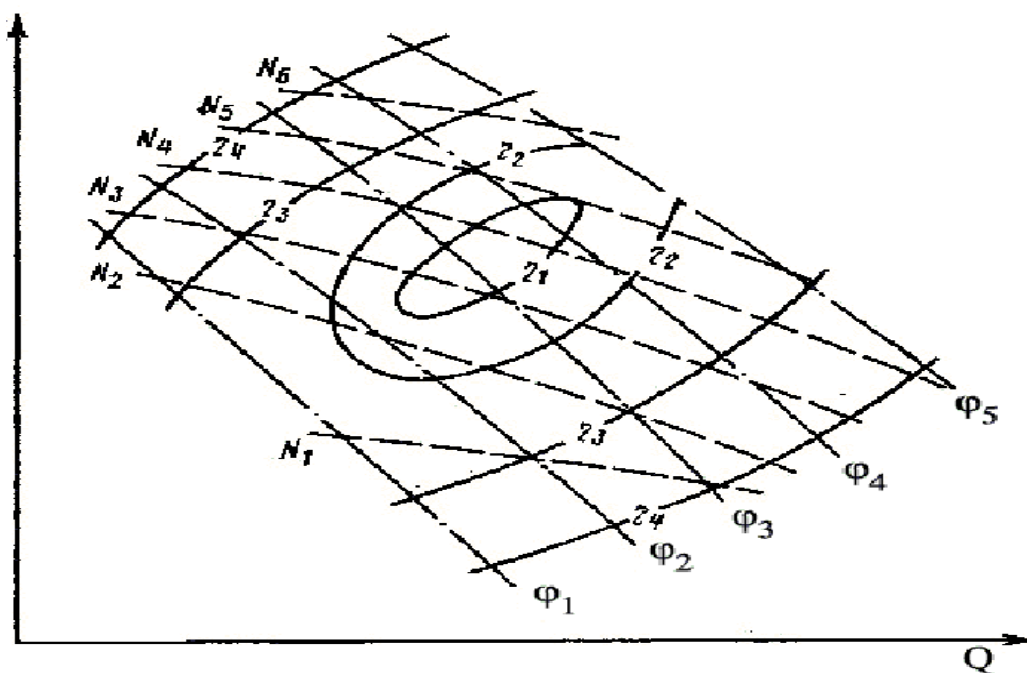
Rasm 1.46 O'qiy nasoslarning universal xarakteristiklari
