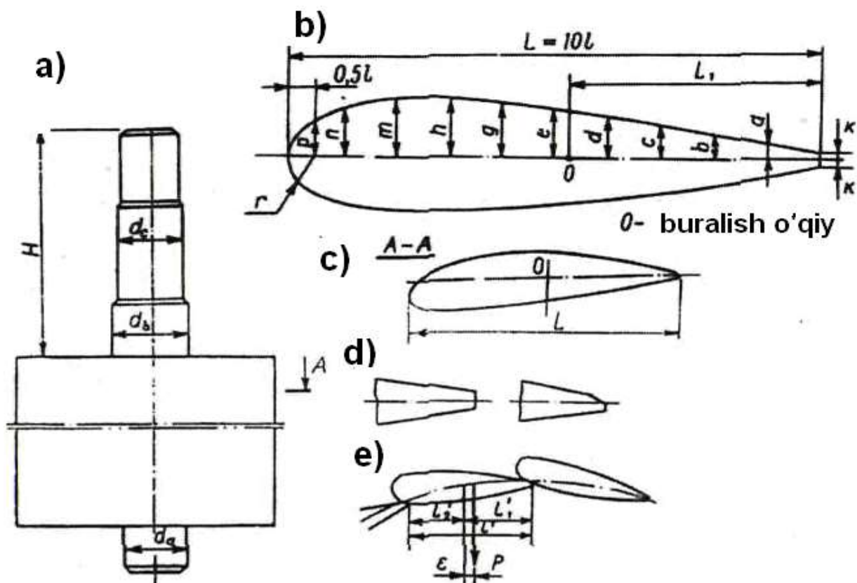
Rasm 2.20 Yo'naltiruvchi apparat kurakchalari konstruksiyasi va profil ko'rinishi
