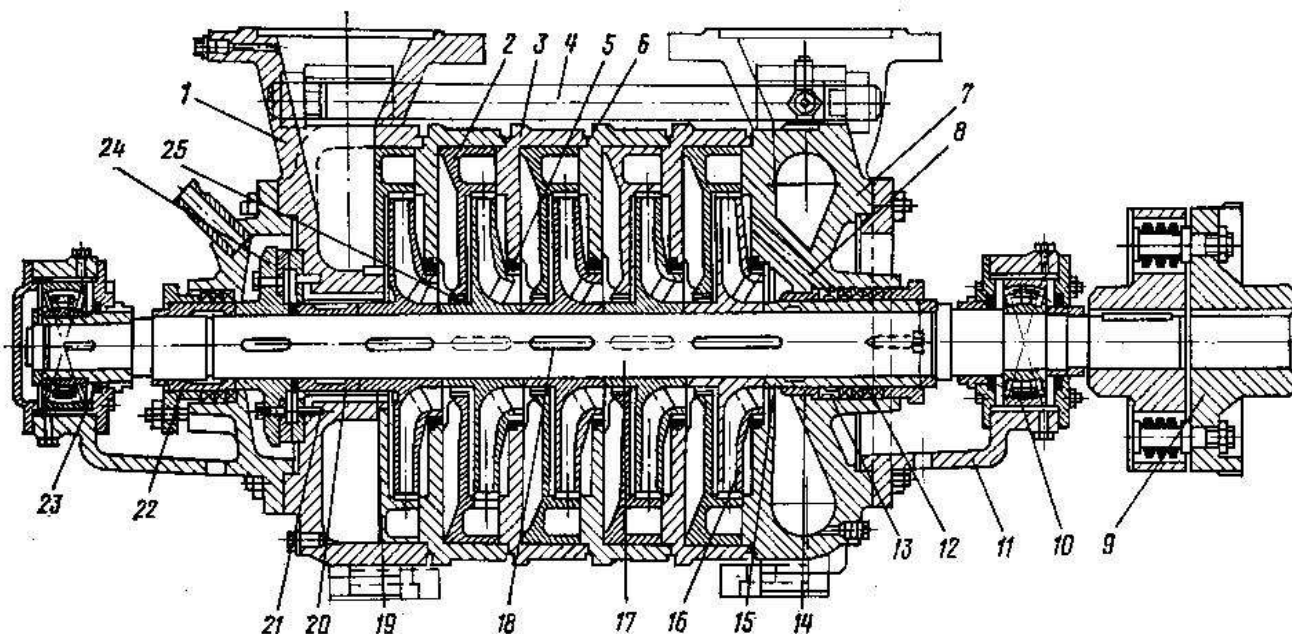
Rasm 1.8. Koʻp bosqichli markazdan qochma seksiyali nasosning konstruksiyasi.
