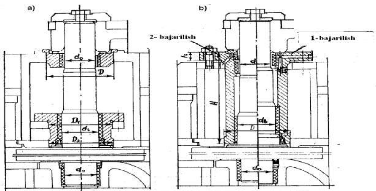
Rasm 2.23 Kurakcha o'qining turbina qopqog'i va pastki xalqa bilan birikishi.
