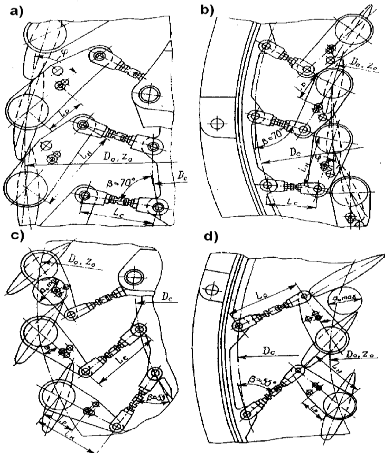
Rasm 2.19. Burovchi xalqa bilan yo'naltiruvchi apparat mexanizmini birikish sxemasi va parametrlari
