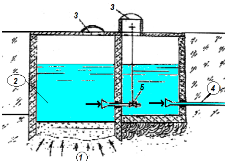
40- расм. Кўтарилиб чиқаётган булоқлар каптажи:
