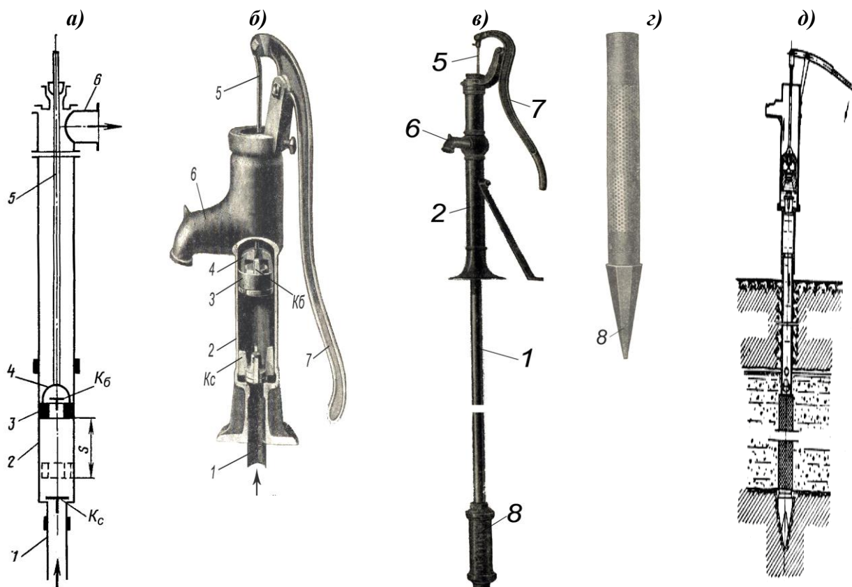
38-расм. Штангали поршенли насос:
