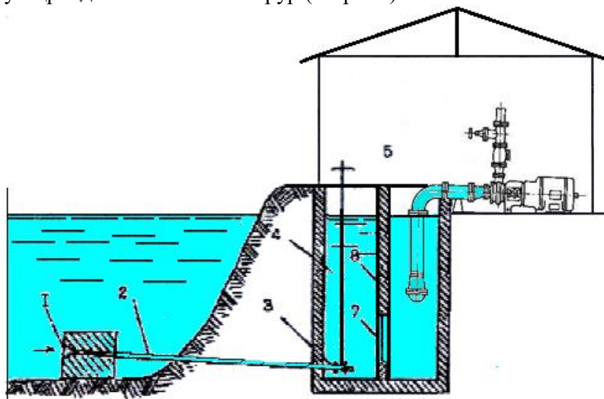
36-расм. Қирғоқдан узоқроқда жойлашган сув олиш иншооти:
