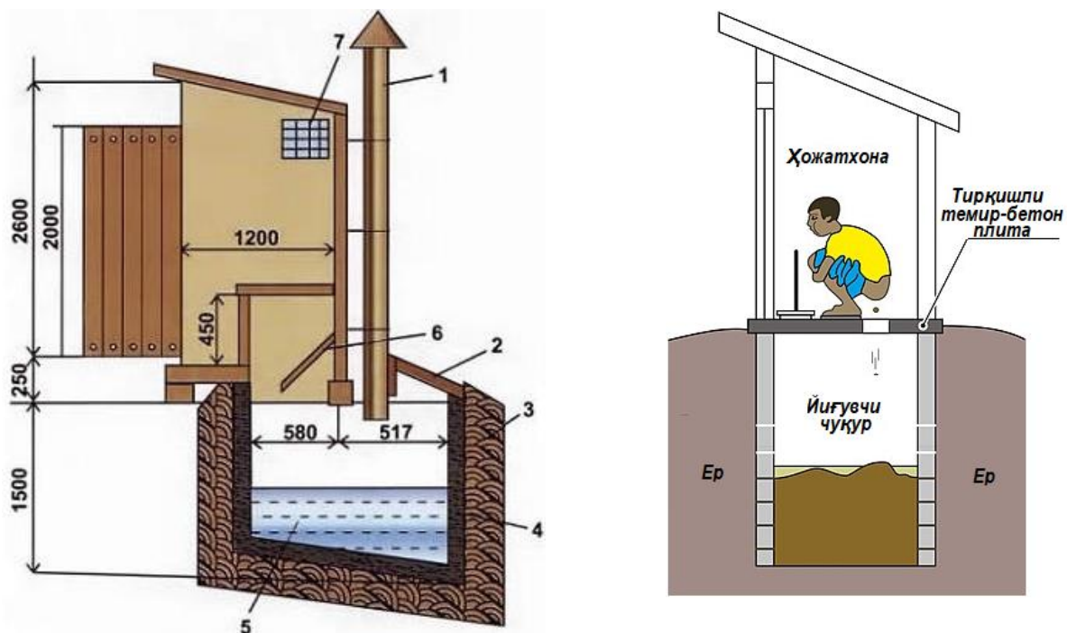
45-расм. Оддий ҳожатхоналарнинг конструкциялари:
