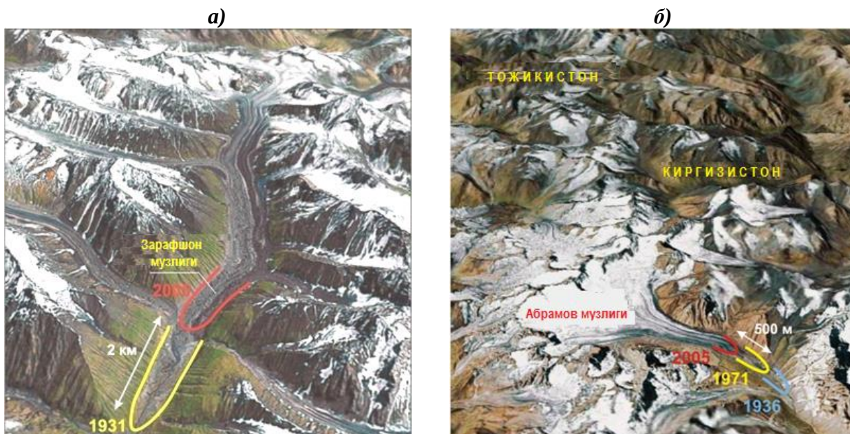
11-расм. Иқлим ўзгариши натижасида Зарафшон ва Абрамова (Қирғизистон) музлиги ўлчамлари ва ҳажмининг қисқариб бориши
