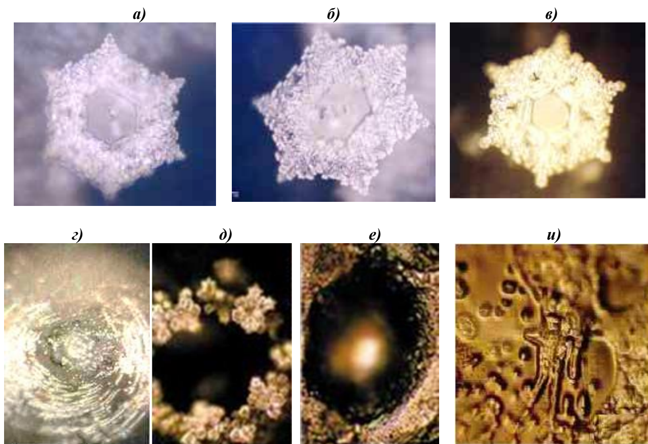
46-расм. Ҳар хил сўзлар айтилганда ҳосил бўлган кристаллар:
