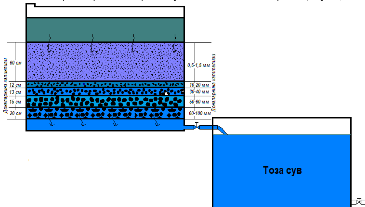
42-расм. Оддий сув тозалаш иншооти:
