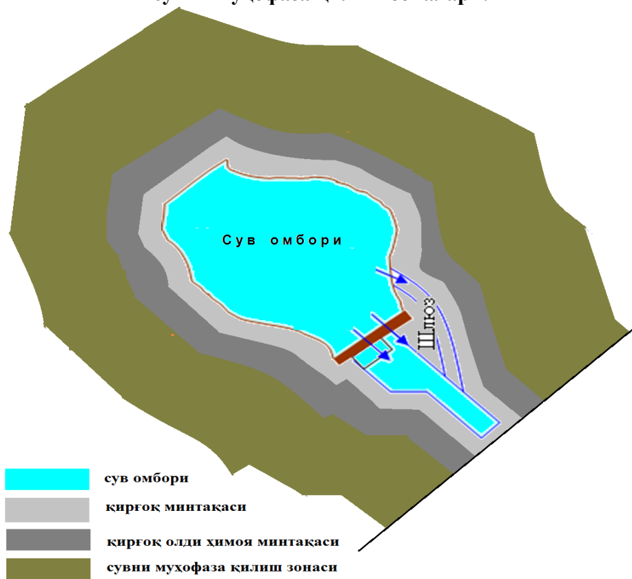
54-расм. Сүв омборларининг сүвни муҳофаза қилиш зоналари.
