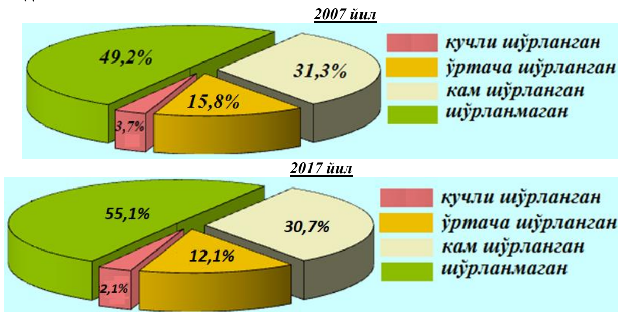
20-расм. Ерларнинг мелиоратив ҳолатини ўзгариш динамикаси
