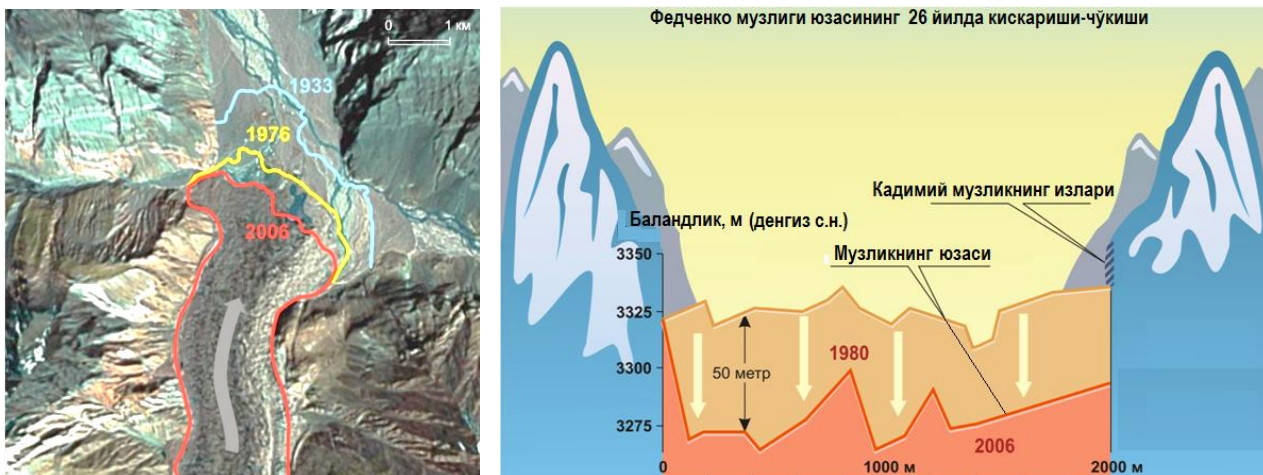
9-расм. Иқлим ўзгариши натижасида Федченко музлиги (Тожикистон) ўлчамлари ва ҳажмининг қисқариб бориши.
