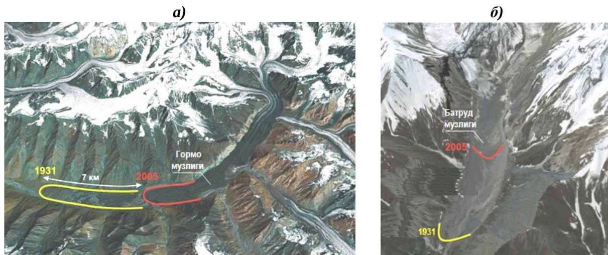
10-расм. Иқлим ўзгариши натижасида Горма ва Батруд музлиги (Тожикистон) ўлчамлари ва ҳажмининг қисқариб бориши.
