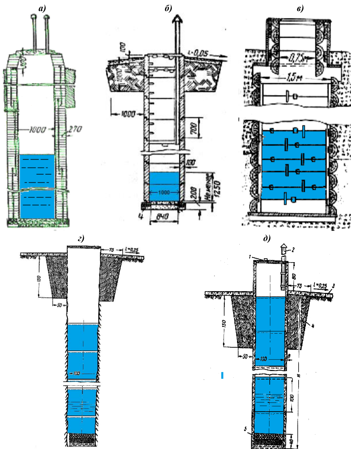
39-расм. Деворлари ҳар хил материаллар билан қопланган шахтали қудуқлар: а-ғиштли; б-ийгма темир-бетон; в-ёғоч; з-қопламасиз ; д-харсангтошли.
